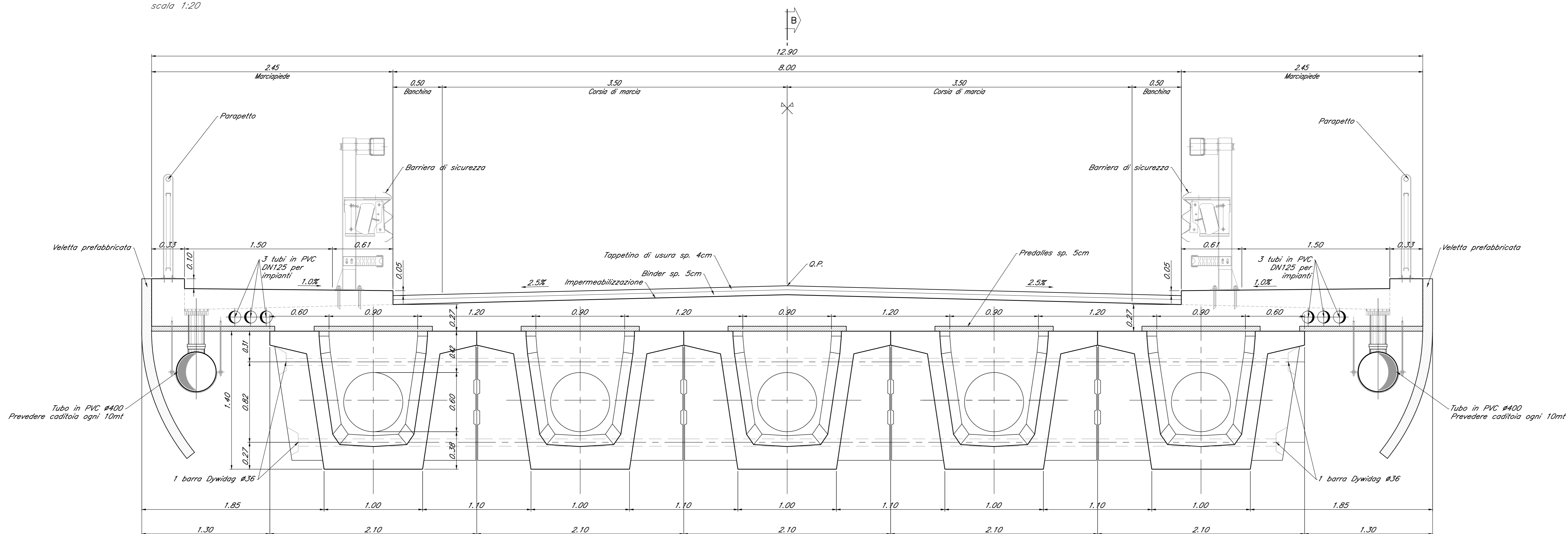
Sezione "A" scala 1:20
