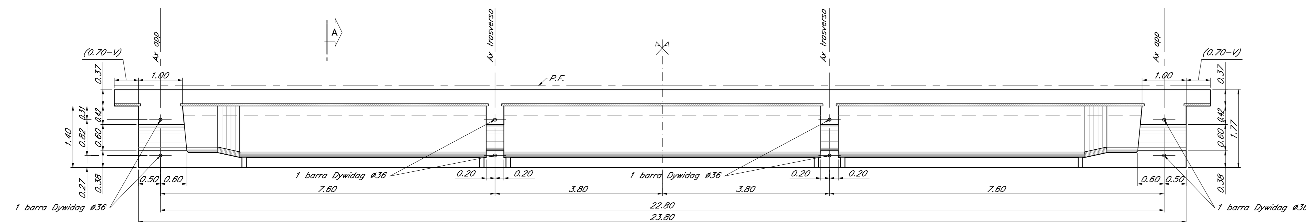
Sezione "A" scala 1:20
