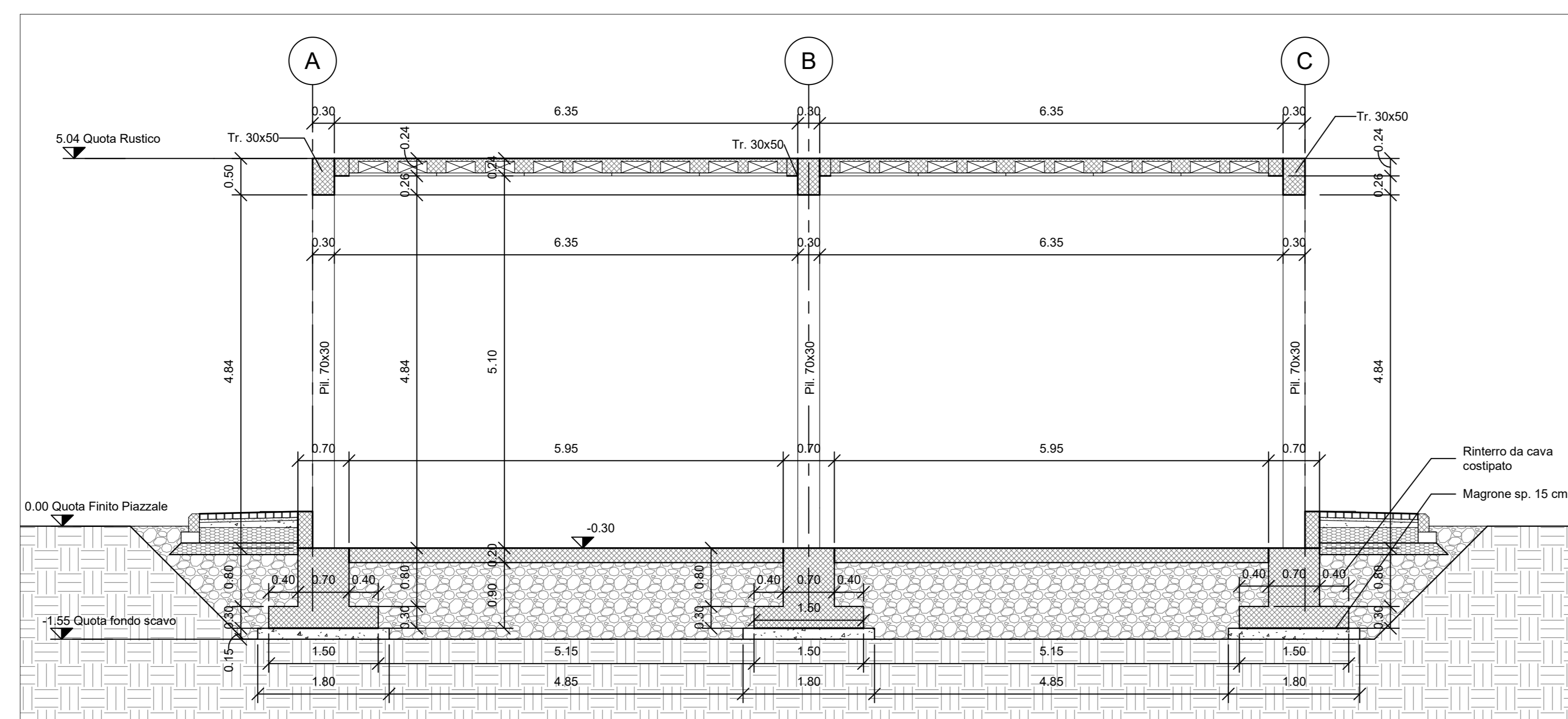
Sezione STR B-B' 1 : 50
