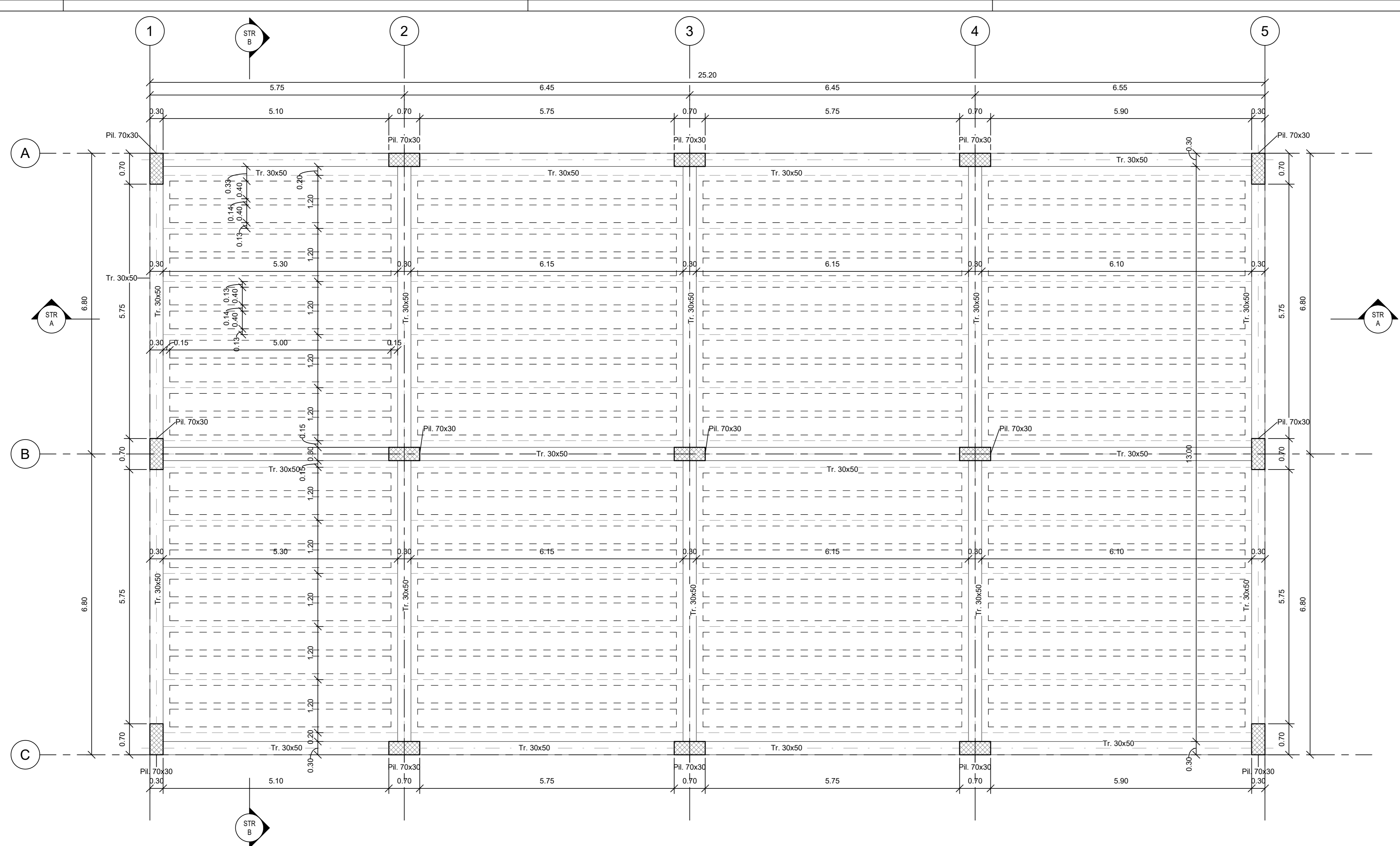
Carpenteria Copertura 1 : 50
