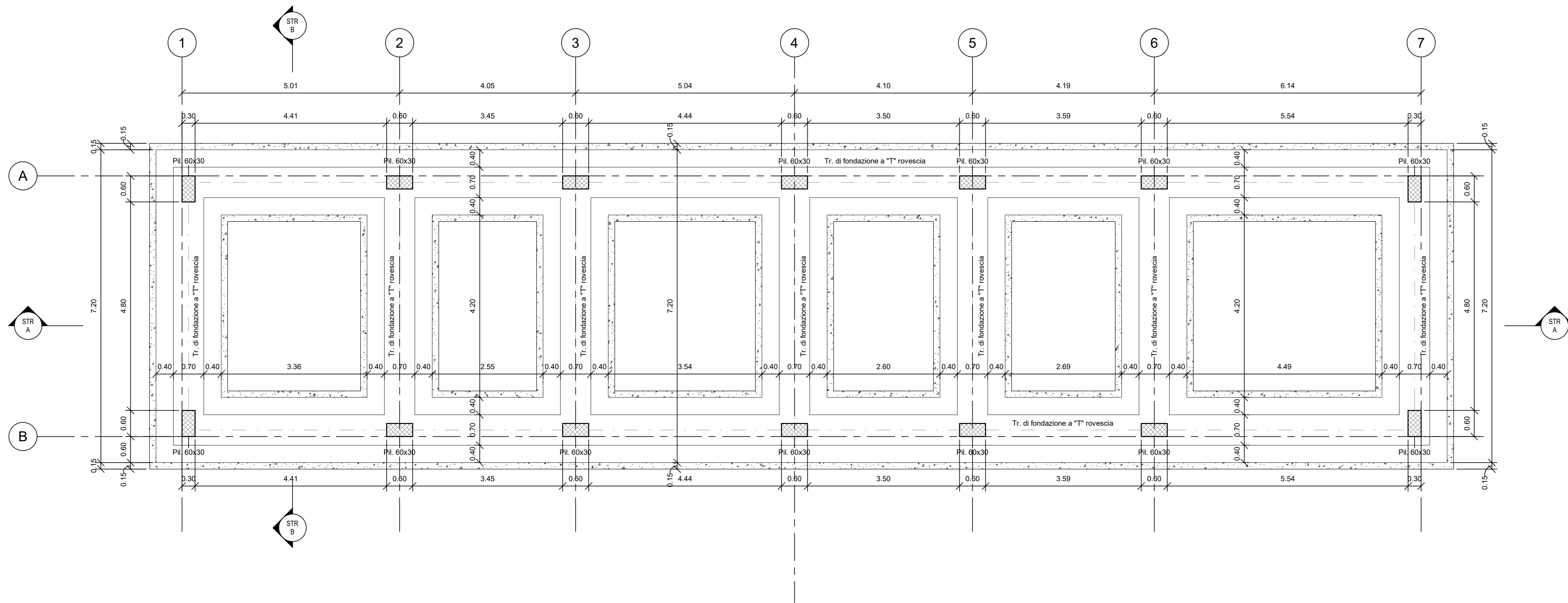
Carpenteria Fondazione - Planimetria 1 : 50
