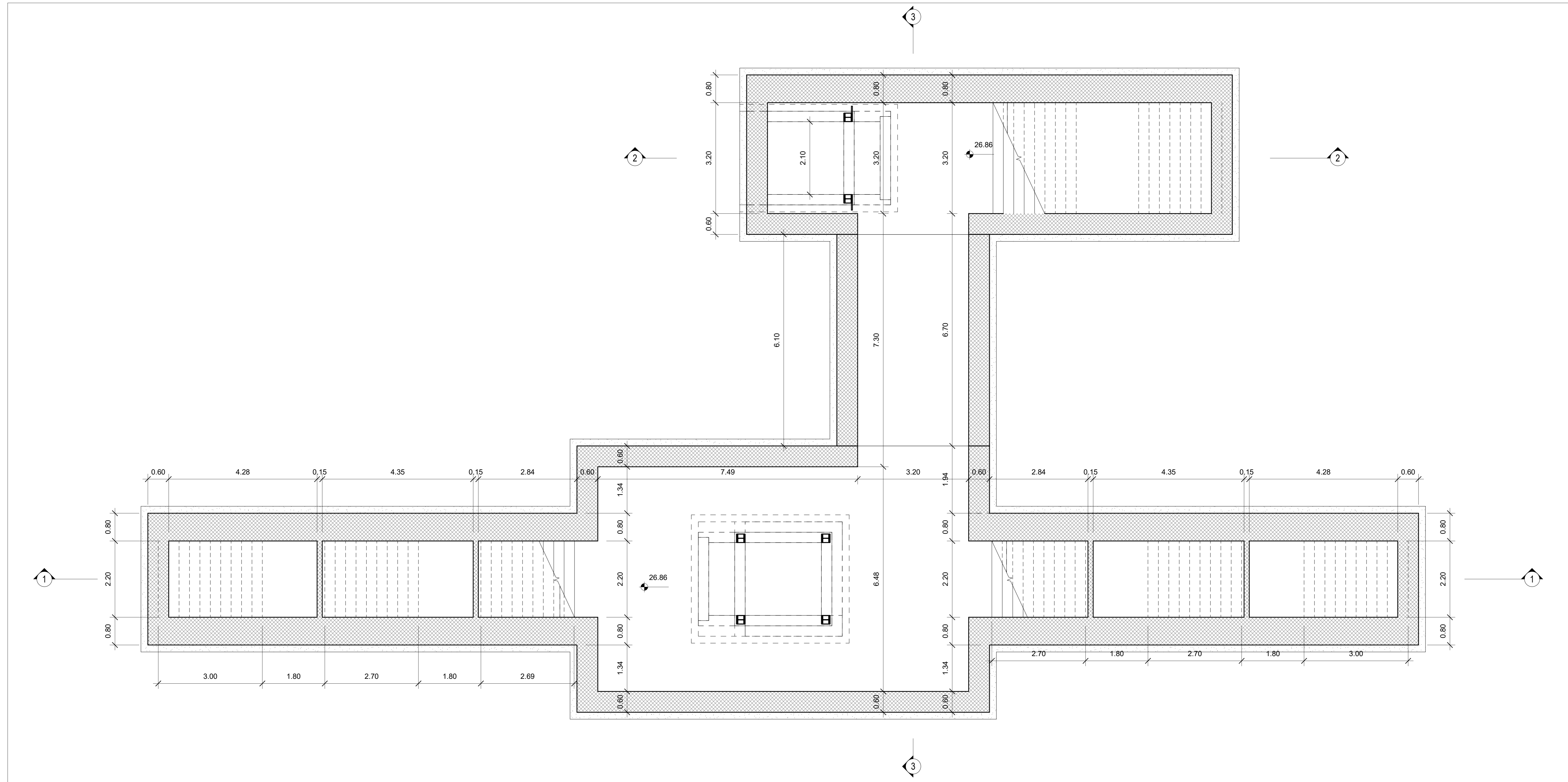
SAN-STR-Sottopasso 1 : 50
