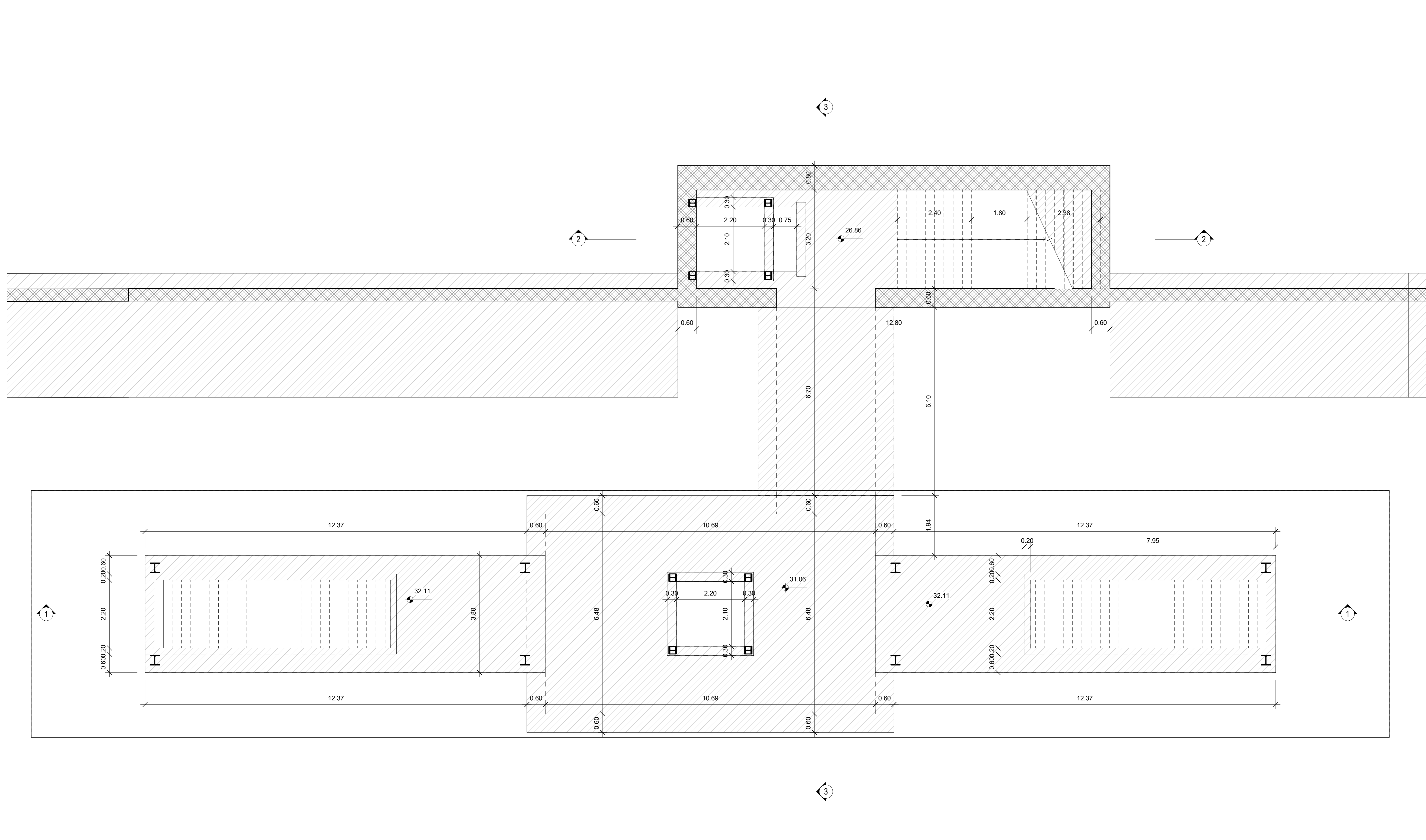
Pianta Spiccato Sottopasso 1:50
