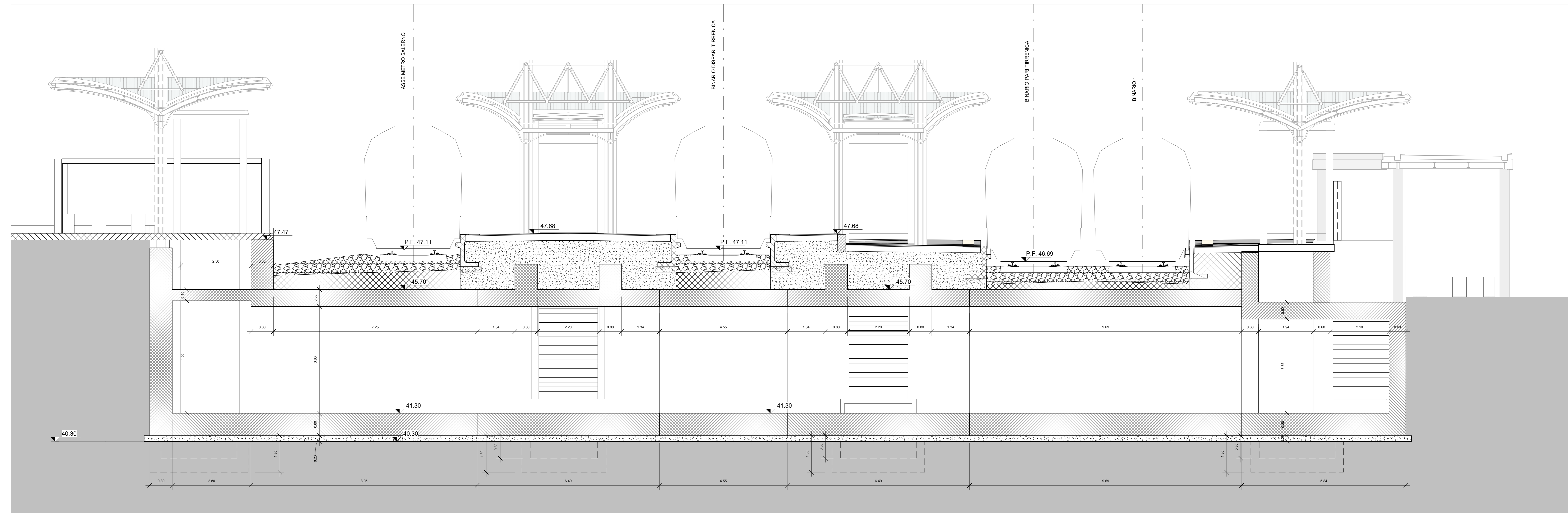
STR-SezA 1 : 50
