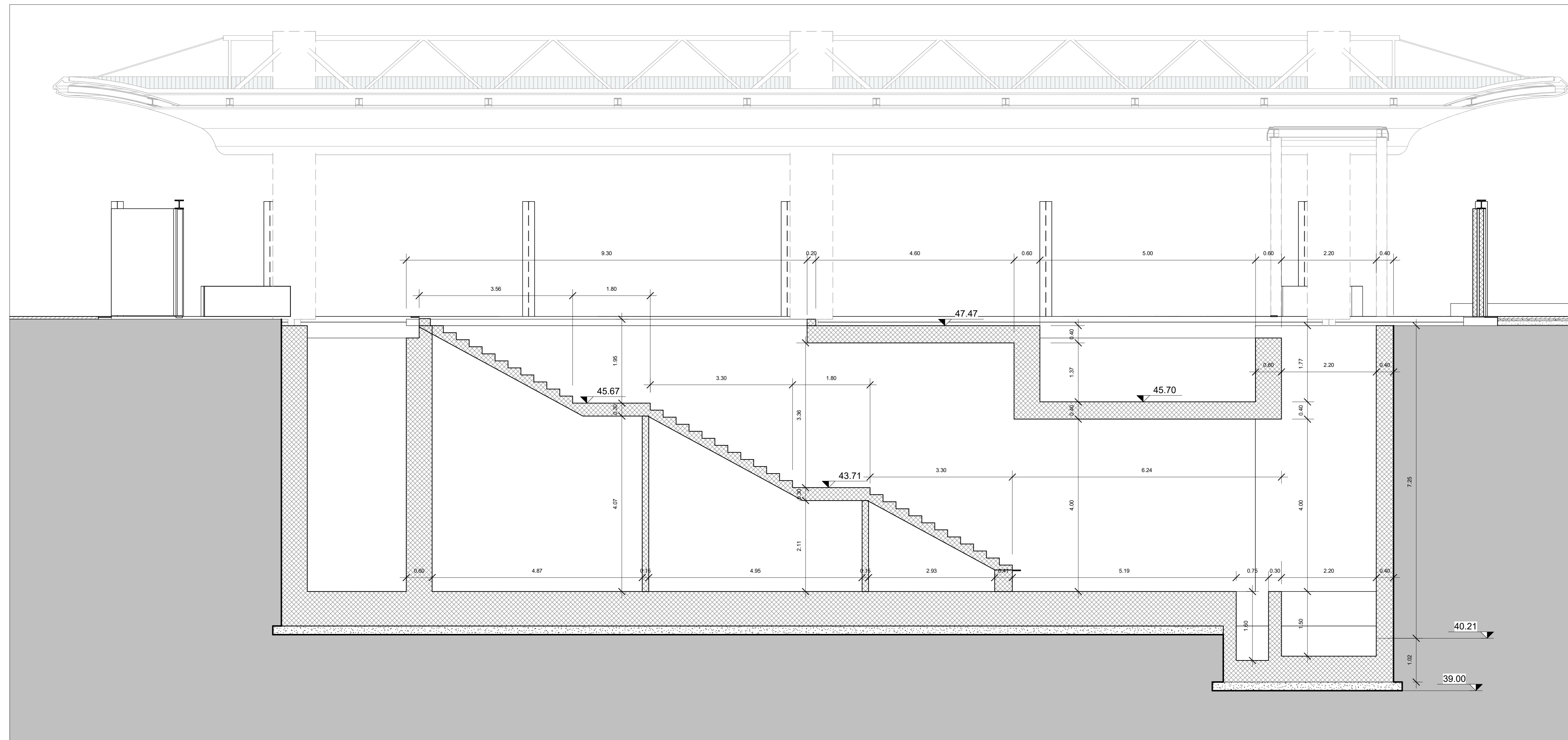
STR-SezB 1 : 50
