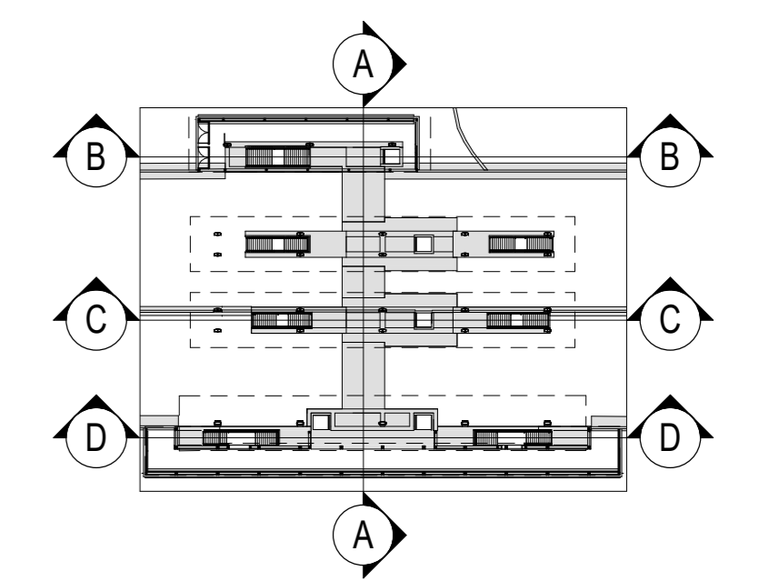
Keyplan 1 : 1000
