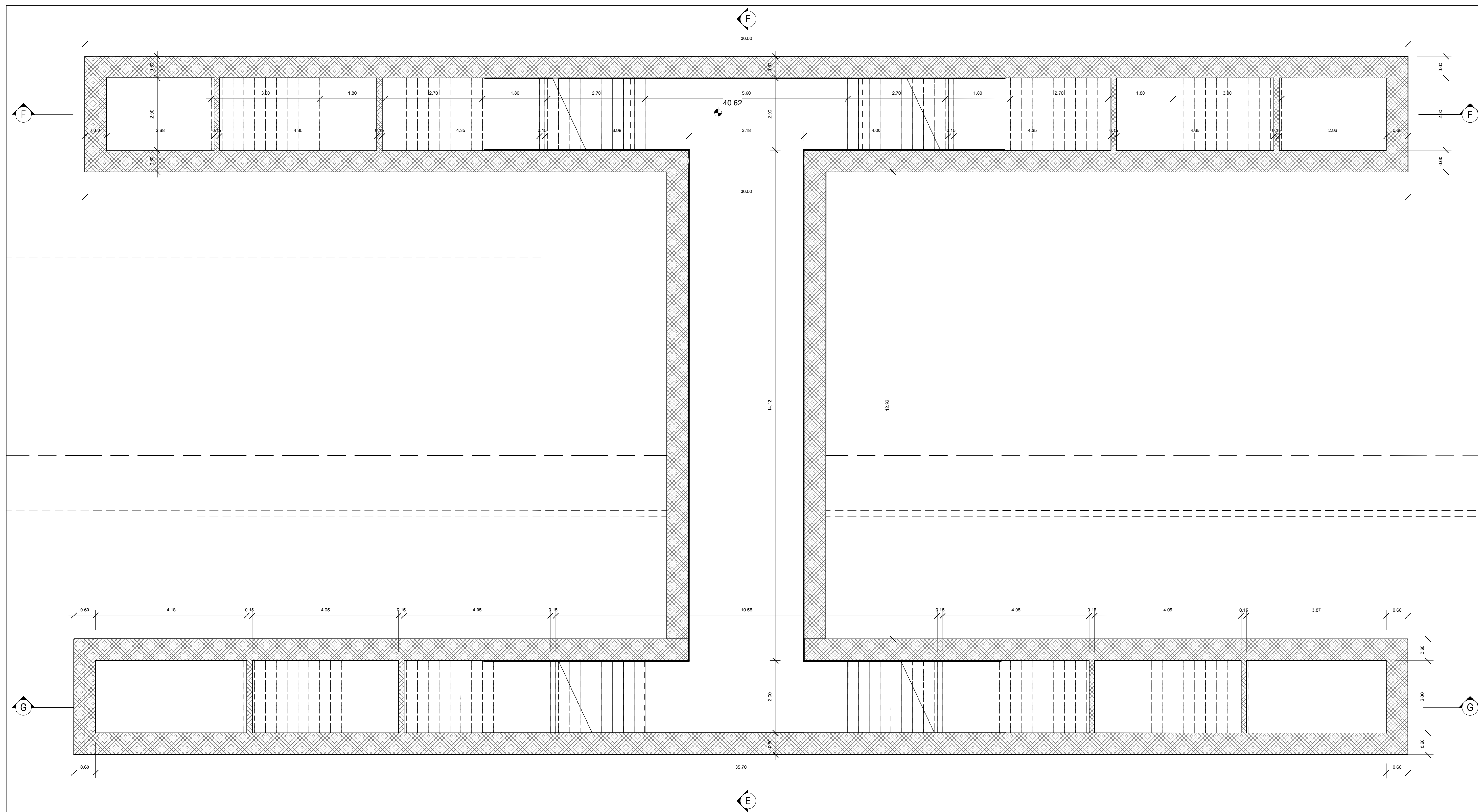
Pianta Sottopasso Emergenza 1:50
