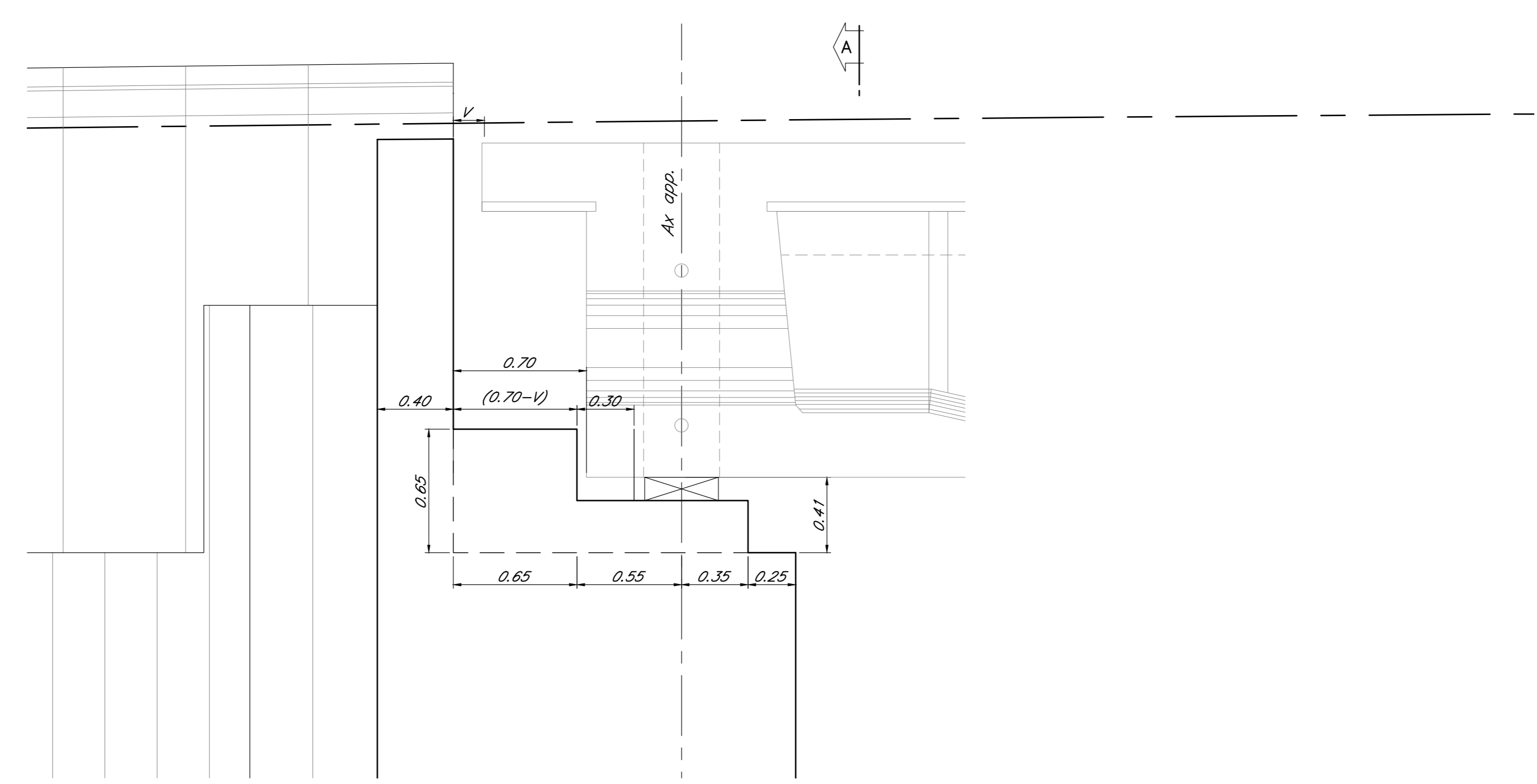
Sezione "B" Particolare baggioli scala 1:20
