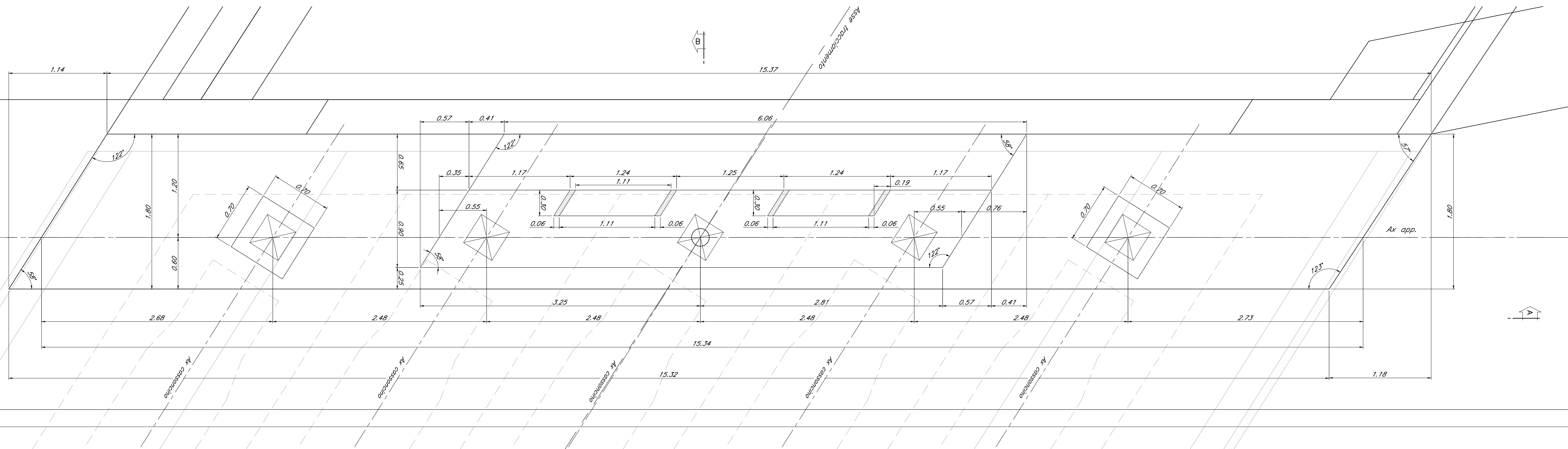
Vista dall'alto scala 1:20
