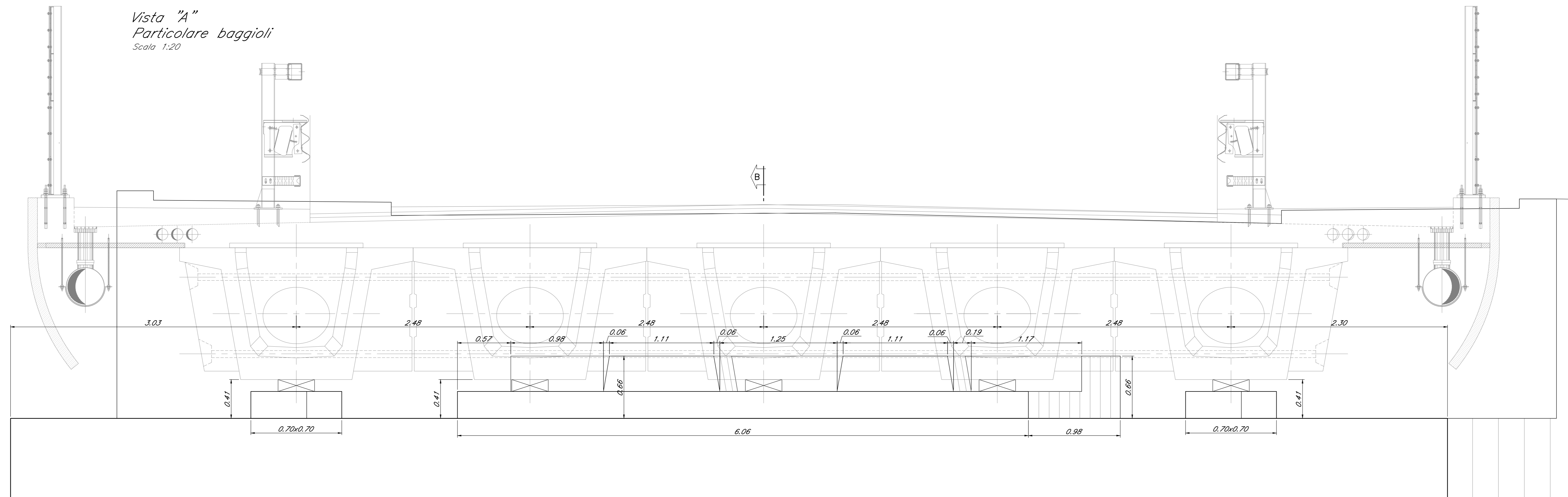
Sezione "B" Particolare baggioli Scala 1:20
