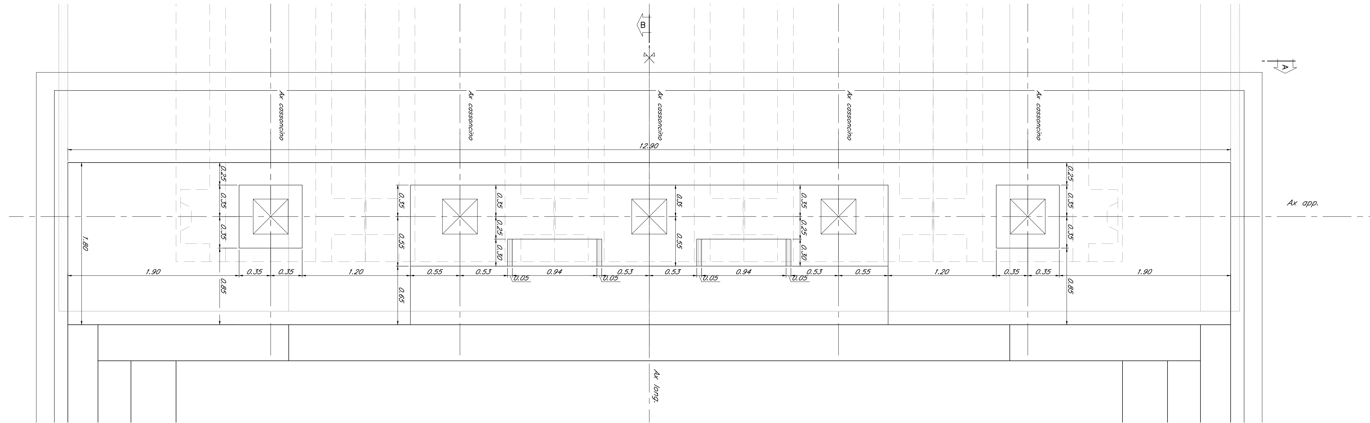
Vista dall'alto scala 1:20
