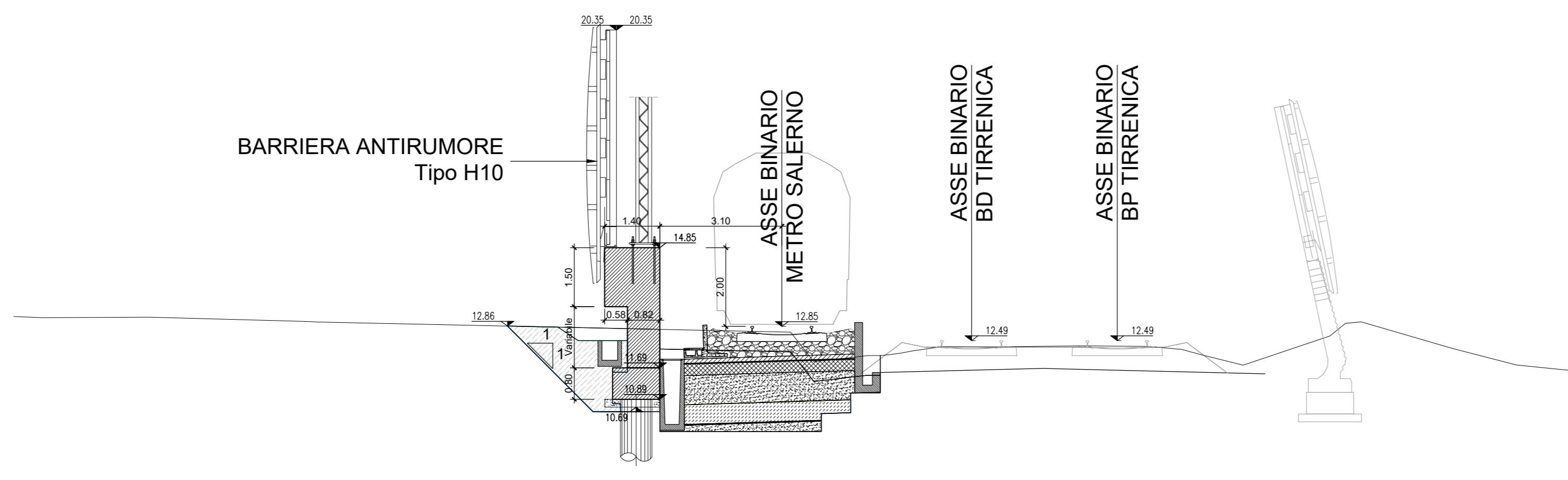
BARRIERE ANTIRUMORE SEZIONE TRASVERSALE 12 - Km 0+550.00 Scala 1:100
