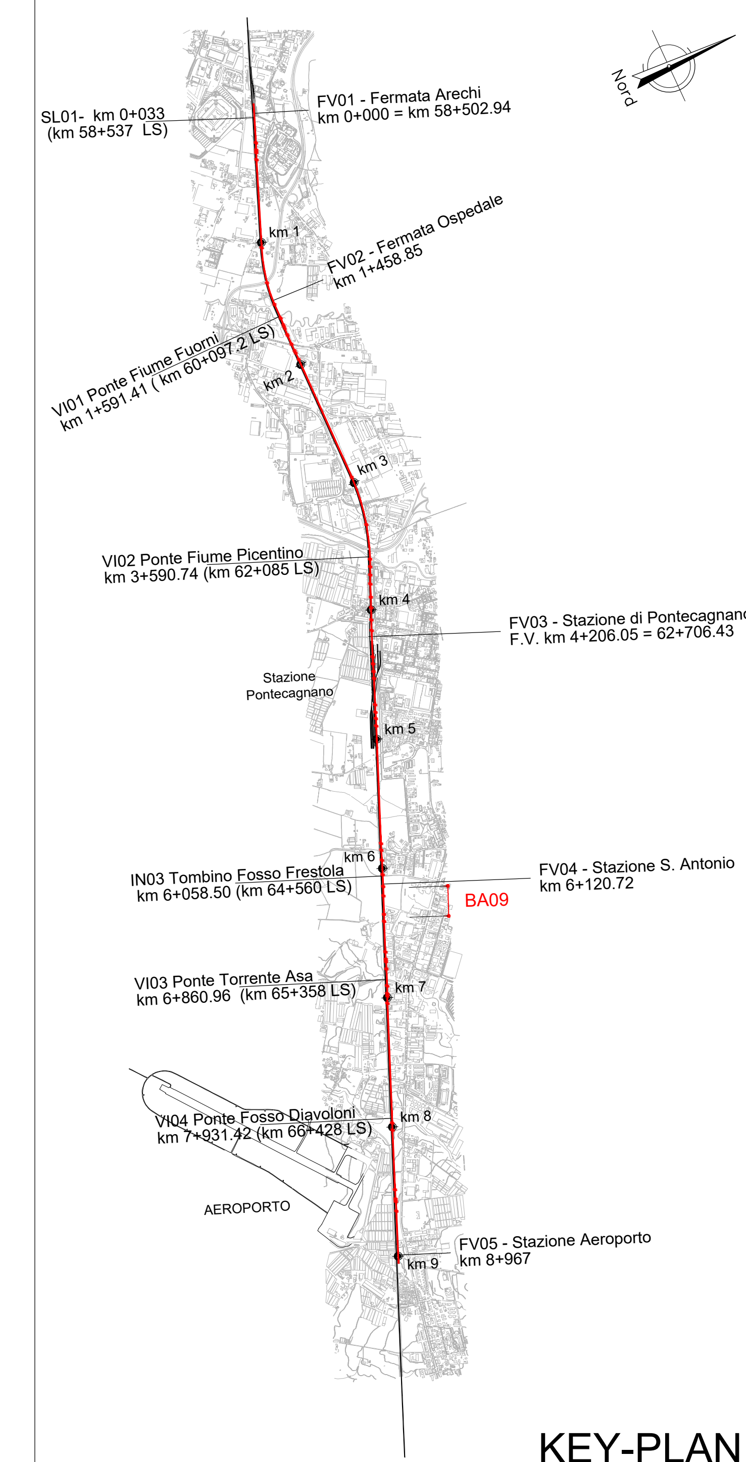
KEY-PLAN
