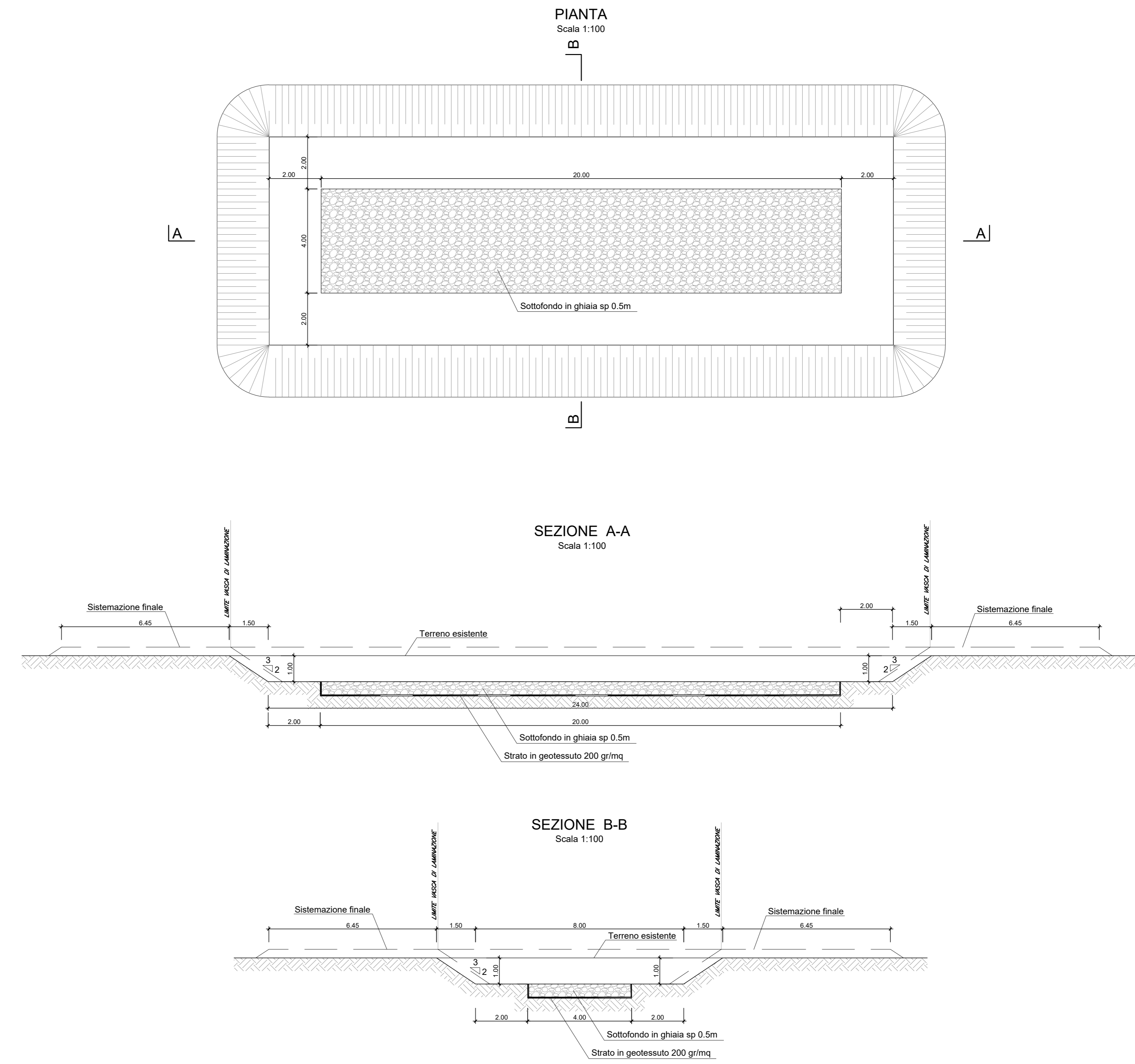
TIPOLOGICO VASCA DI DISPERSIONE
