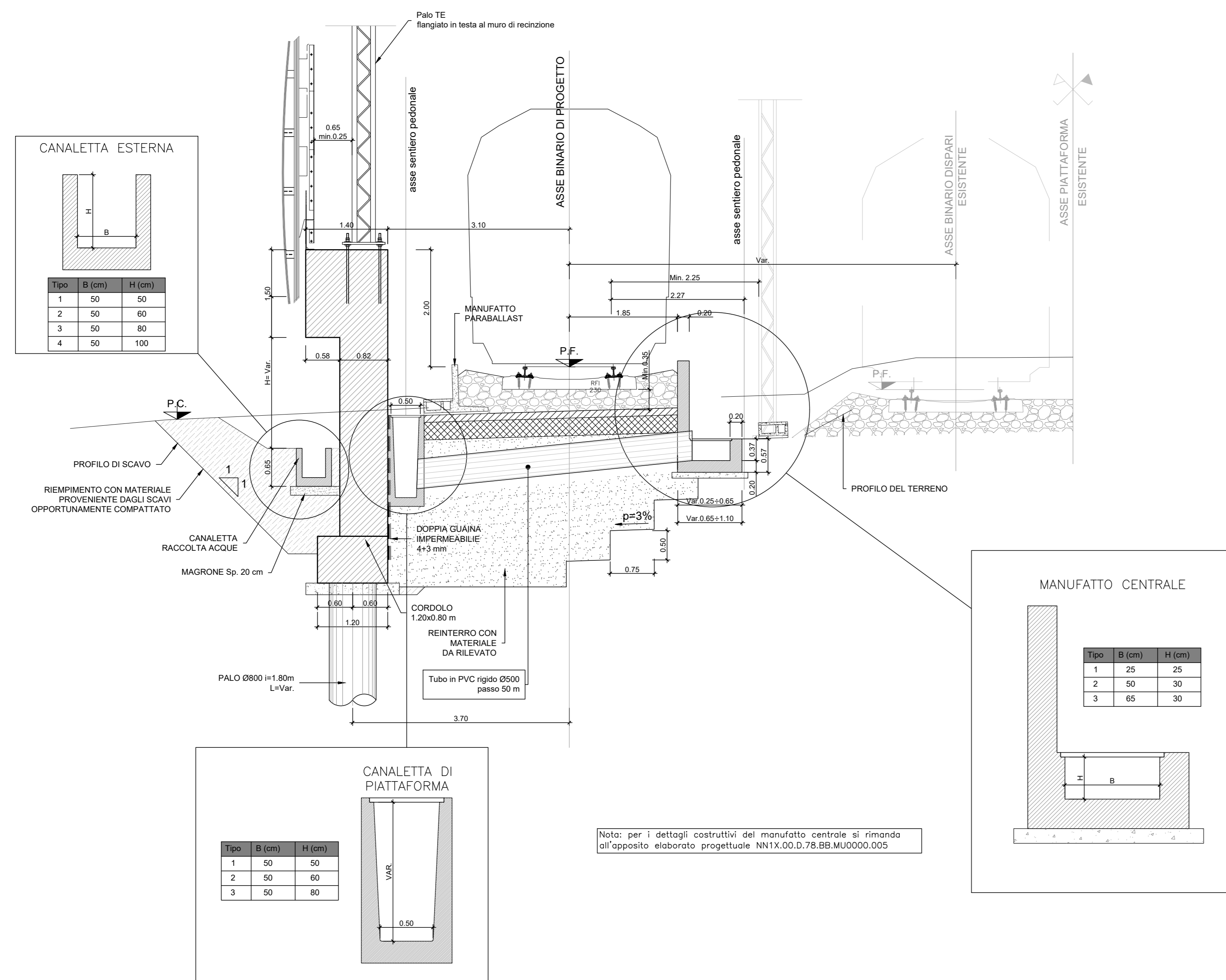
Sezione tipologica con scarico delle acque del manufatto centrale su canaletta di piattaforma
