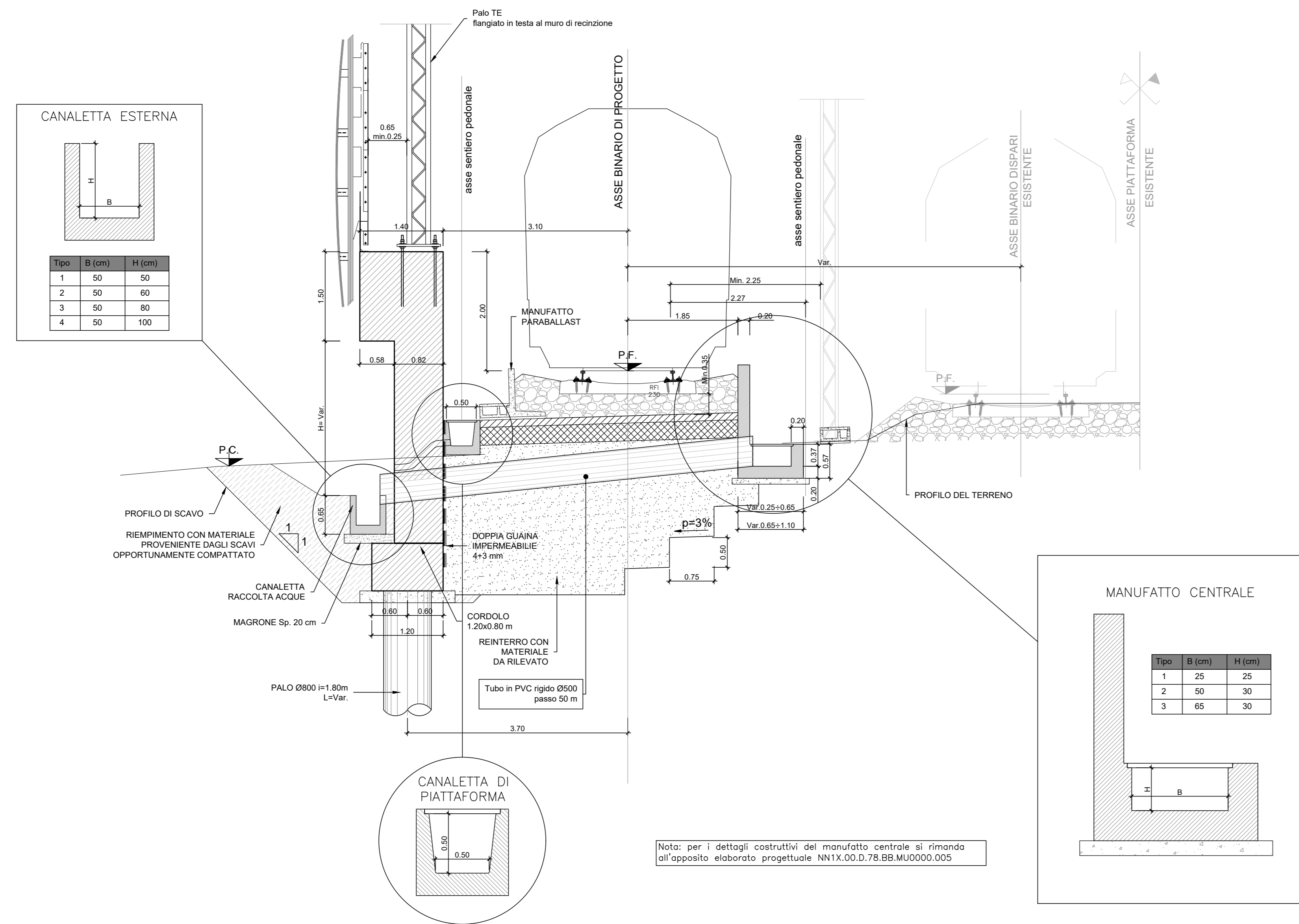
Sezione tipologica con scarico delle acque del manufatto centrale su canaletta esterna
