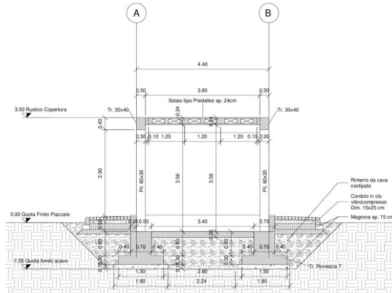
Sezione STR B-B'
