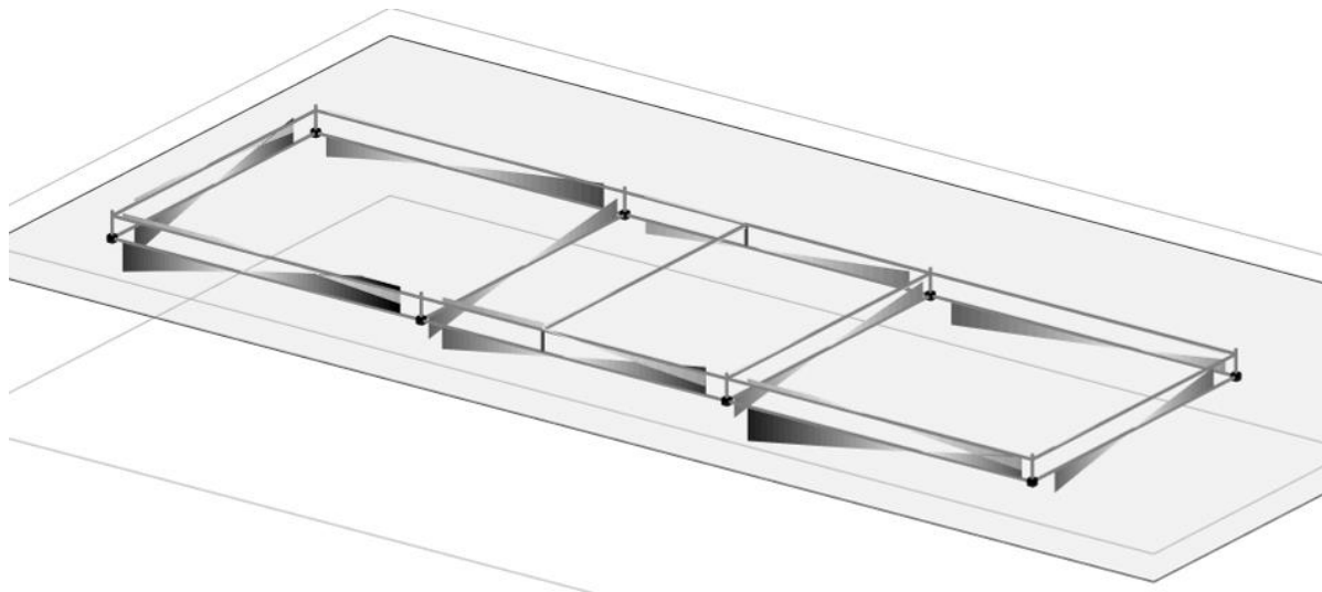
Figura 7-5 – Sollecitazioni di taglio SLU_CC37.
