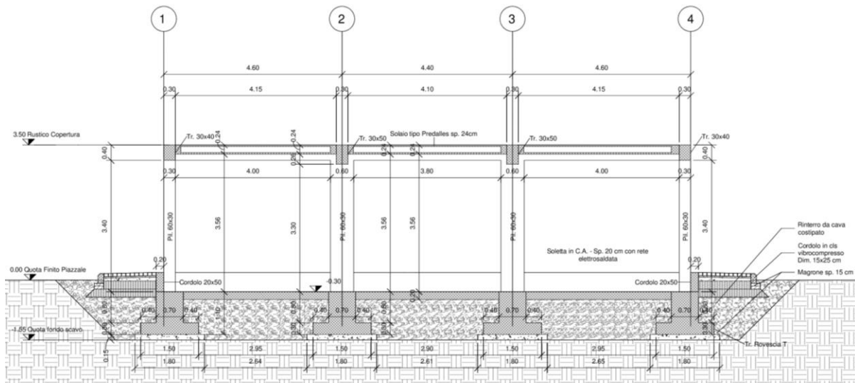
Figura 2-1 – Carpenteria Fondazione e Copertura.
