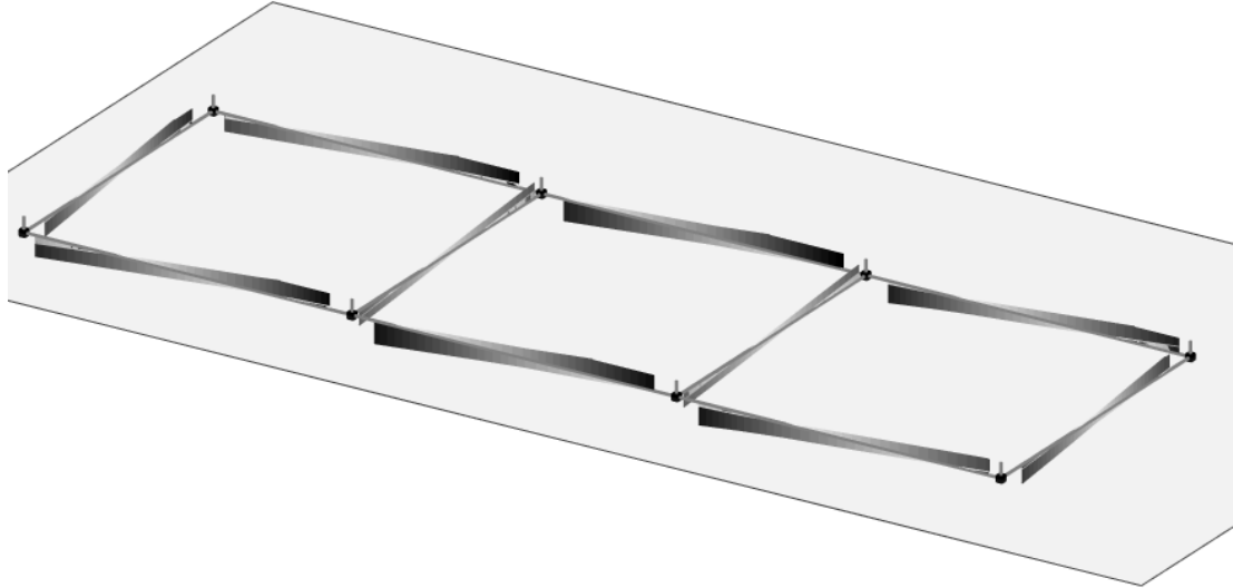
Figura 7-3 – Sollecitazioni di taglio SLV_CC1.
