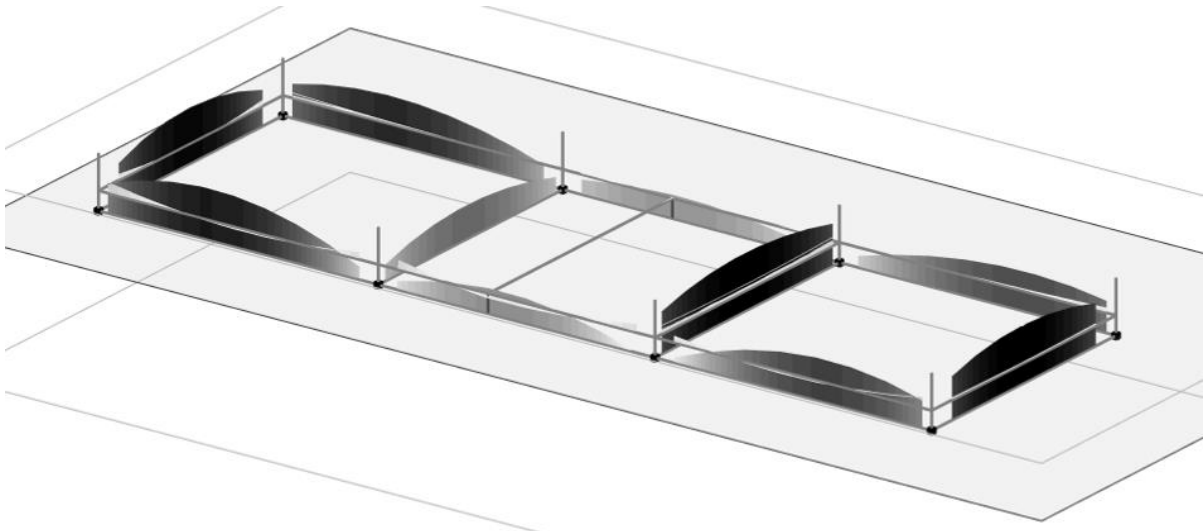
Figura 7-4 – Sollecitazioni flettenti SLU_CC37.
