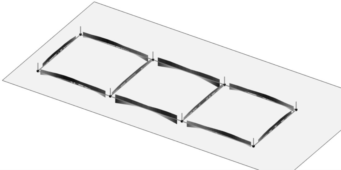
Figura 7-2 – Sollecitazioni flettenti SLV_CC1.
