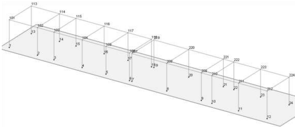
Figura 7.1-2 Numerazione nodi.
