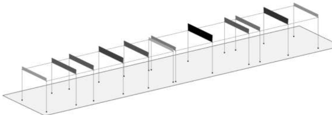
Figura 7.1-16 Schemi di carico - Permanenti solai
