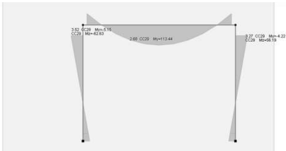
Figura 7.1-9 Diagramma dei momenti M3 – COMB_INV_SLU – Telaio interno.
