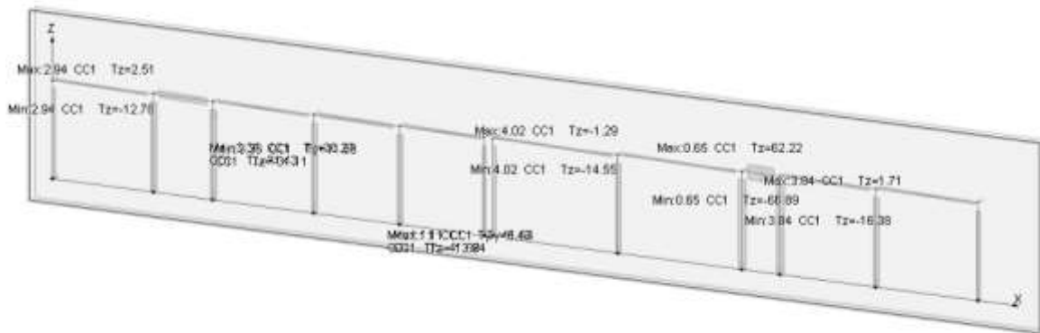
Figura 7.1-12 Diagramma del taglio V2 – COMB_INV_SLV_CC1 – Telaio di bordo
