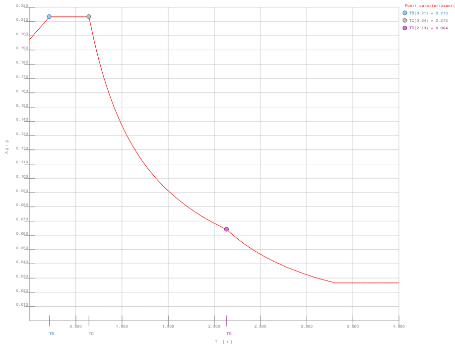
Spettro SLV
