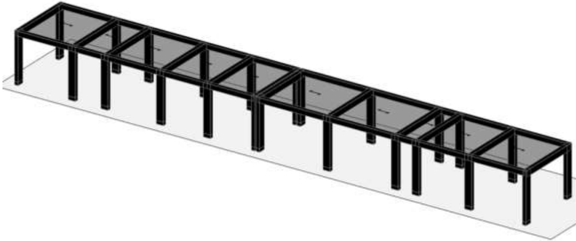
Figura 7.1-1 - Vista estrusa del modello.
