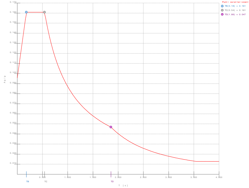
Spettro SLD
