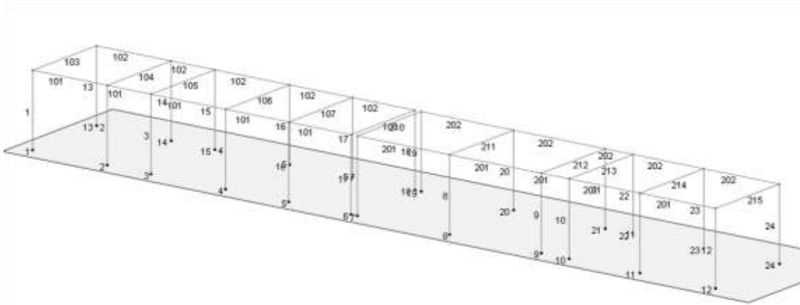
Figura 7.1-3 Modello di calcolo – numerazione aste.
