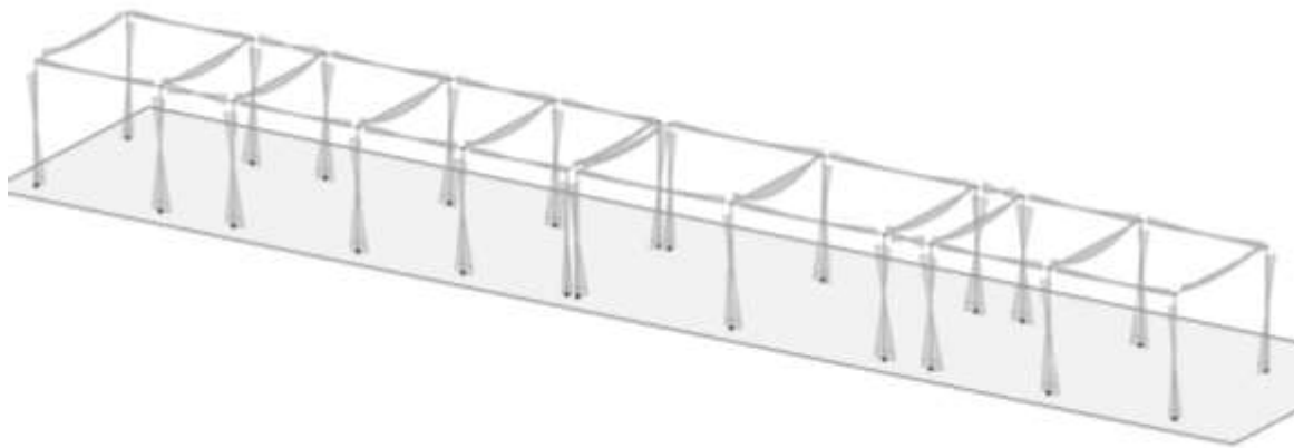
Figura 7.1-4 Diagramma dei momenti M3 – COMB_INV_SLV
