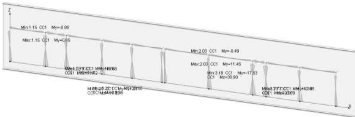
Figura 7.1-6 Diagramma dei momenti M3 - COMB_INV_SLV – Telaio di bordo
