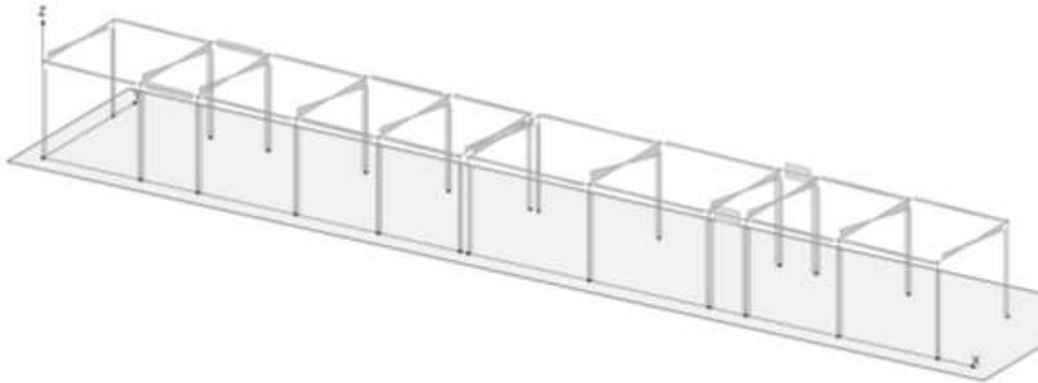
Figura 7.1-11 Diagramma del taglio V2 – COMB_INV_SLV.
