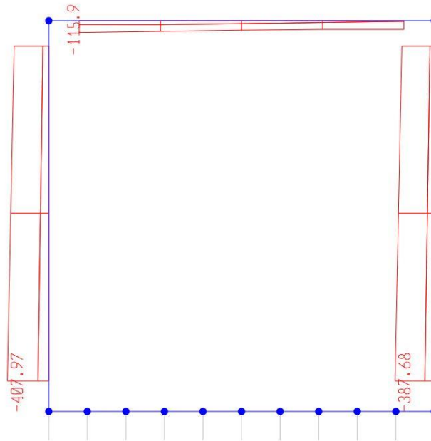
Sforzo normale
