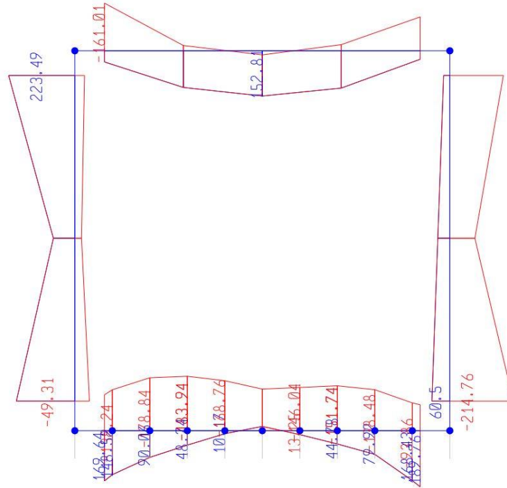
Momento Flettente
