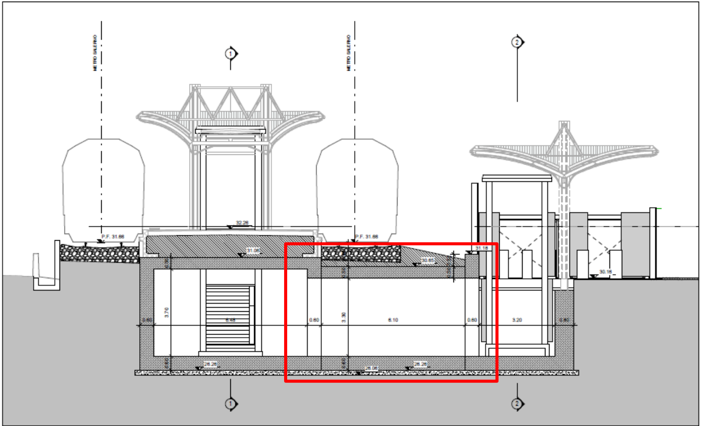
Figura 1b. Sezione trasversale dell'opera con individuazione del sottopasso
