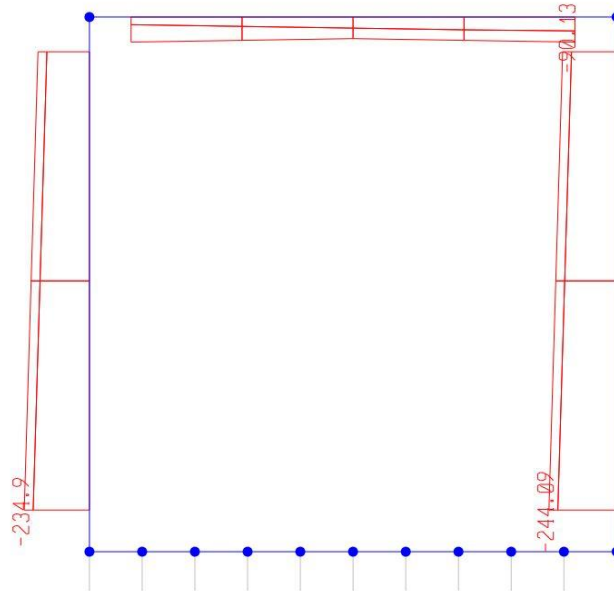
Sforzo normale
