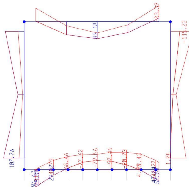
Momento Flettente
