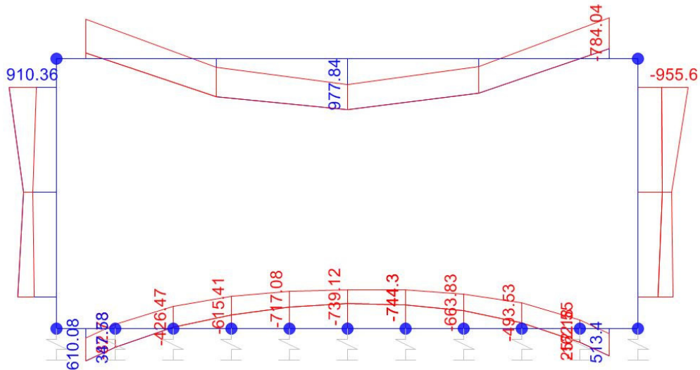
Momento Flettente
