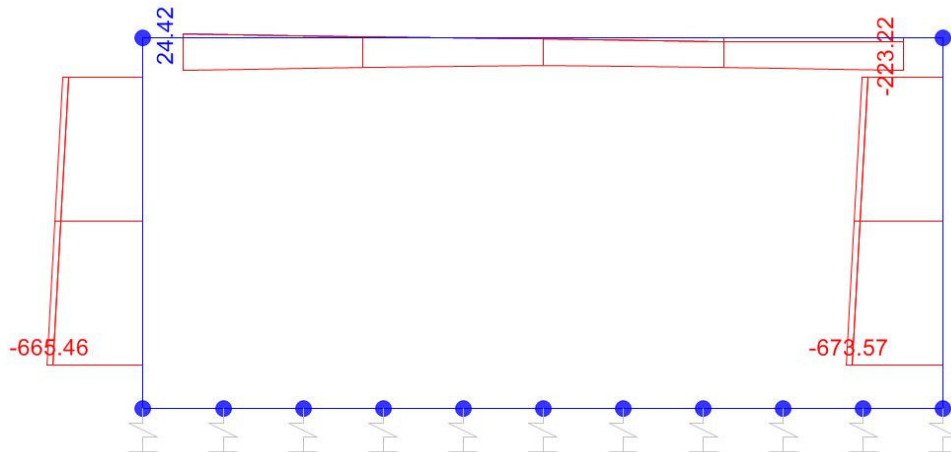
Sforzo normale
