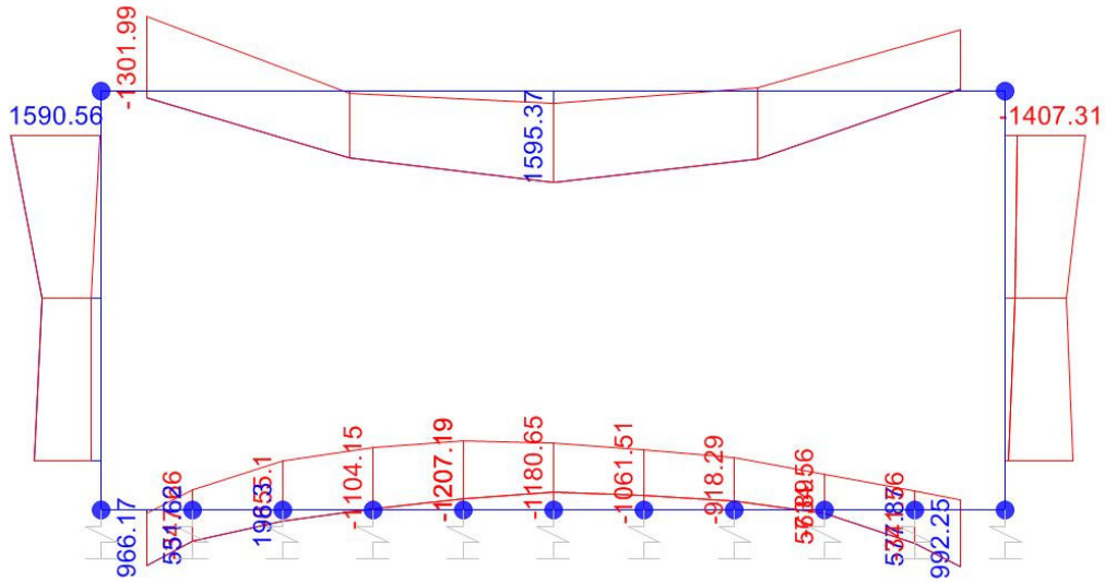
Momento Flettente
