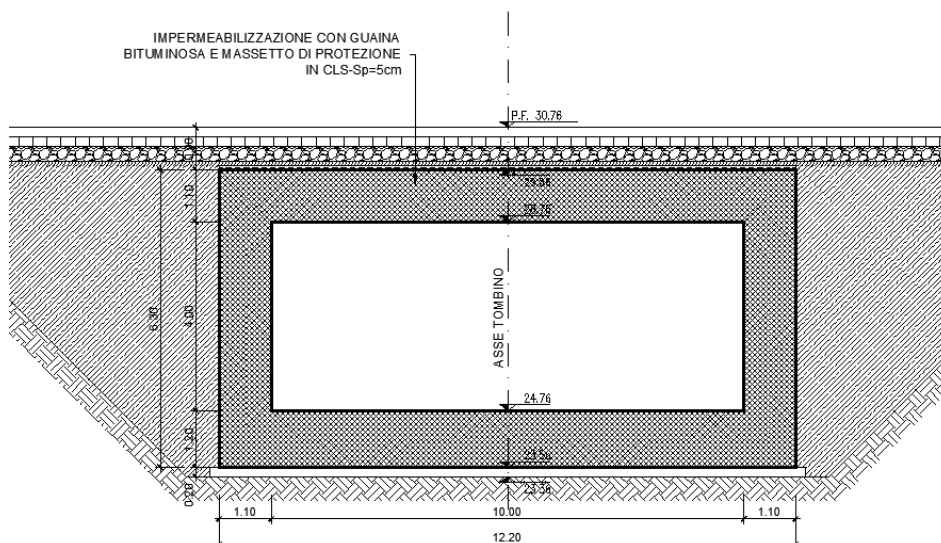
Figura 1c. Sezione trasversale dello scatolare
