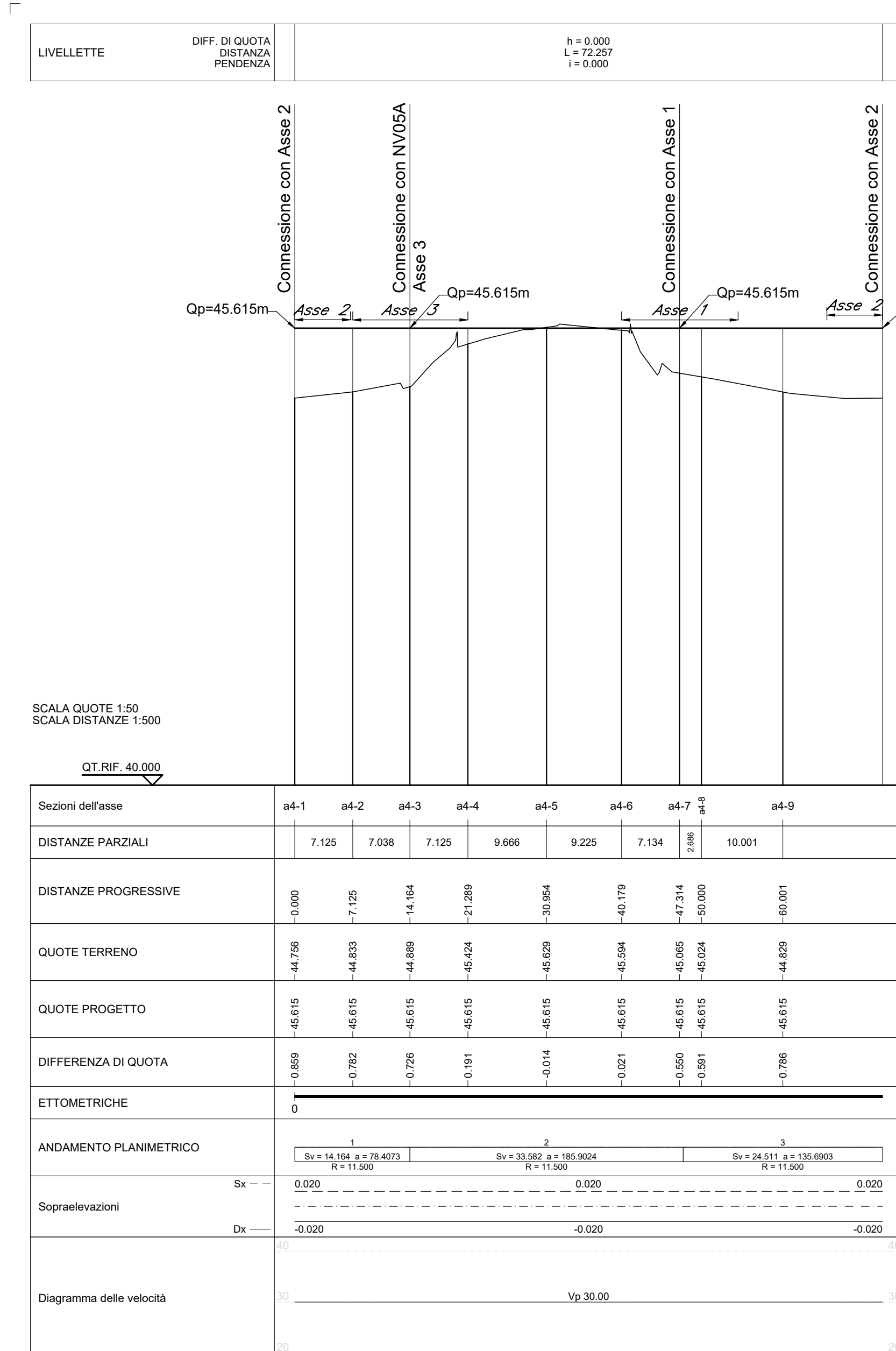
PROFILO - ASSE 4 SCALA 1:500
