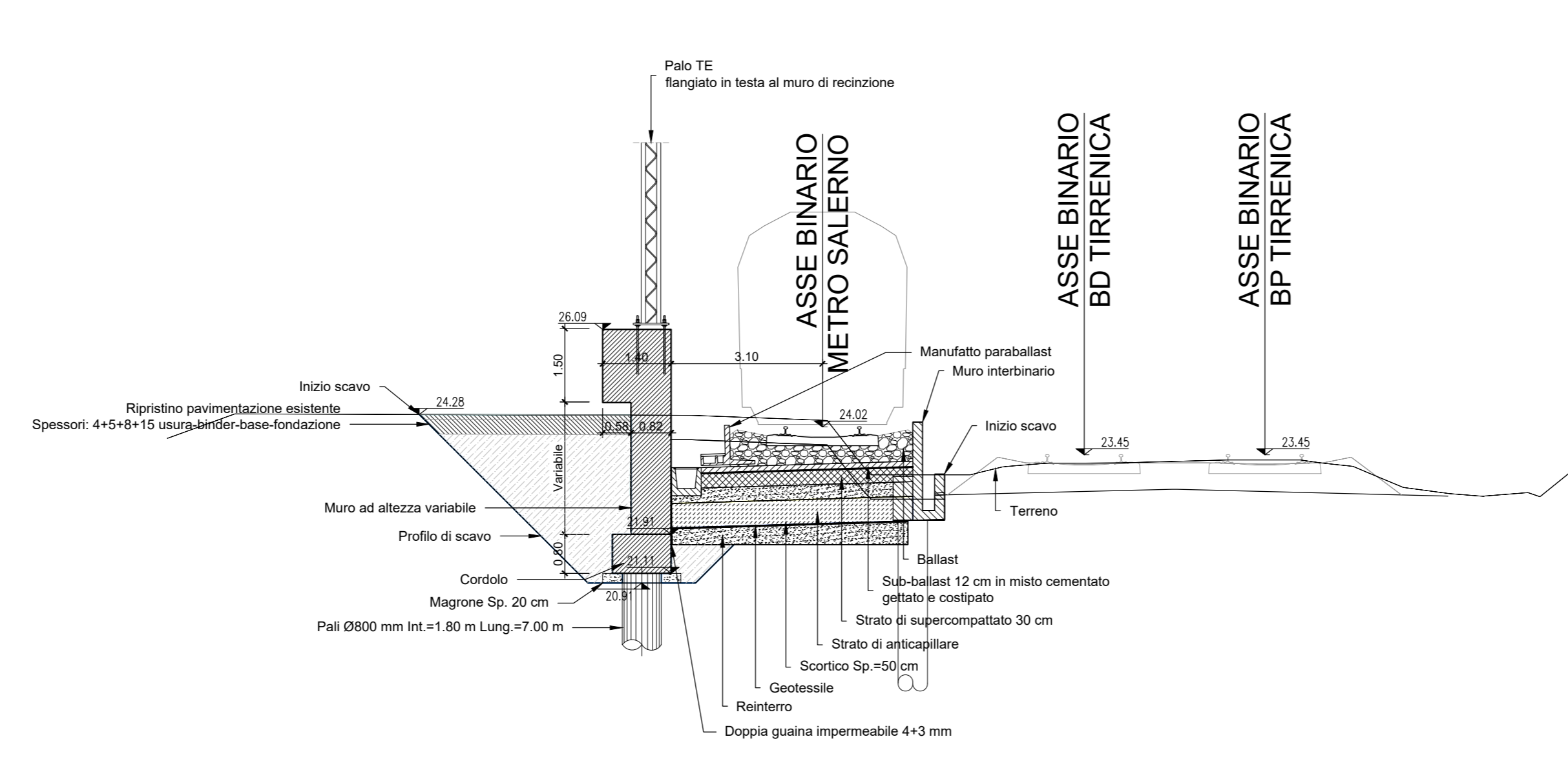
MURO DI RECINZIONE "TIPO 1" SEZIONE TRASVERSALE 47 - Km 2+250.00 Scala 1:100
