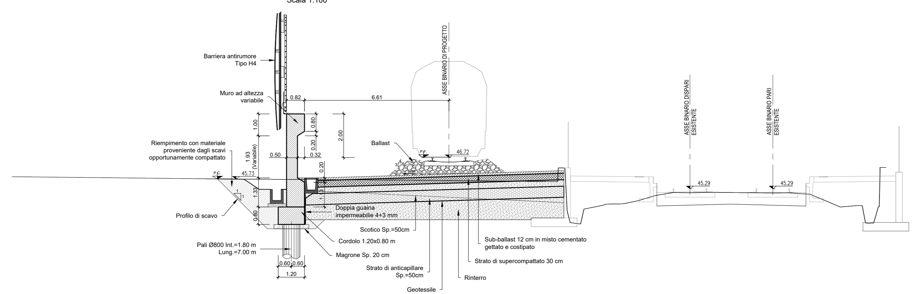
MURO DI RECINZIONE "TIPO 2" SEZIONE TRASVERSALE TIPICA A-A
