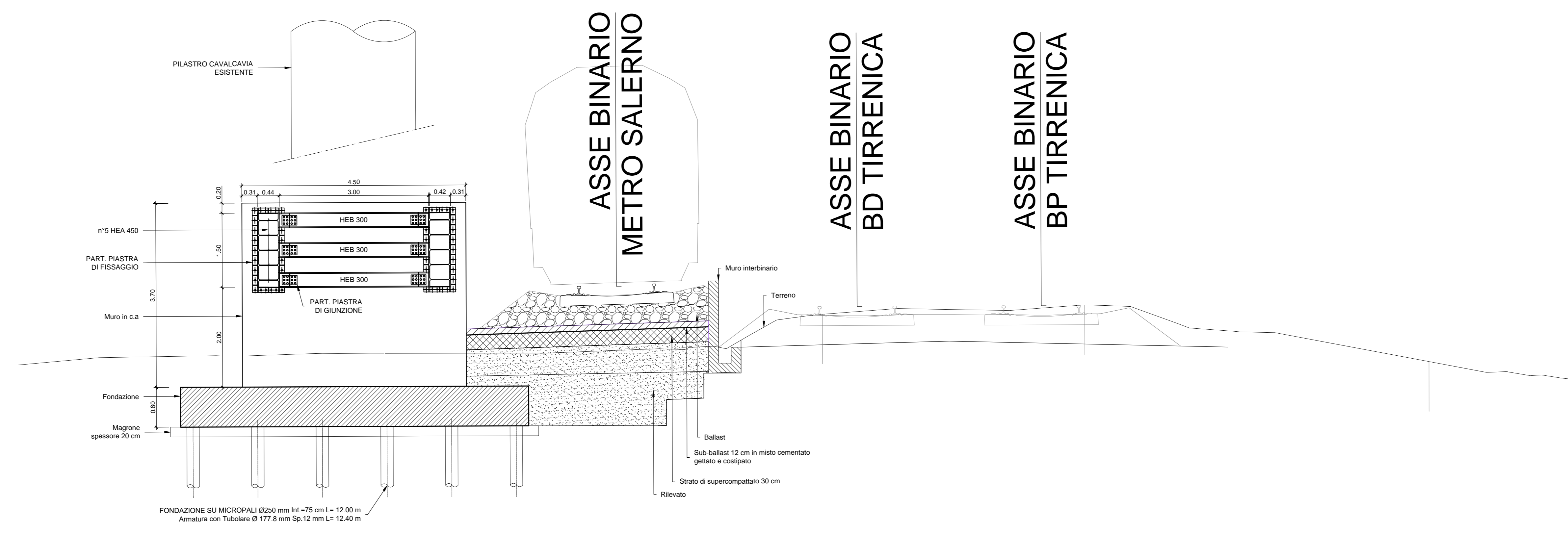
MURO di PROTEZIONE SEZIONE TRASVERSALE TIPICA A-A Scala 1:100
