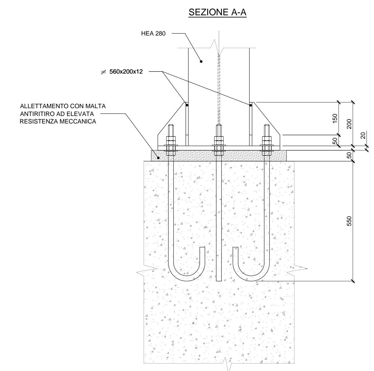
PIASTRA DI BASE Scala 1:10
