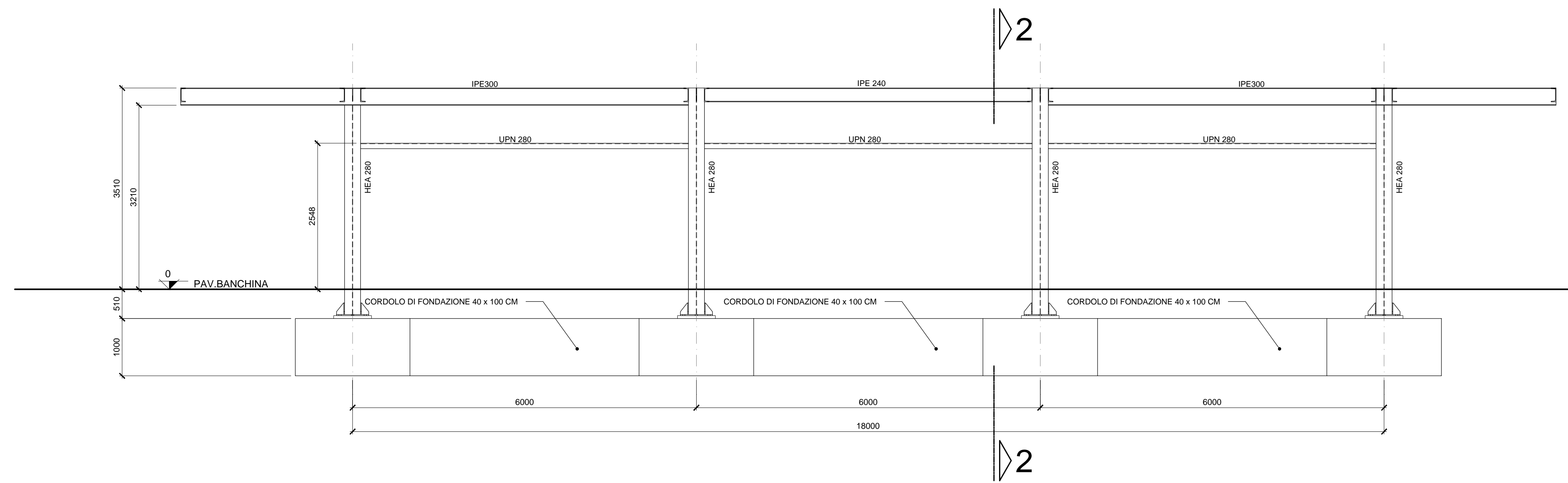
SEZIONE 1-1 Scala 1:50
