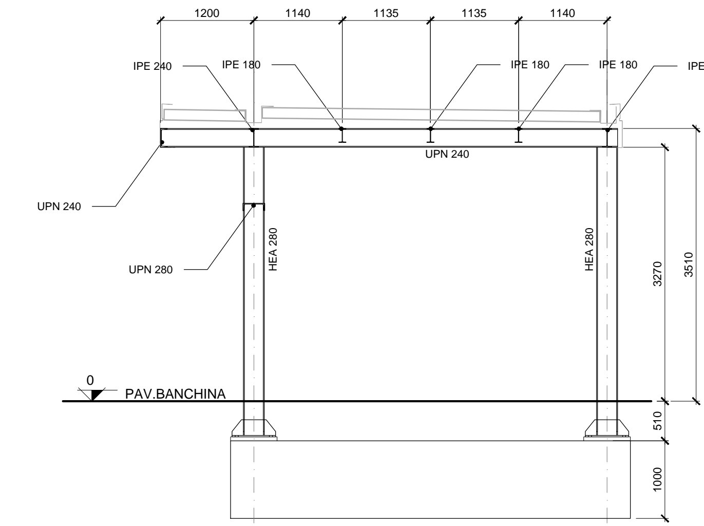
SEZIONE 2-2 Scala 1:50
