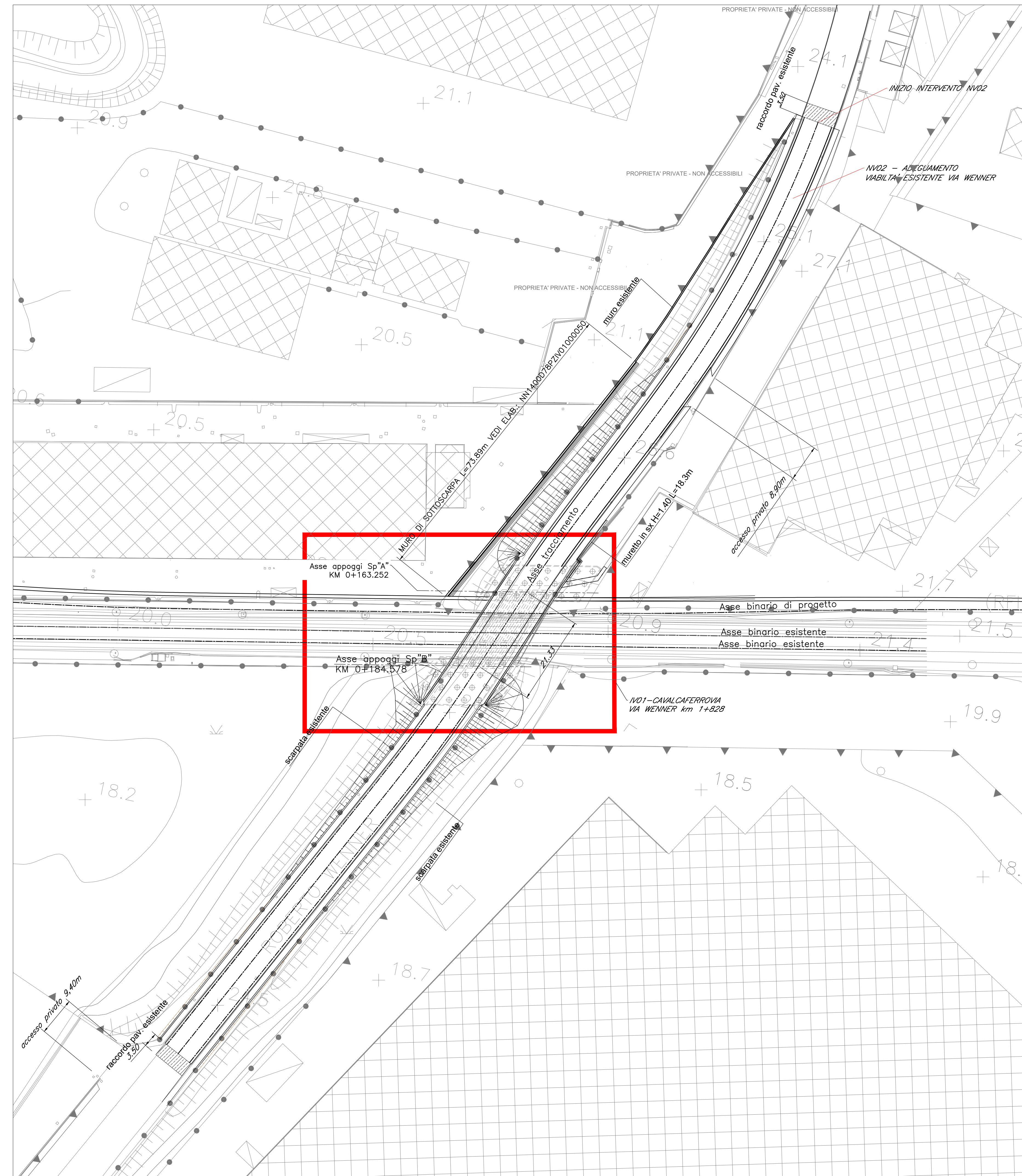
PLANIMETRIA GENERALE DI PROGETTO SCALA 1:500
