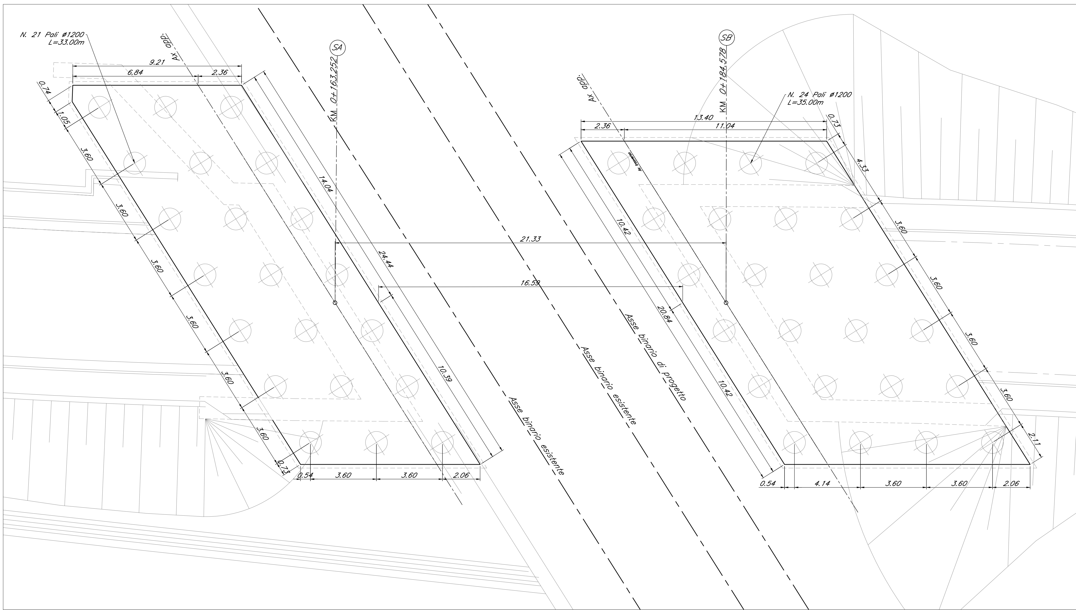
PIANTA IMPALCATO SCALA 1:100
