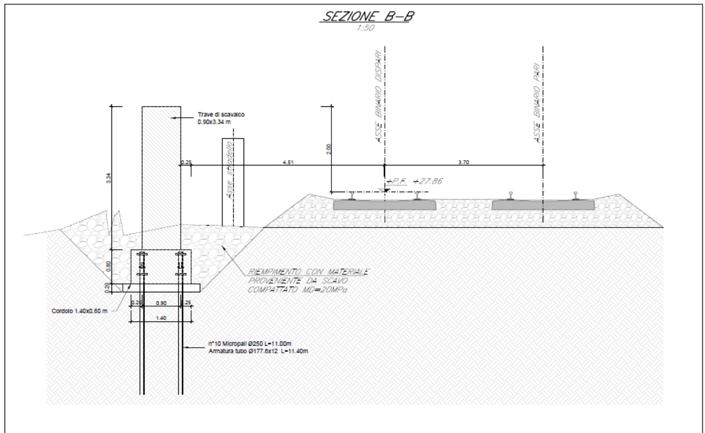
Figura 2 – Sezione Scavalco L = 26.50 m.
