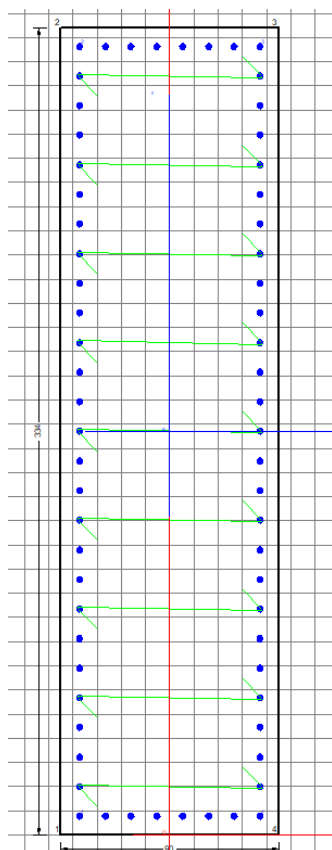
Figura 17 – Sezione della trave armata.
