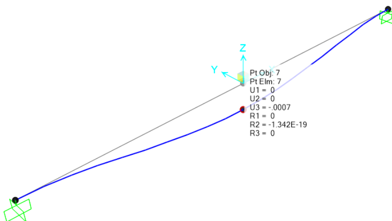
Figura 19 – Deformabilità modello incastro - incastro.
