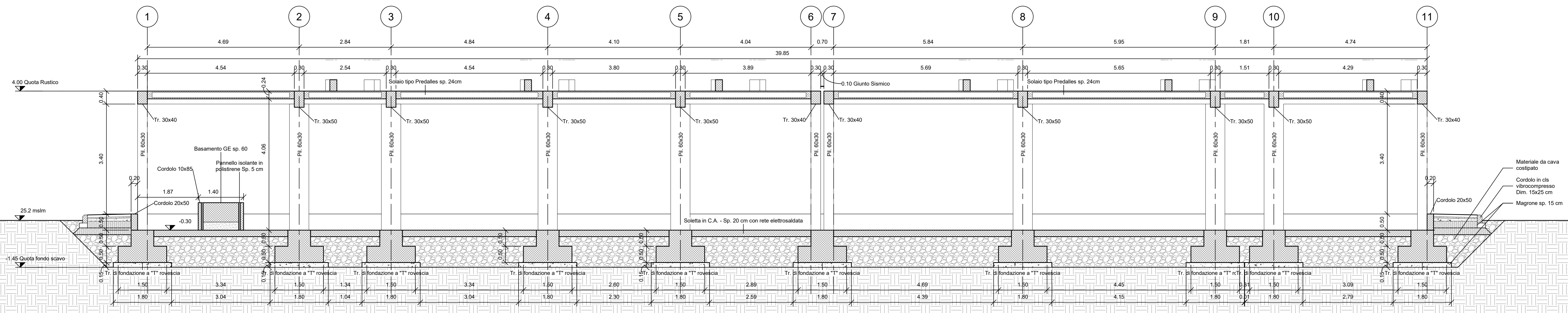
Sezione STR A-A' 1 : 50
