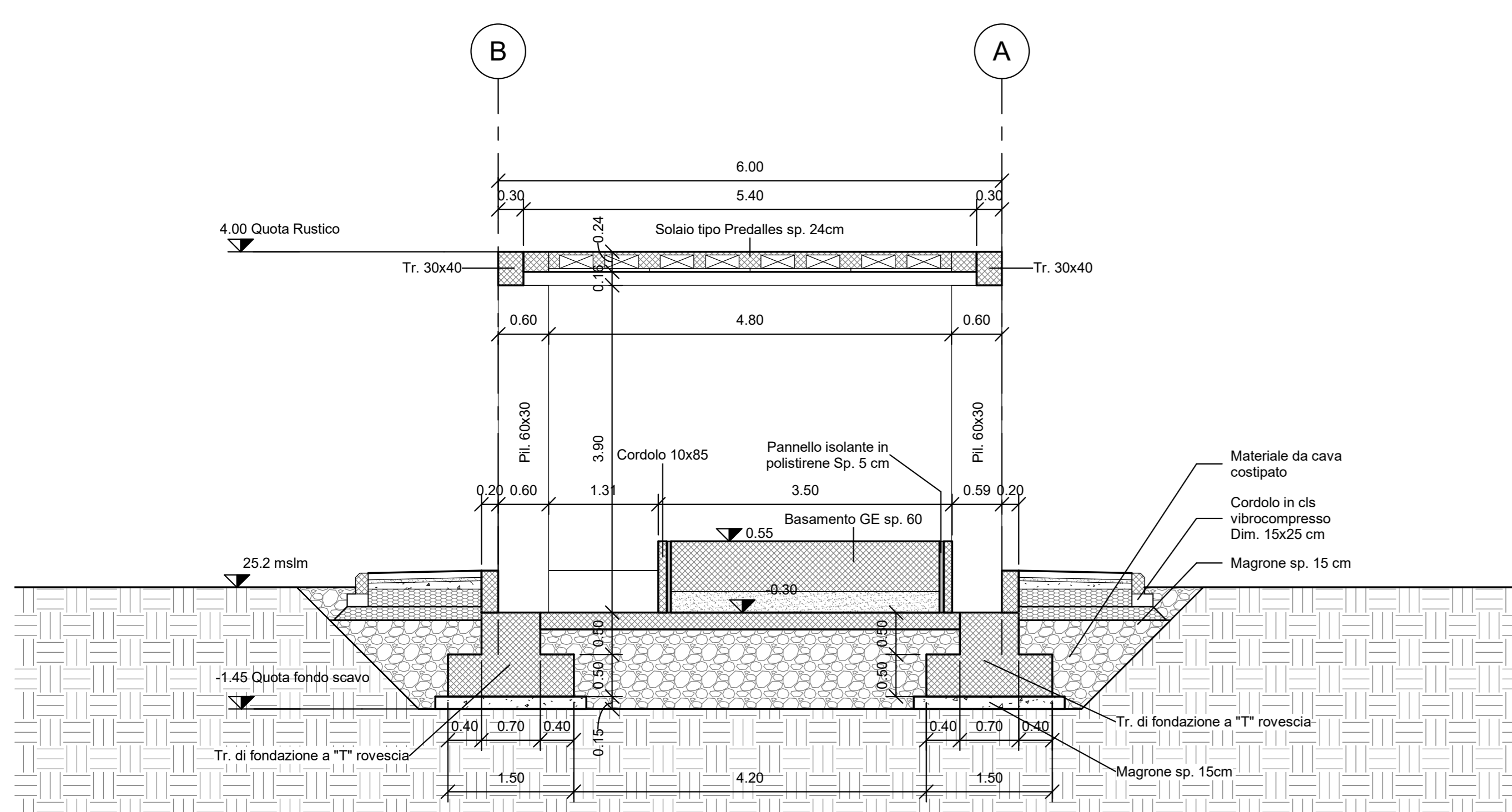
Sezione STR B-B' 1 : 50
