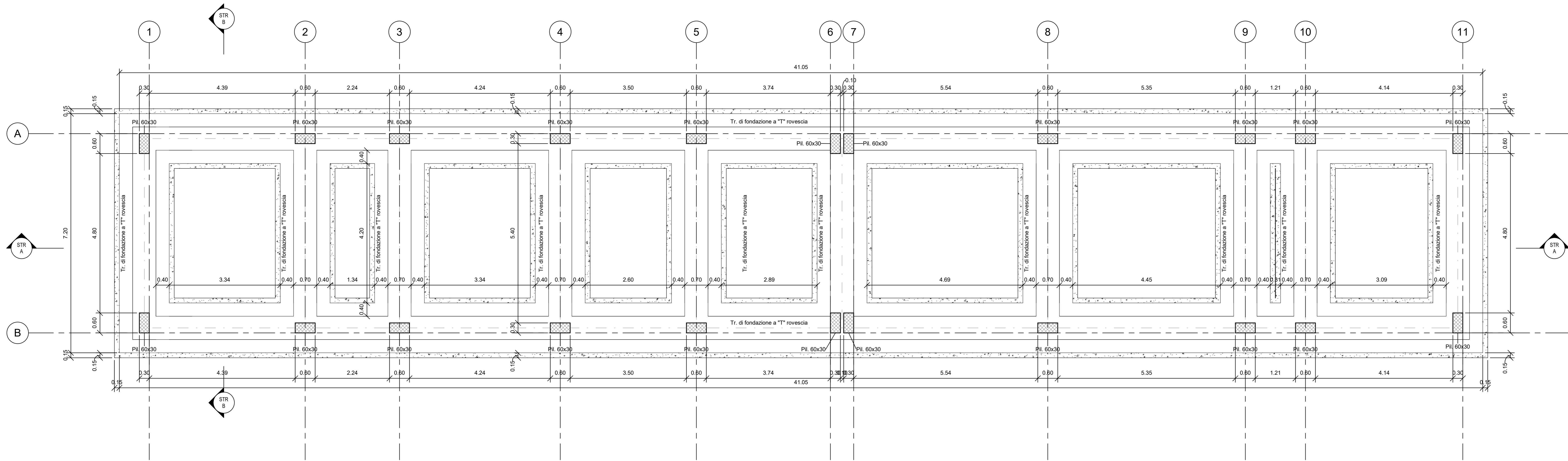
Carpenteria Fondazione 1 : 50
