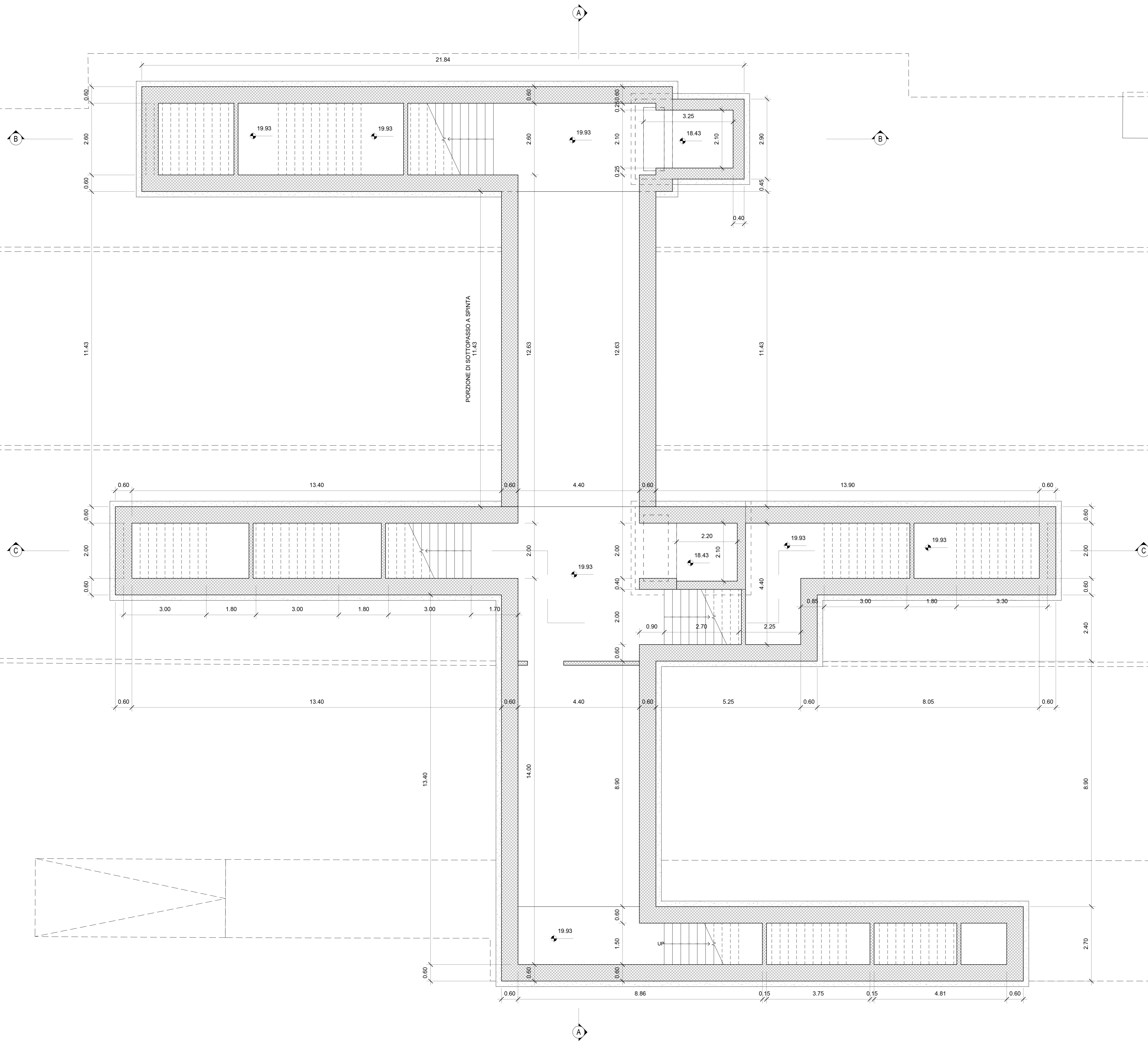
Pianta Sottopasso 1 : 50
