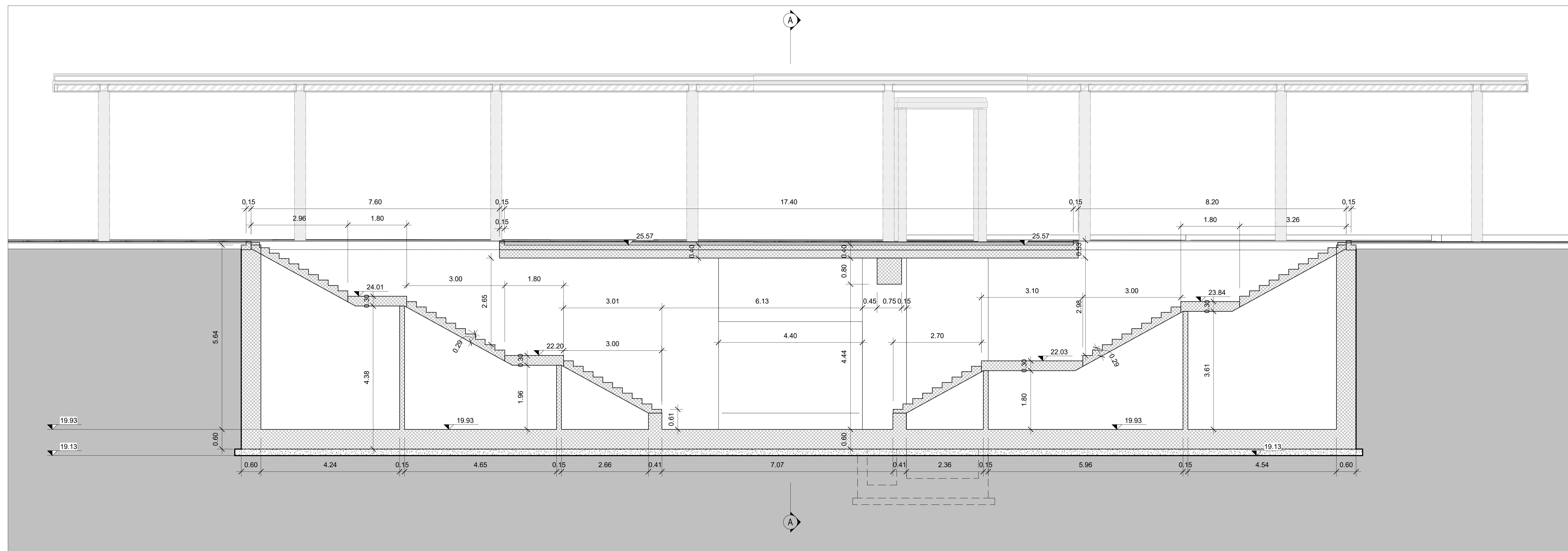
STR-Sez C 1 : 50
