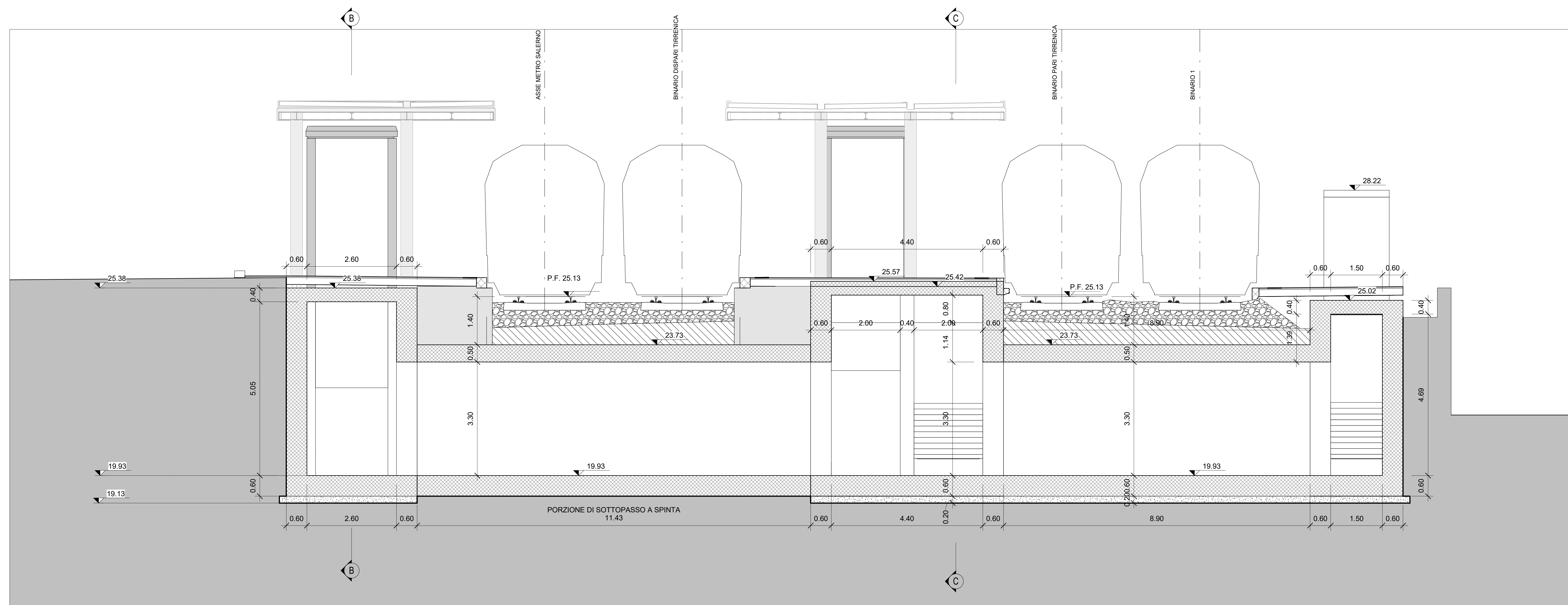
STR-Sez A 1 : 50
