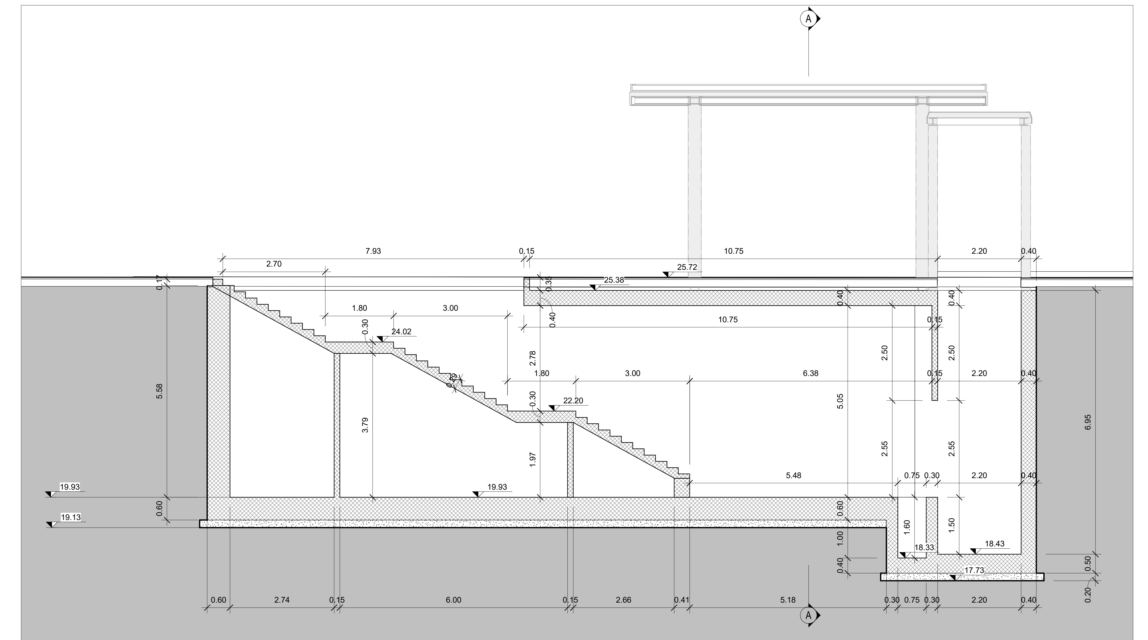
STR-Sez B 1 : 50
