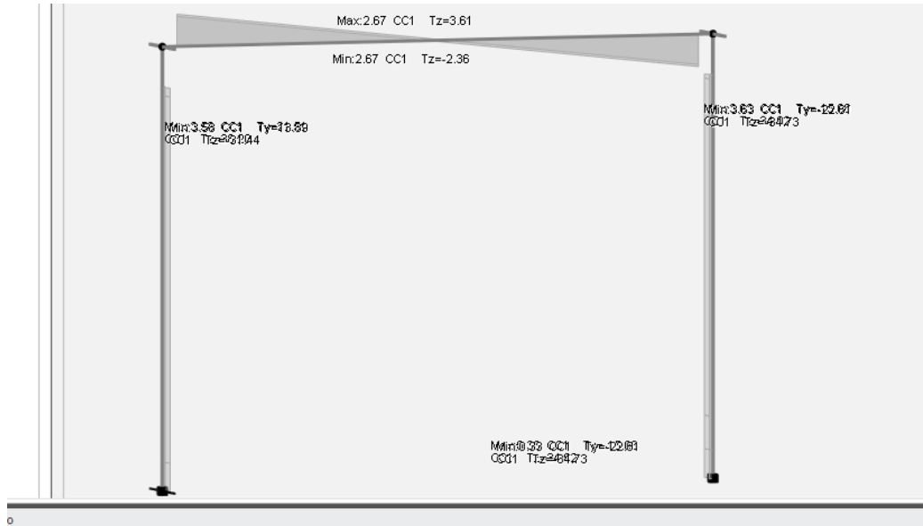
Figura 7.1-13 Diagramma del taglio V2 – COMB_INV_SLV – Telaio interno
