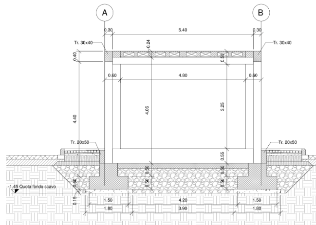
Sezione STR B-B'
