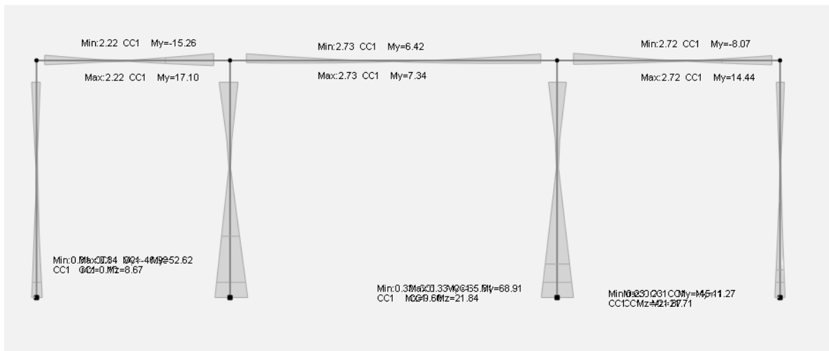
Figura 7.1-6 Diagramma dei momenti M3 - COMB_INV_SLV – Telaio di bordo
