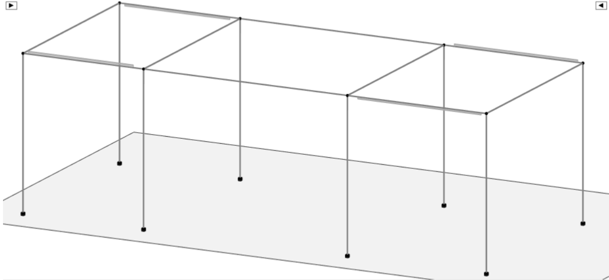
Figura 7.1-7 Diagramma della torsione T- COMB_INV_SLV.
