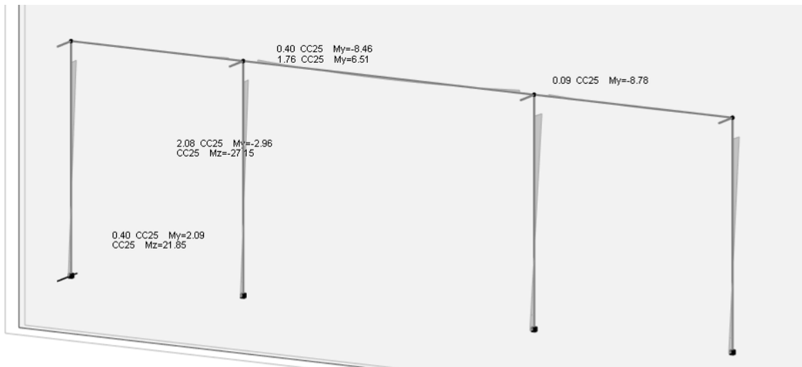
Figura 7.1-10 Diagramma dei momenti M3 – COMB_INV_SLU – Telaio di bordo.
