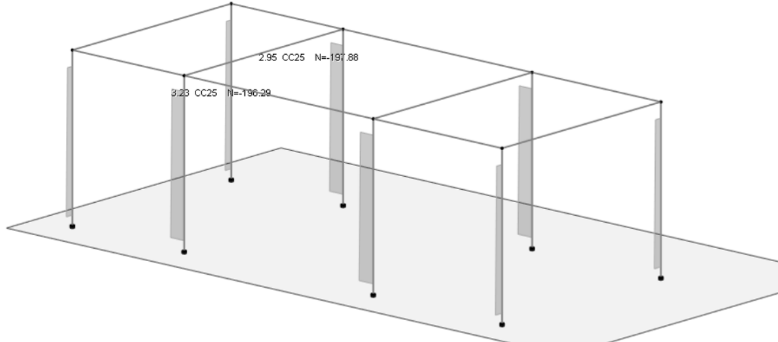
Figura 7.1-15 Diagramma dello sforzo assiale – COMB_INV_SLU
