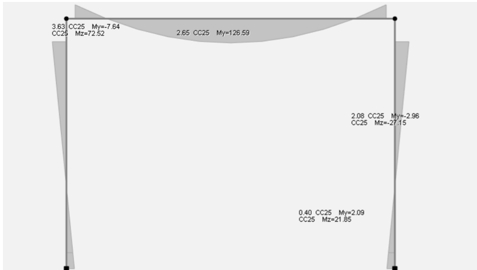
Figura 7.1-9 Diagramma dei momenti M3 – COMB_INV_SLU – Telaio interno.
