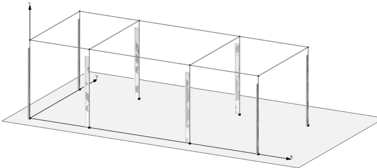
Figura 7.1-14 Diagramma dello sforzo assiale – COMB_INV_SLV
