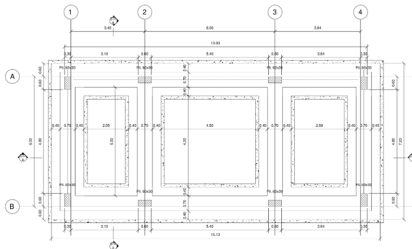
Carpenteria Fondazione 1 : 50
