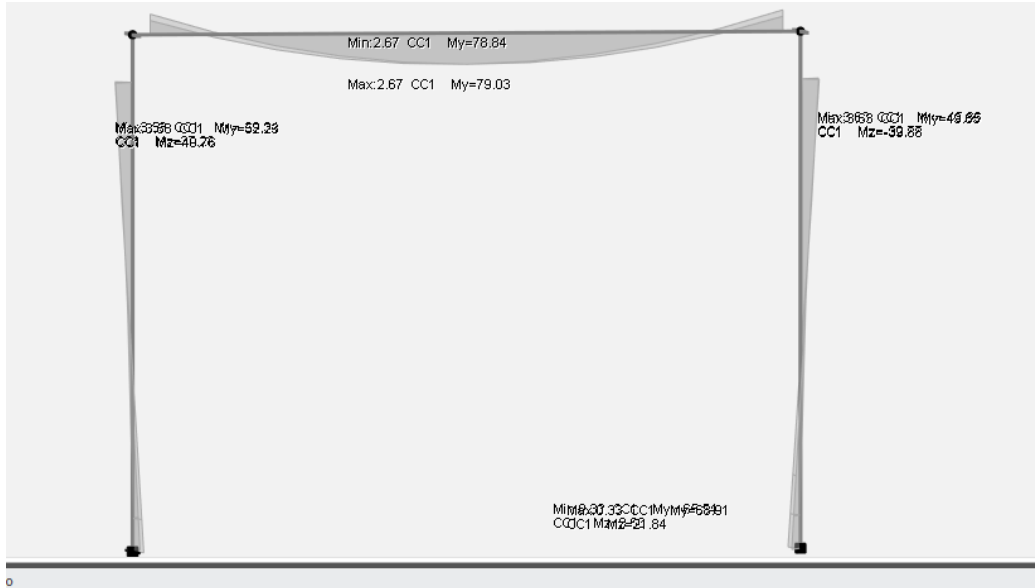
Figura 7.1-5 Diagramma dei momenti M3 - COMB_INV_SLV – Telaio interno
