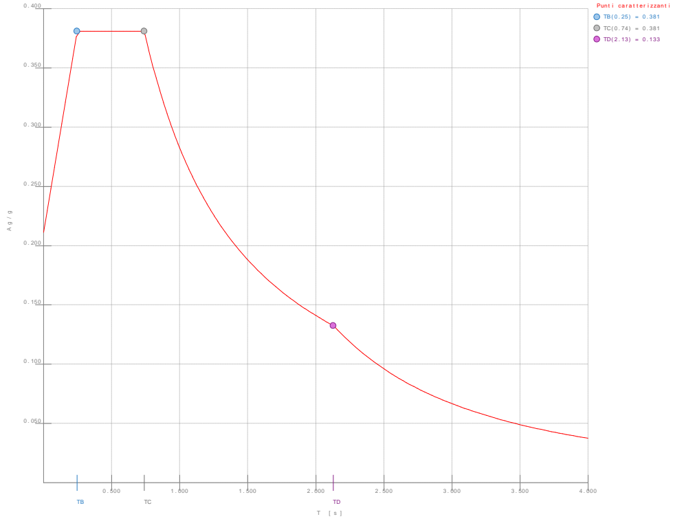
Spettro SND
