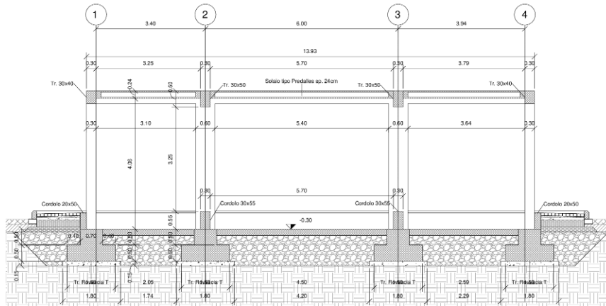
Sezione STR A-A'
