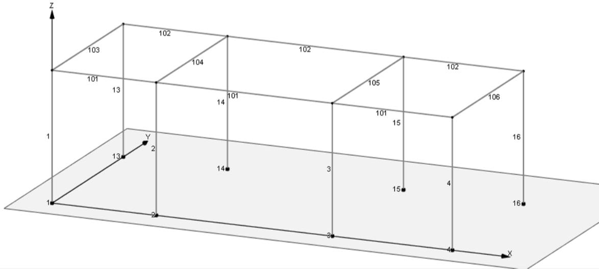
Figura 7.1-3 Modello di calcolo – numerazione aste.
