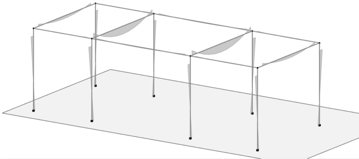
Figura 7.1-8 Diagramma dei momenti M3- COMB_INV_SLU
