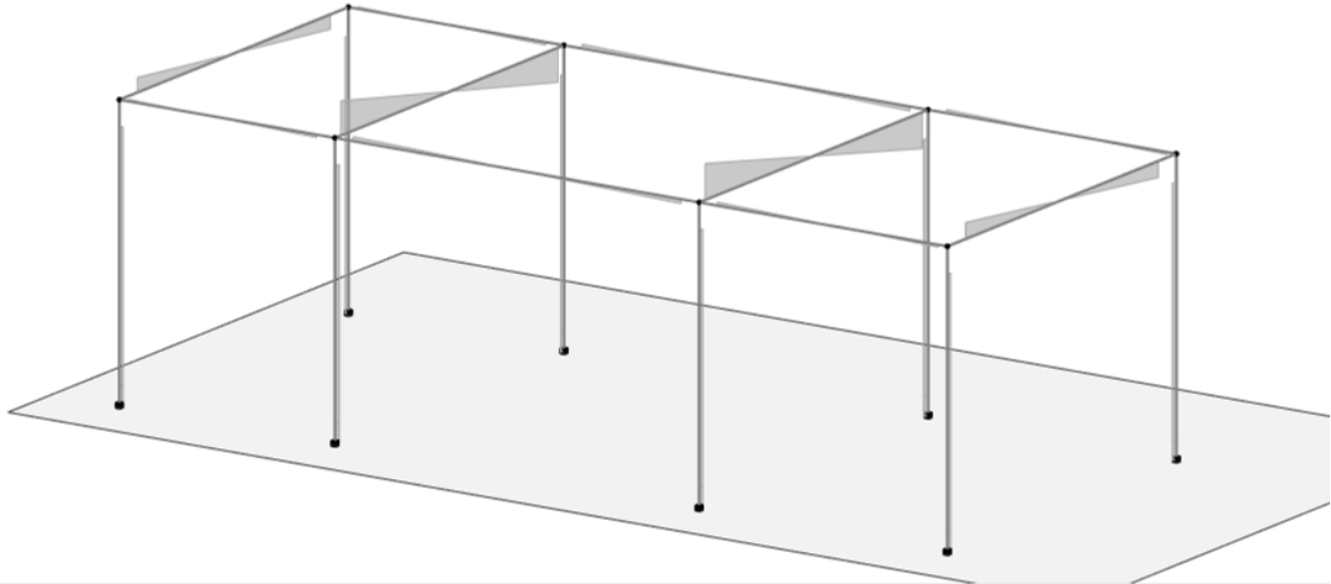
Figura 7.1-11 Diagramma del taglio V2 – COMB_INV_SLU.
