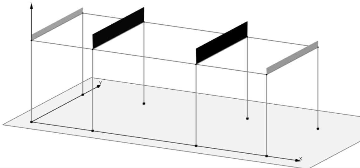
Figura 7.1-16 Schemi di carico - Permanenti solai
