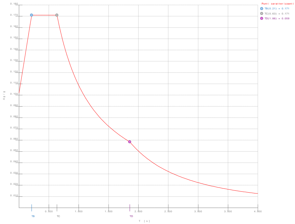
Spettro SLD
