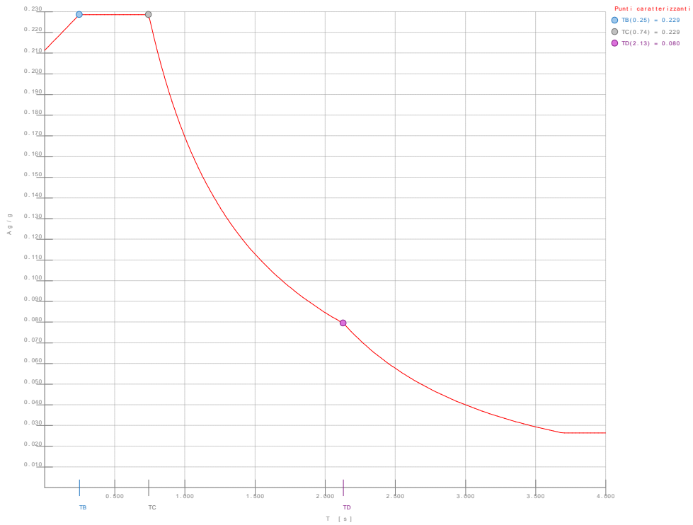
Spettro SLV
