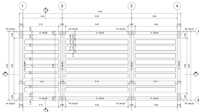
Carpenteria Copertura 1 : 50
