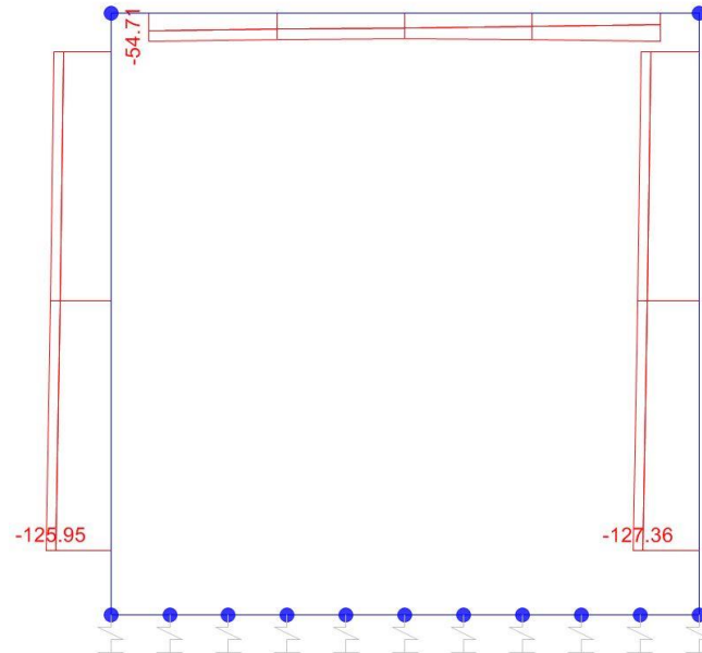
Sforzo normale
