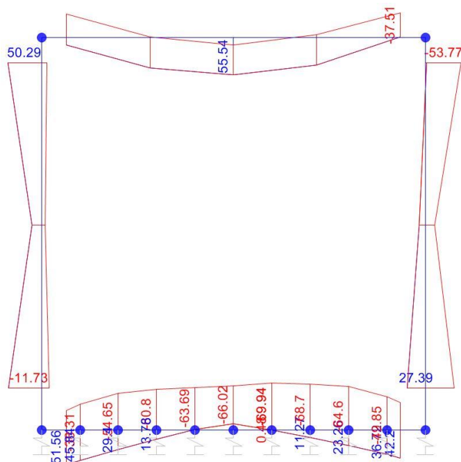
Momento Flettente
