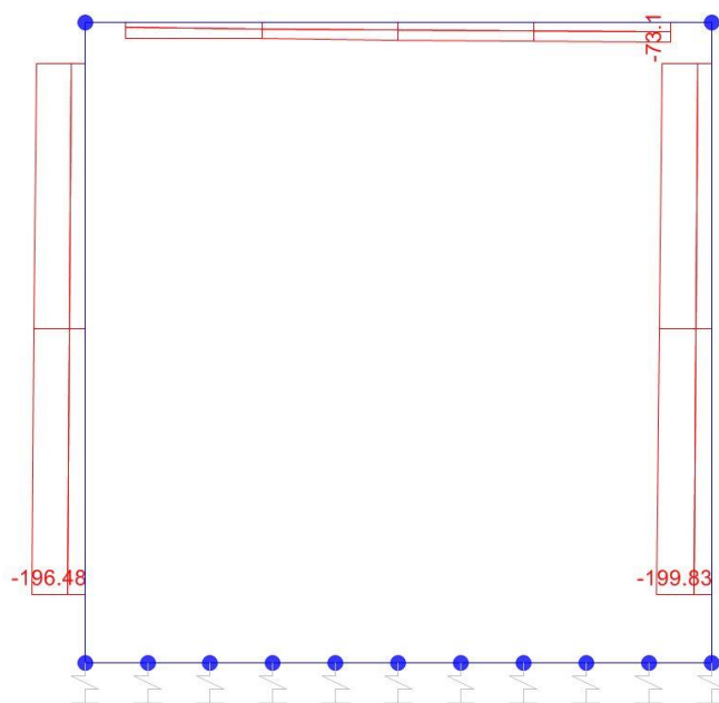
Sforzo normale
