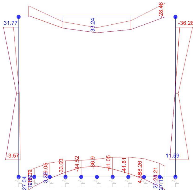
Momento Flettente
