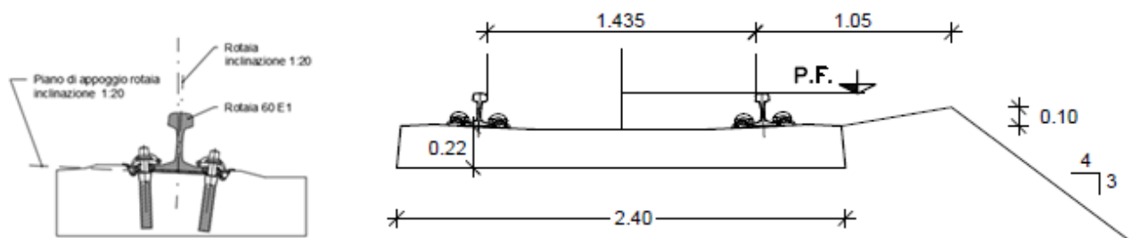
Figura 2 - Telaio del binario costituito da: Traversa RFI-240 con attacco elastico; modulo cm 60 e Rotaia 60 E1 inclinata 1:20
