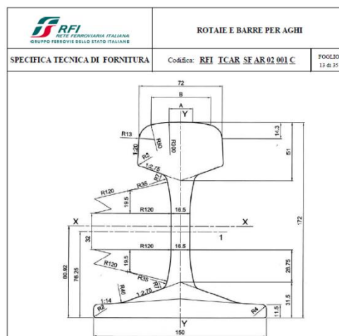
Figura 1 - Rotaia 60E1 (60 UIC)
