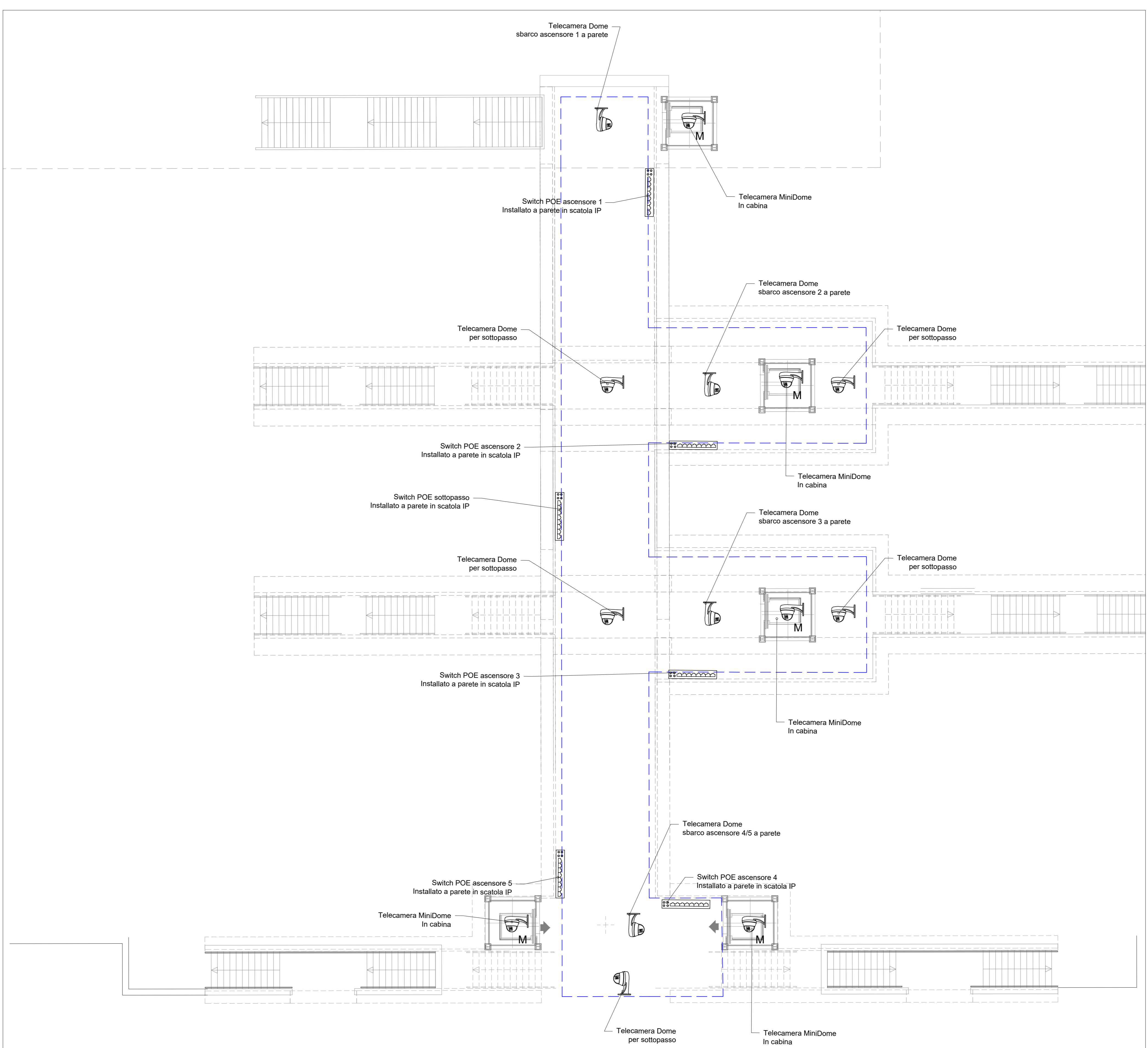
PLANIMETRIA QUOTA ASCENSORI scala 1:100
