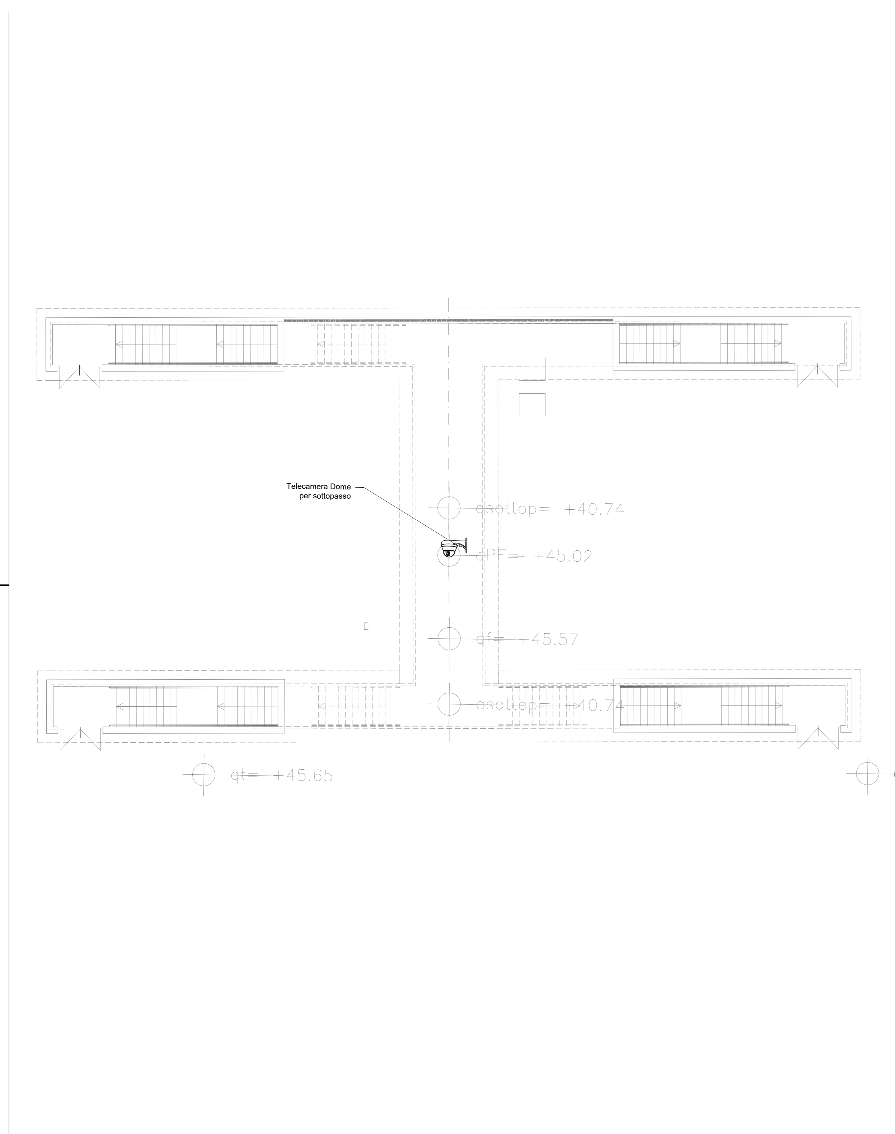
PLANIMETRIA QUOTA SOTTOPASSO LATO FERMATA scala 1:100
