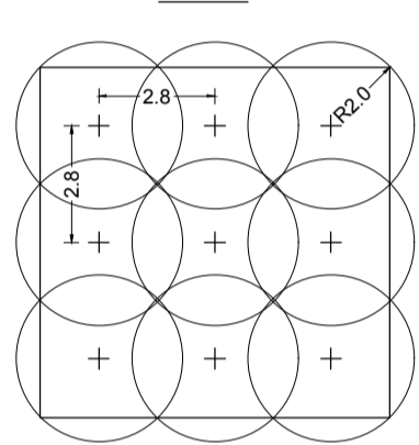
Schema di esecuzione bonifica profonda
