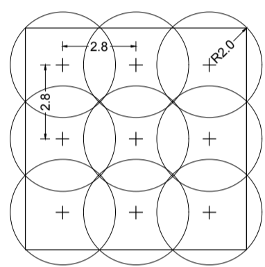
Schema di esecuzione bonifica profonda
