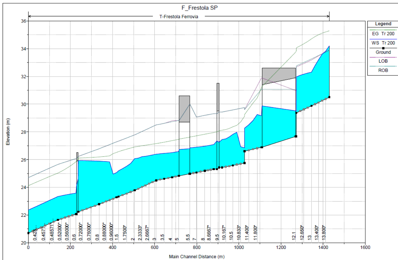
Figura 8 - Profilo di corrente Tr 200 anni Stato di Progetto IN26 Fosso Frestola pk 6+054.
