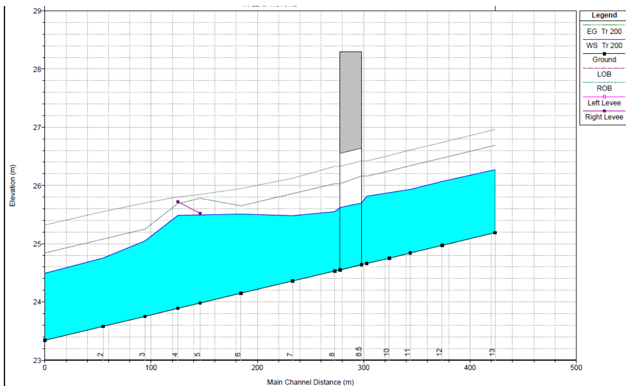
Figura 7 - Profilo di corrente Tr 200 anni Stato di Progetto IN23 pk 5+624.
