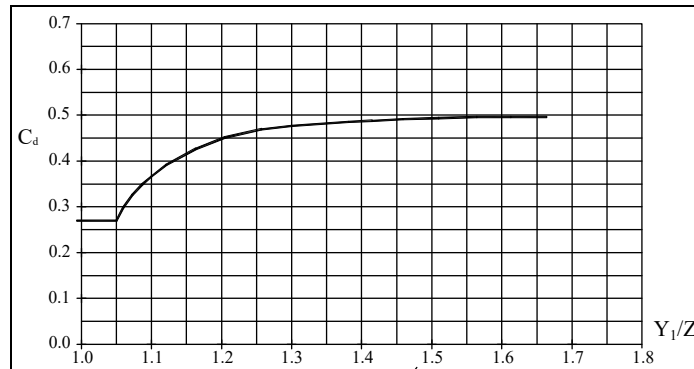
Figura 7 – Diagramma per la stima del coefficiente di deflusso Cd
