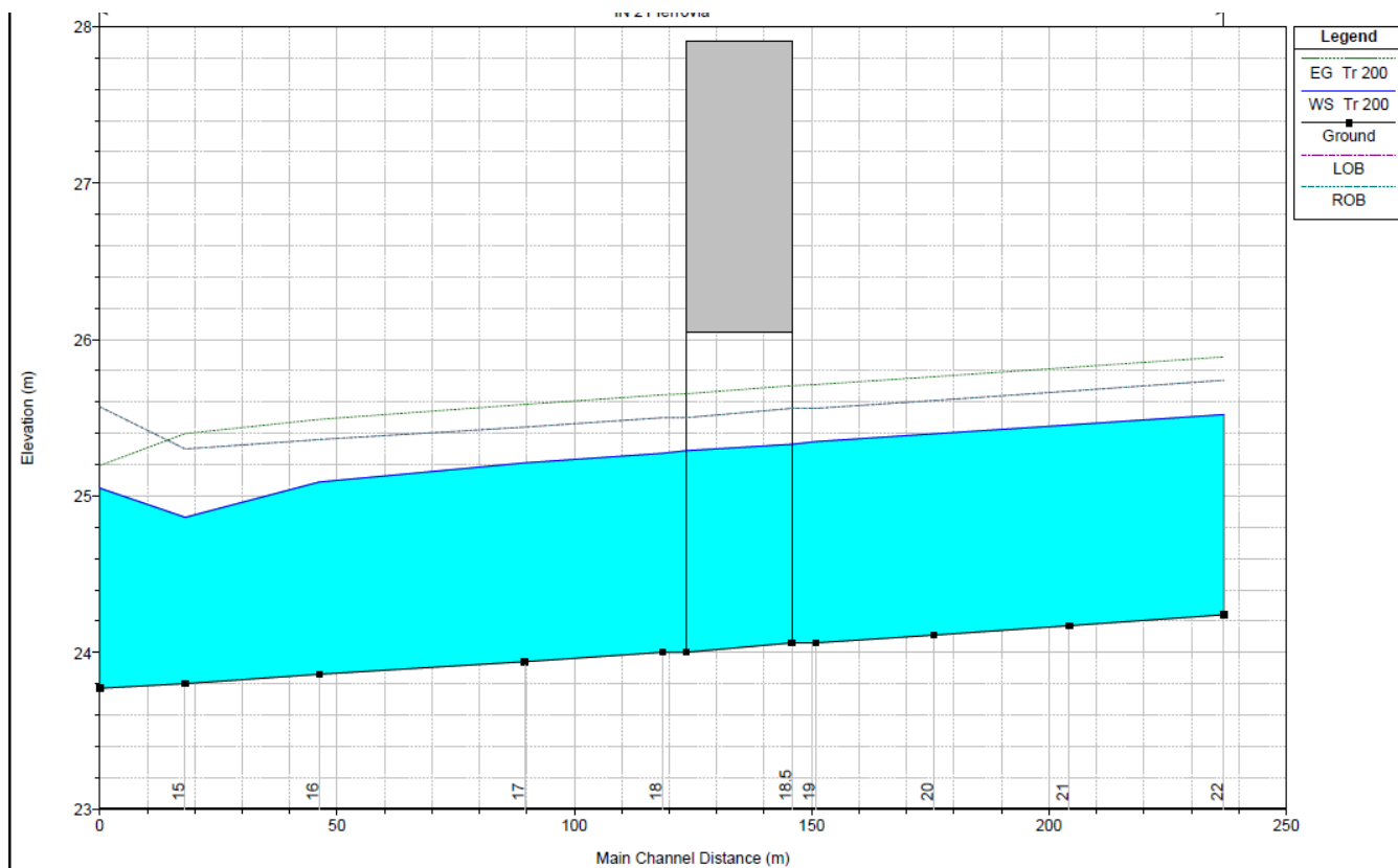
Figura 6 - Profilo di corrente Tr 200 anni Stato di Progetto IN22 pk 5+548.
