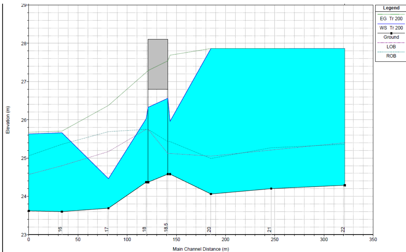
Figura 3 - Profilo di corrente Tr 200 anni Stato Attuale IN 22 pk 5+439.
