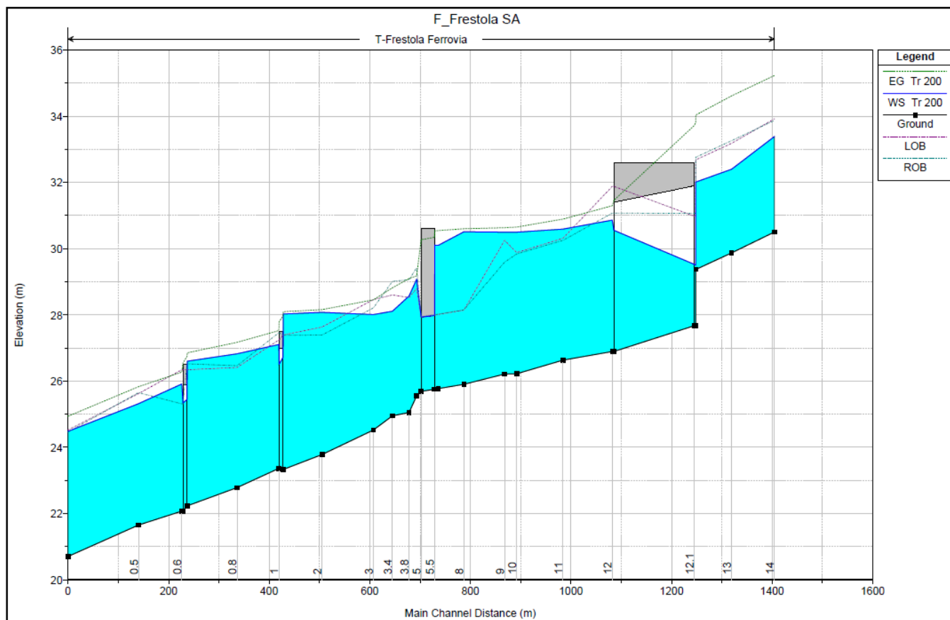
Figura 5 - Profilo di corrente Tr 200 anni Stato Attuale IN26 Fosso Frestola pk 6+037.
