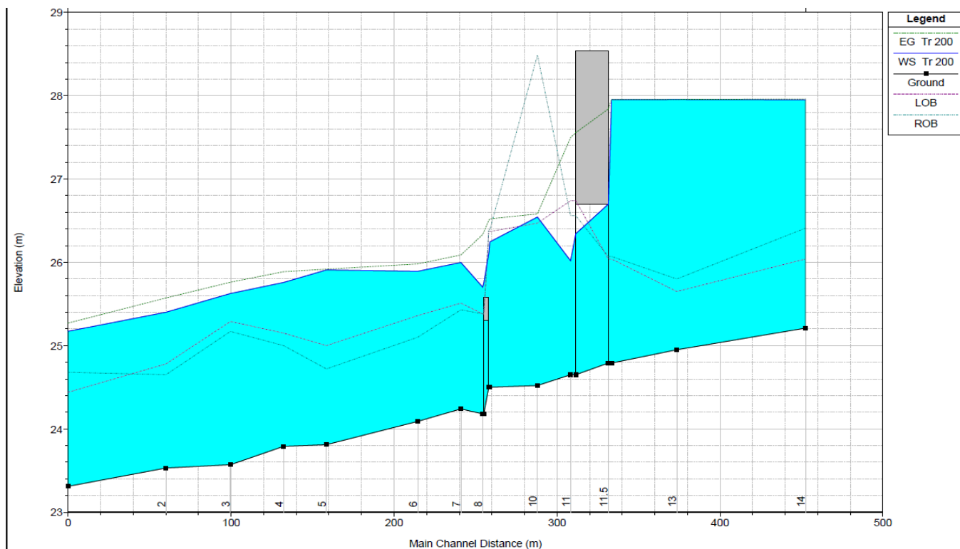
Figura 4 - Profilo di corrente Tr 200 anni Stato Attuale IN23 pk 5+613.
