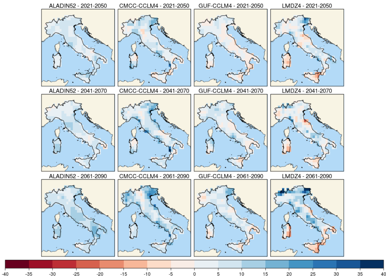
Figura 10 - Precipitazione massima giornaliera (mm), scenario RCP8.5.
