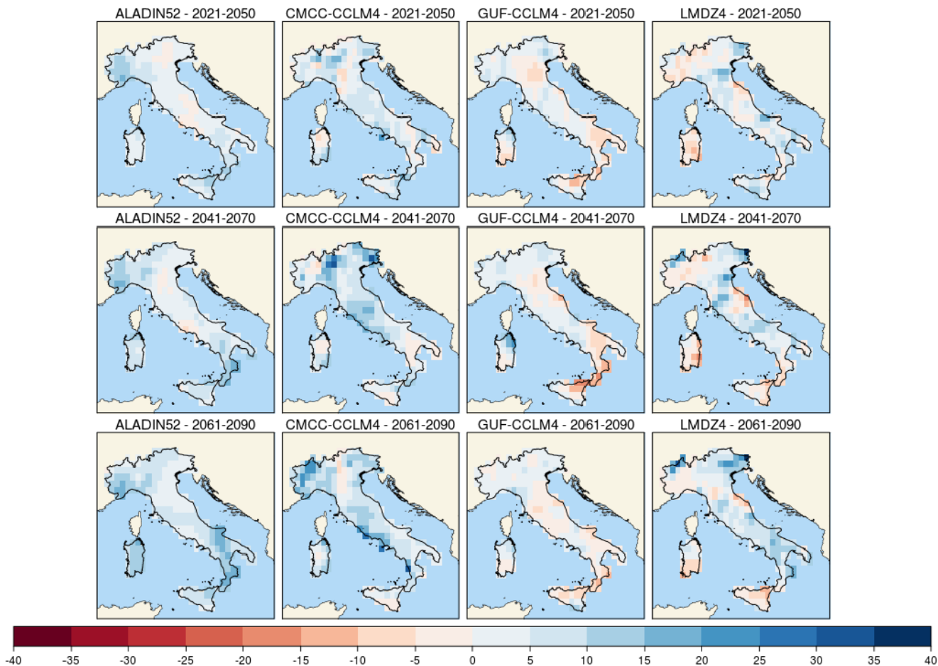
Figura 9 - Precipitazione massima giornaliera (mm), scenario RCP4.5.
