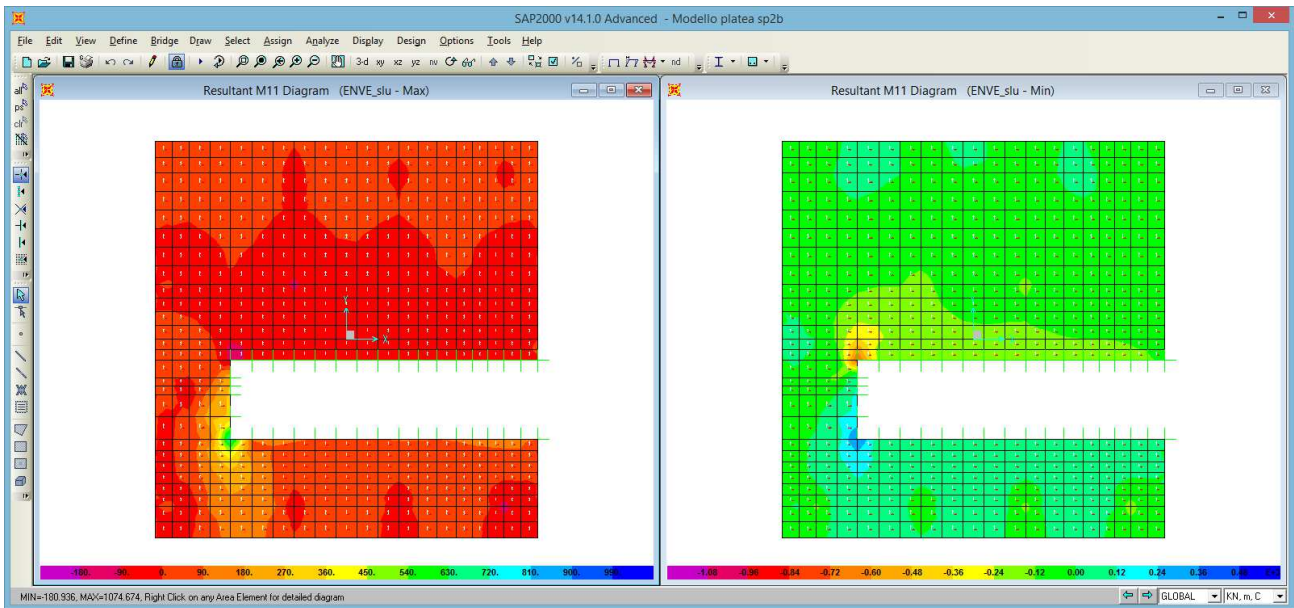
Figura 64 - Azioni sollecitanti M11 platea di fondazione spalla 2b (ENVE_slv)
