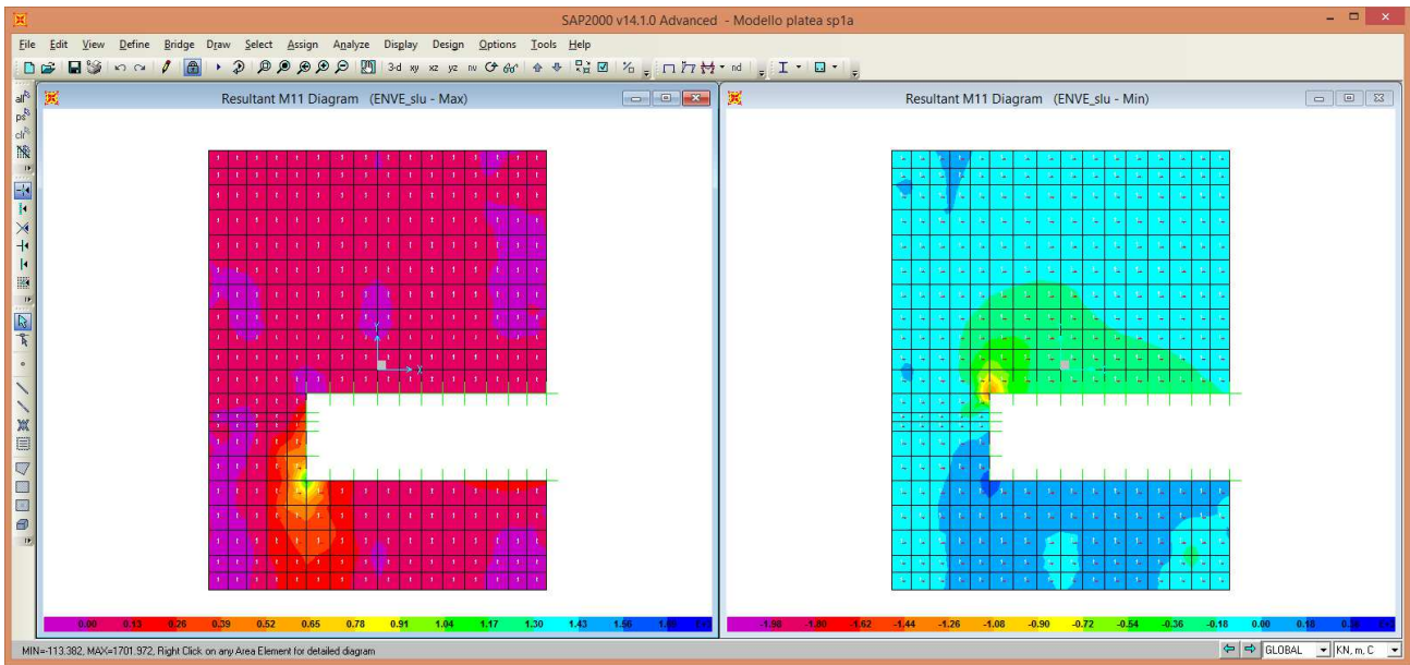
Figura 19 - Azioni sollecitanti M11 platea di fondazione spalla 1a (ENVE_slv)
