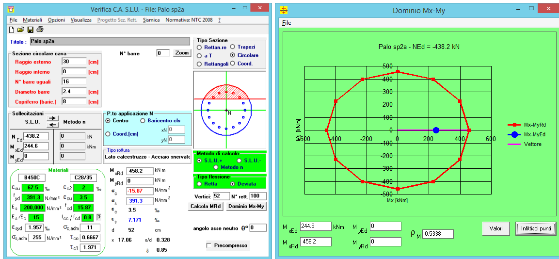
Figura 3 – Verifica a tensoflessione palo di fondazione spalla 2a - minimo FS
