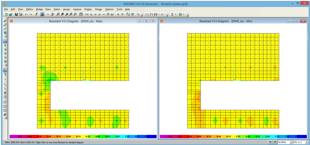
Figura 75 – Verifica a taglio platea di fondazione spalla 2b (ENVE_slu) - trasversale
