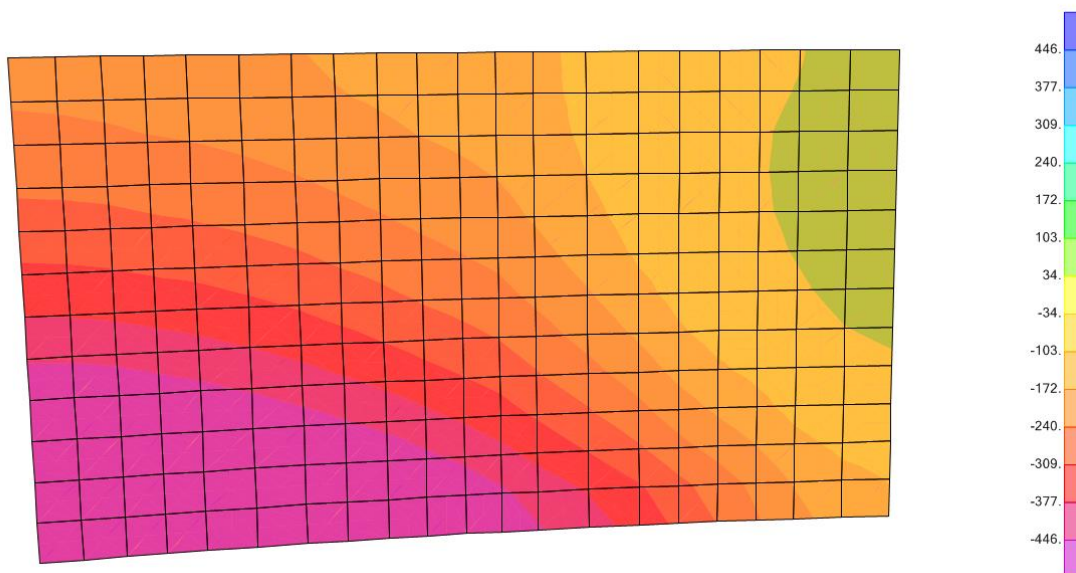
Figura 36: P120SX – andamento di V23 ed evidenziazione (in fucsia) delle zone in cui è necessario predisporre armature a taglio.
