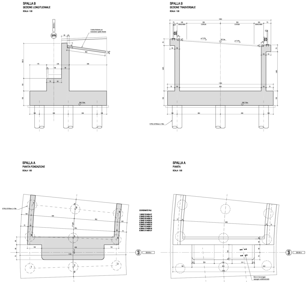
Figura 7: Casseratura Spalla B.
