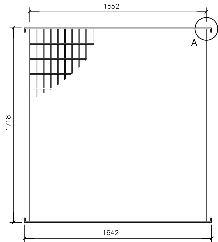
Sez. A-A
