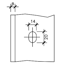
Particolare D'
