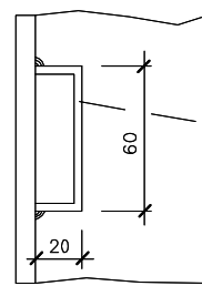
Particolare E
