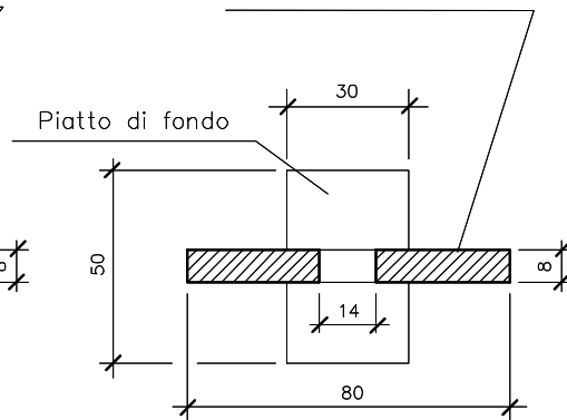
Profilato piatto 80x8
