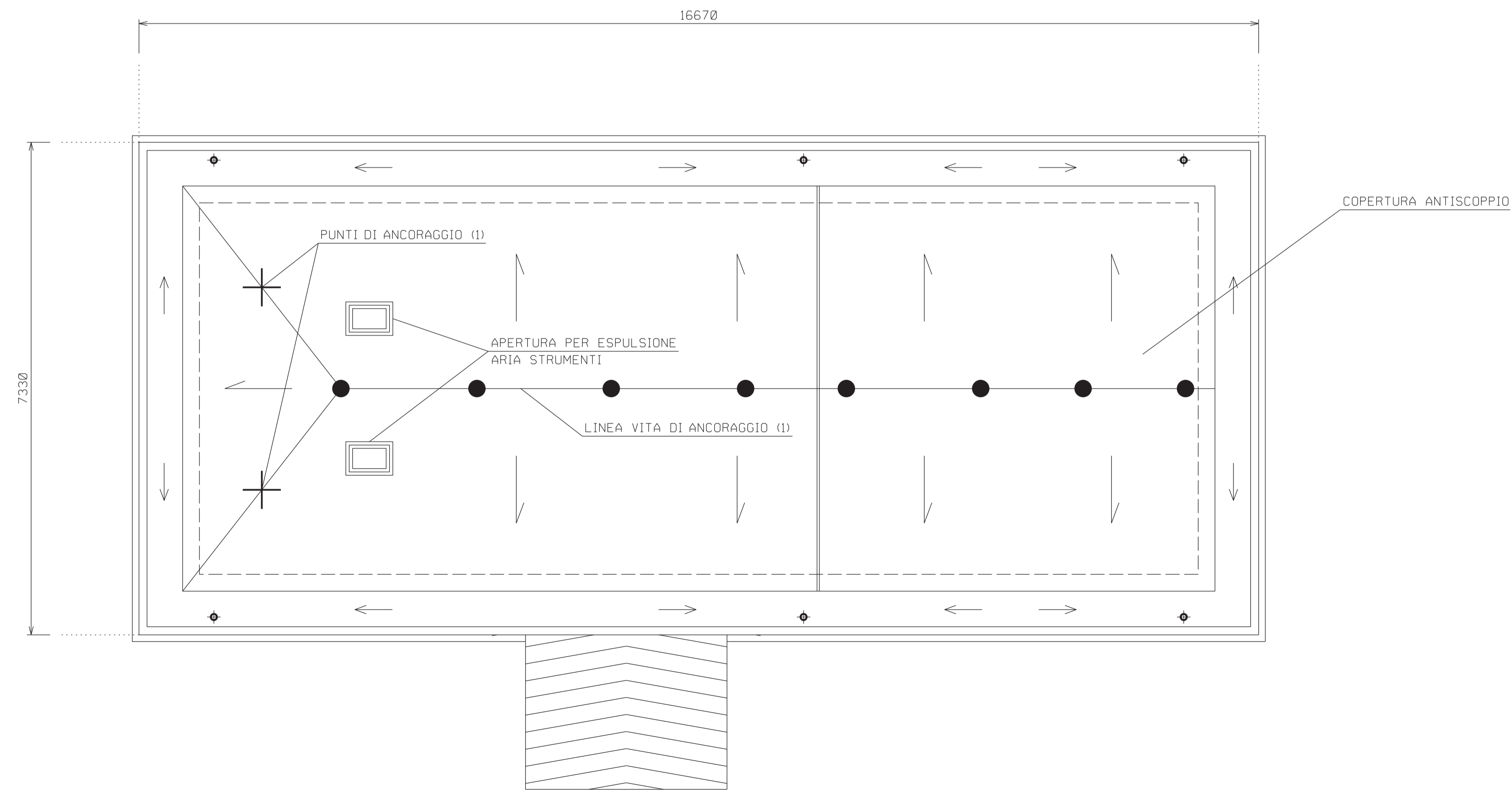
PIANTA COPERTURA
