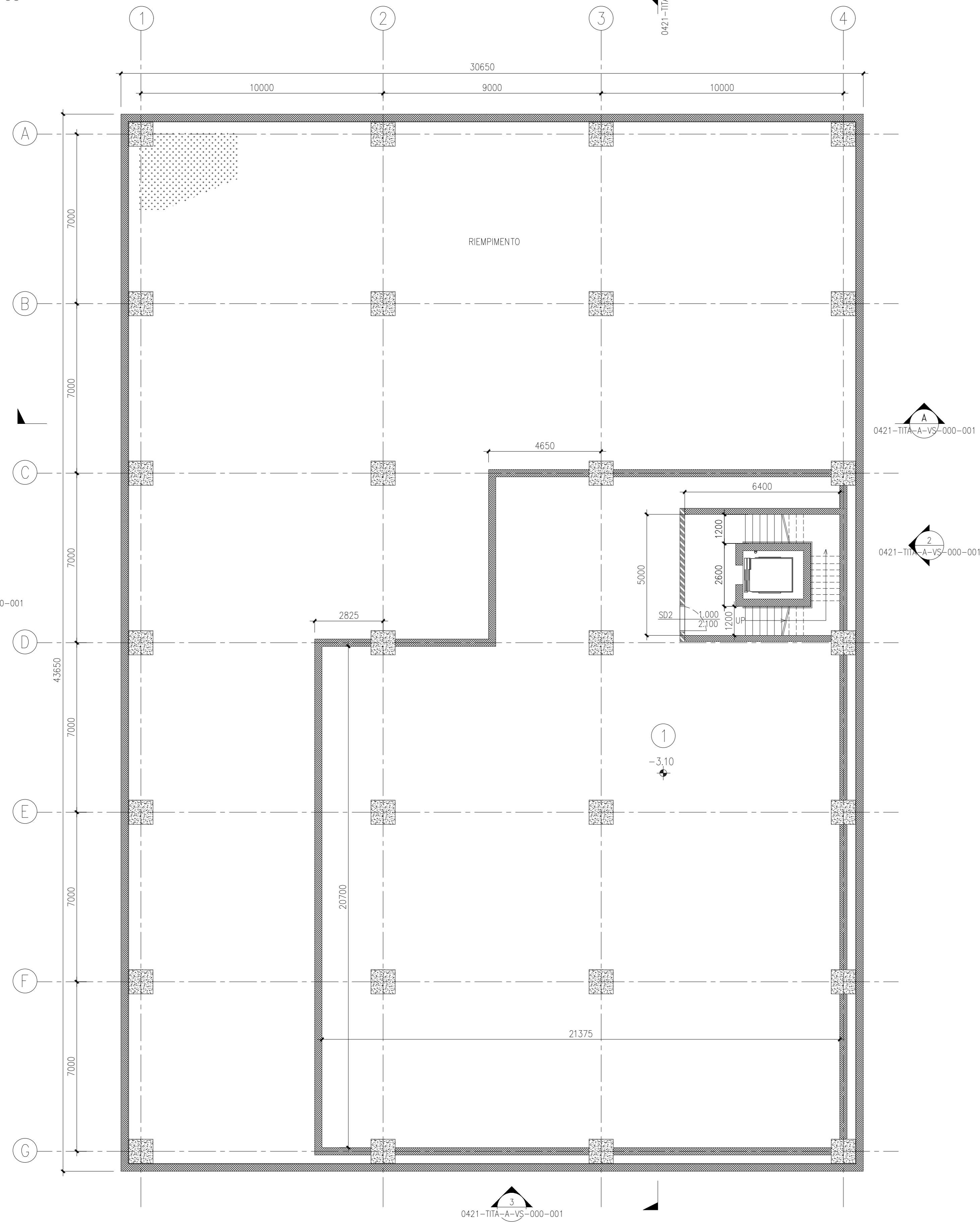
PIANTA A QUOTA -3.10M SCALA 1:100
