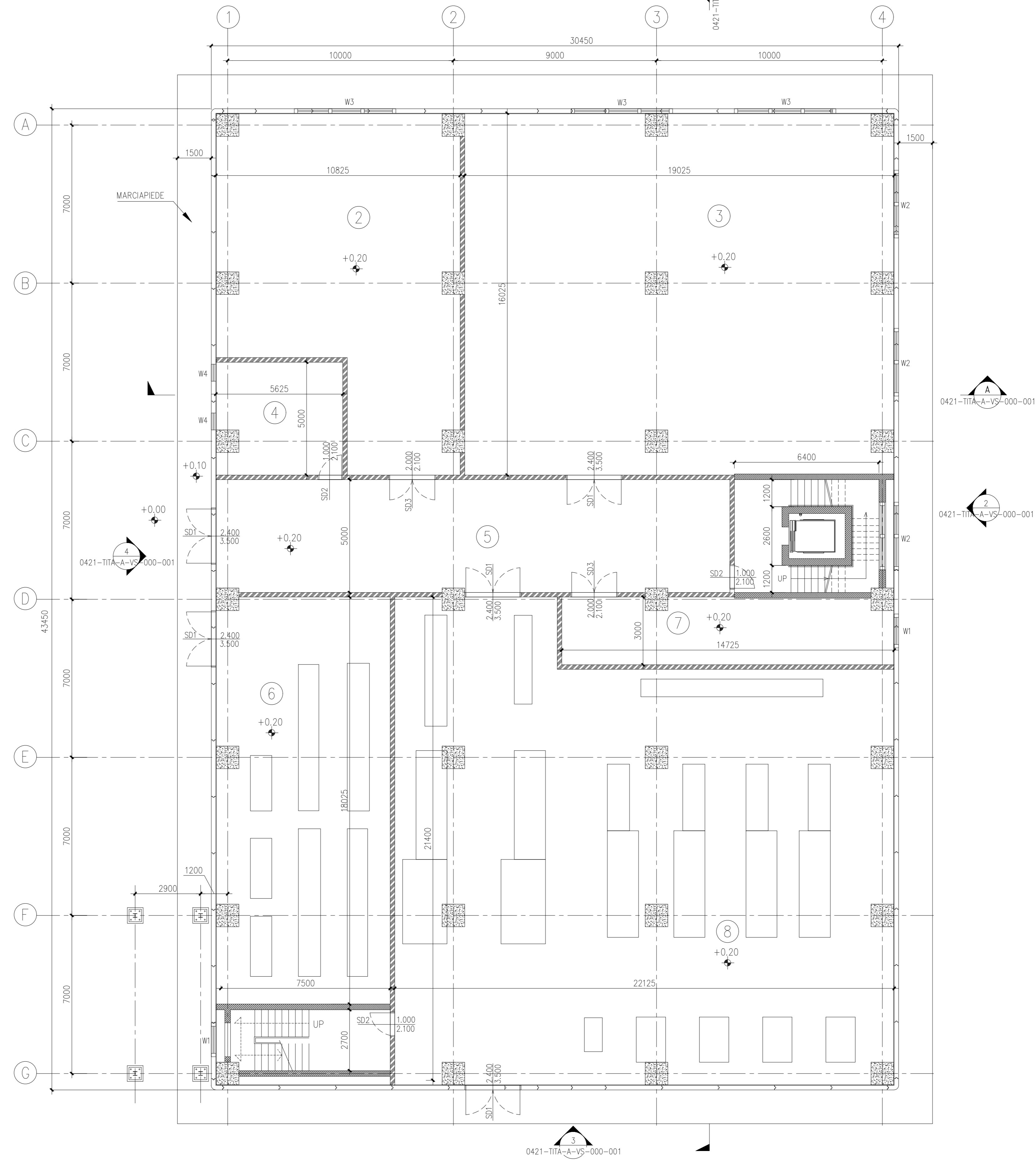
PIANTA A QUOTA +0.20M SCALA 1:100
