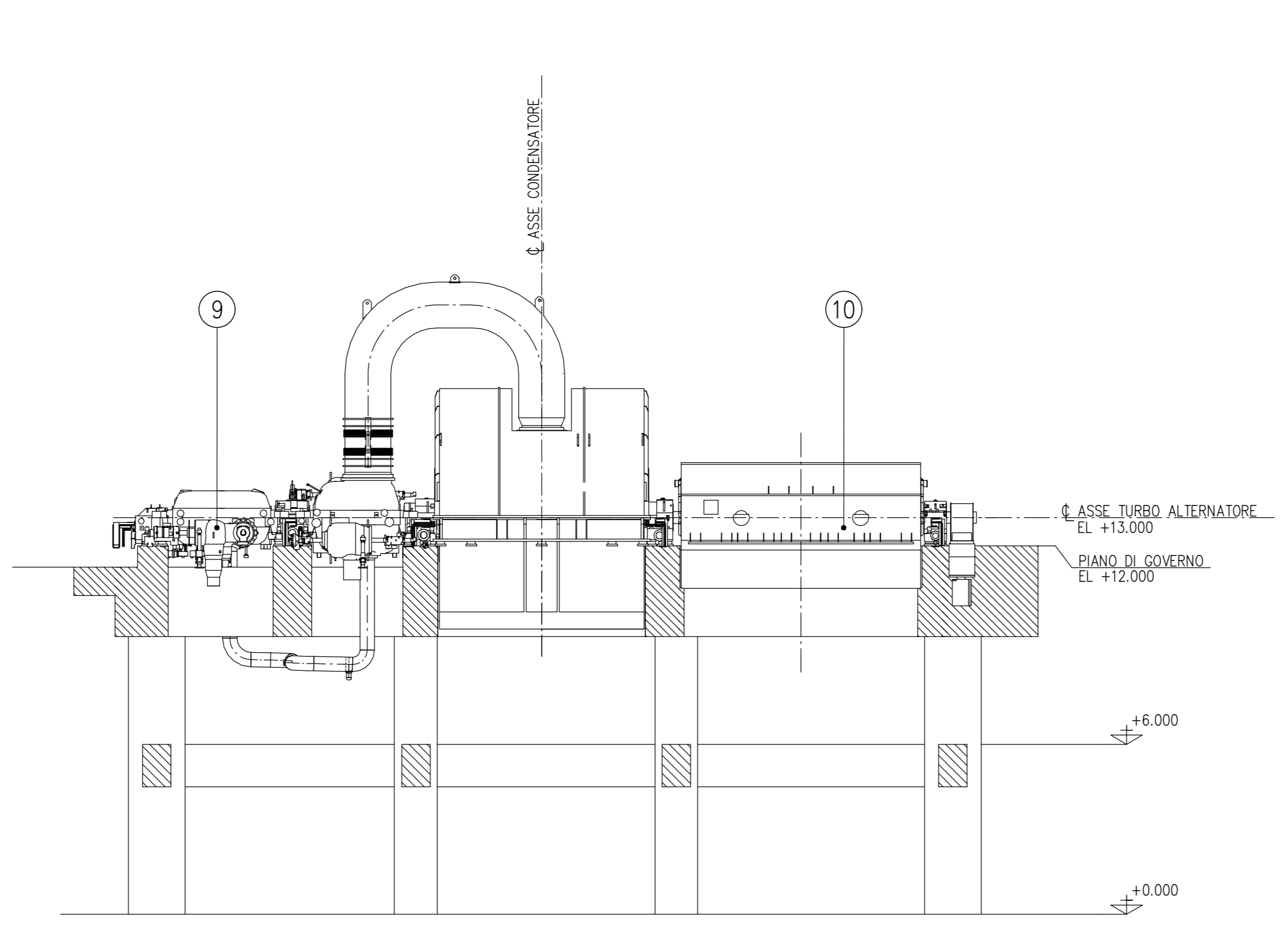
SEZIONE LATERALE TURBINA VAPORE
