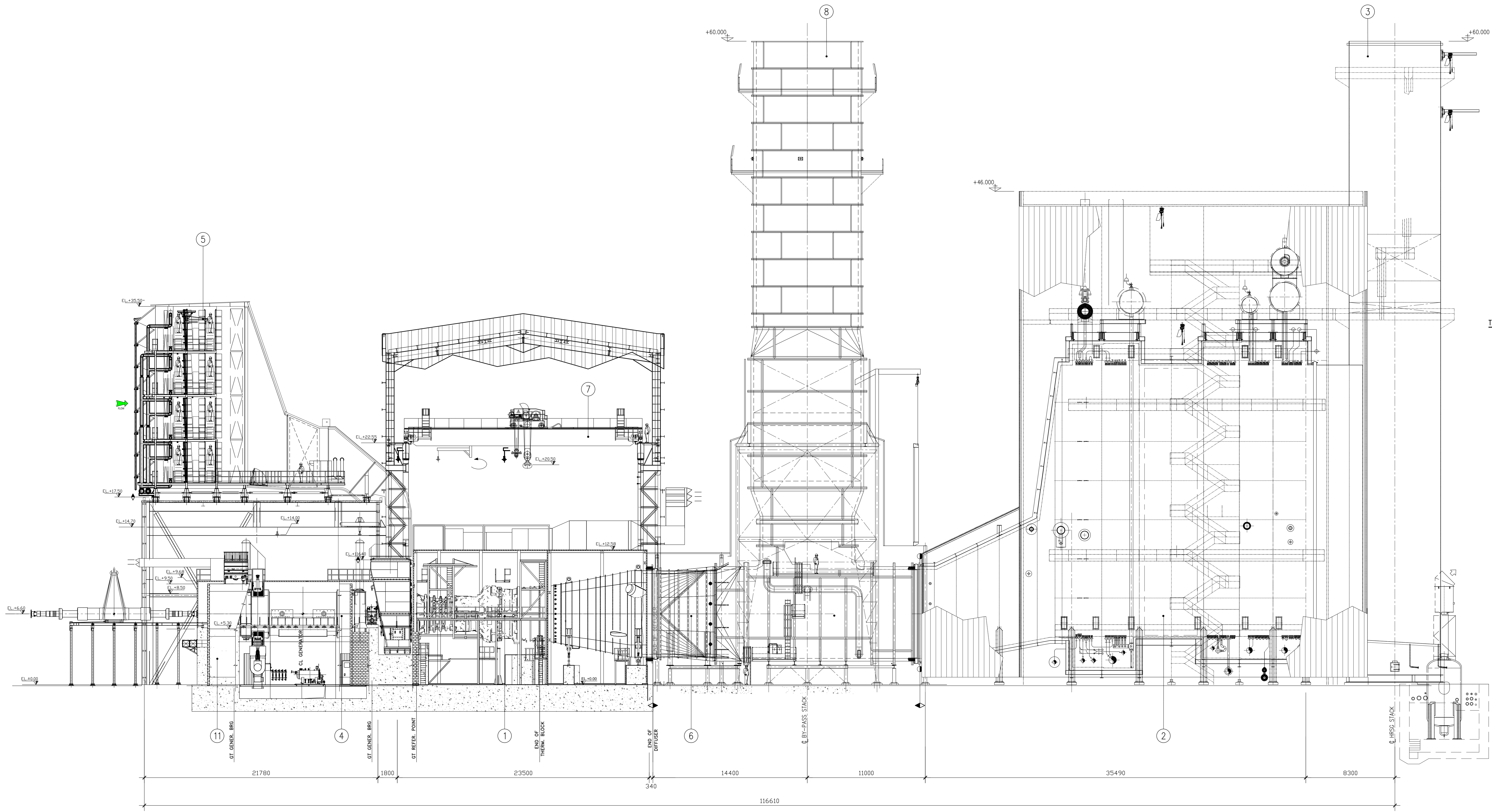
SEZIONE LATERALE TURBINA GAS E CALDAIA A RECUPERO
