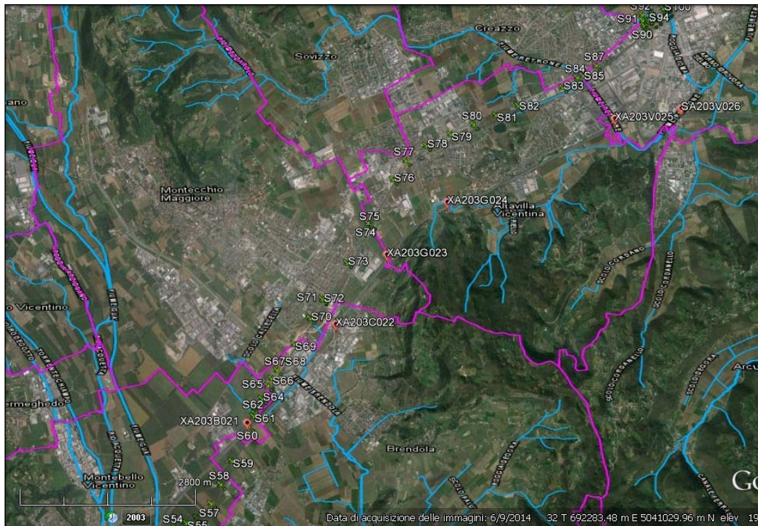
Figura 32a - Sondaggi geognostici eseguiti lungo la tratta km 38+500 e 44+250.
