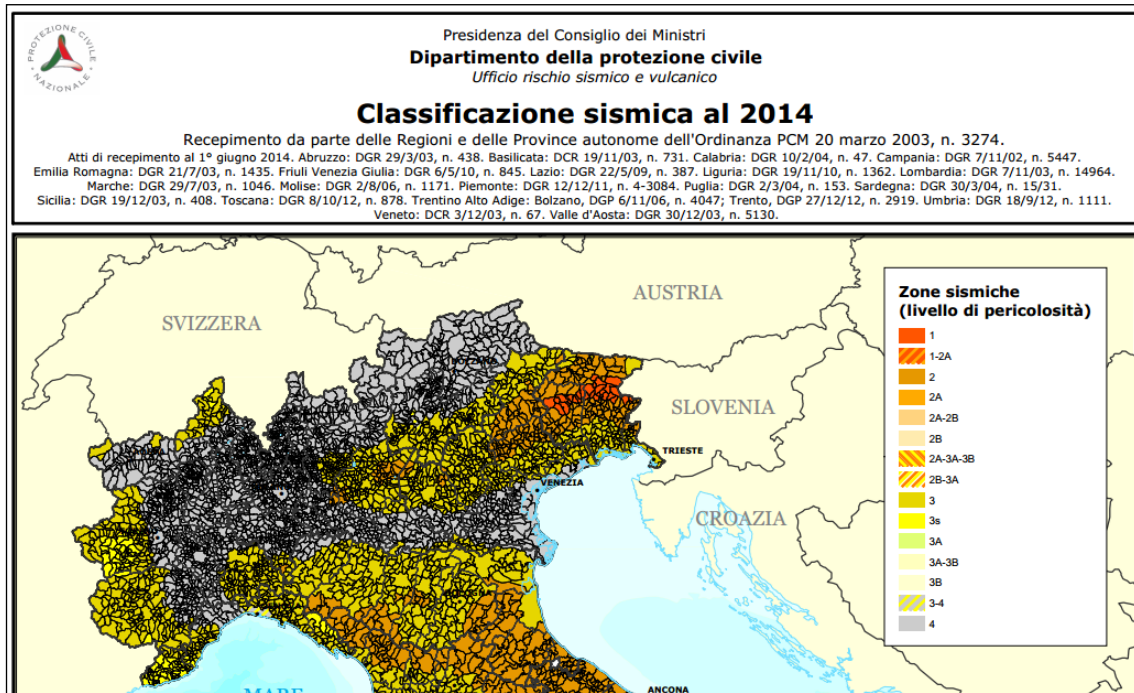
Figura 24 – Mappa di classificazione sismica 2014 – dettaglio Regione Veneto
