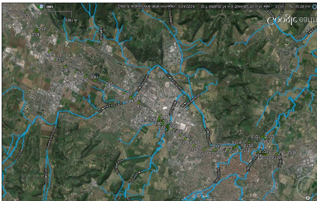
Figura 4 - Idrografia principale e secondaria nel bacino idrografico del Retrone-.
