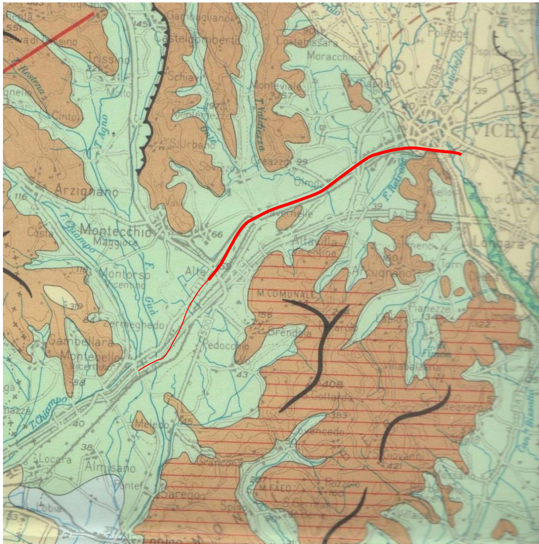
Figura 34 - Carta delle Unità Geomorfologiche (Da Regione Veneto).
