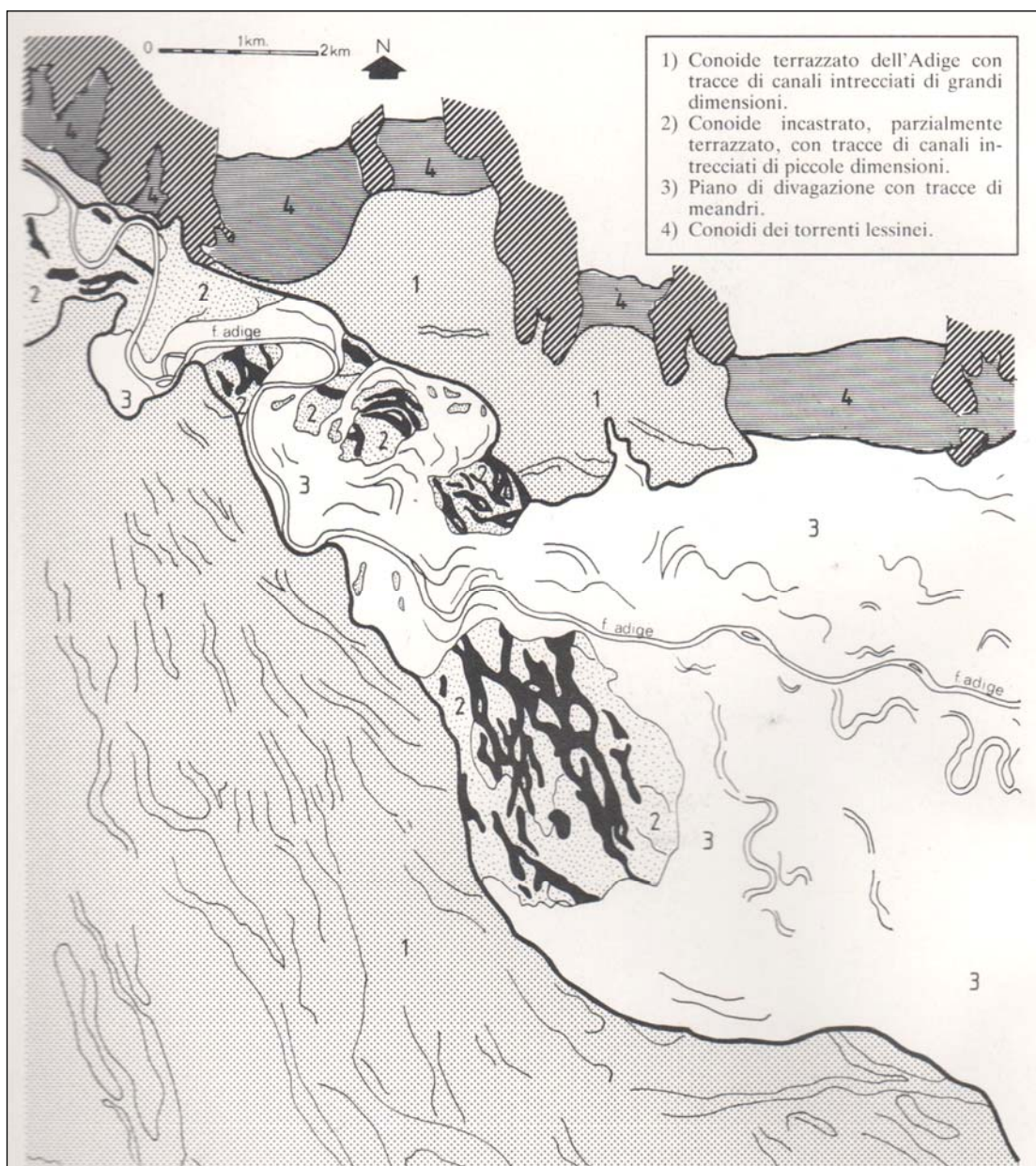
Figura 21 – Schema geomorfologico della porzione di pianura a SE di Verona da L. Sorbini & Alti (1984) [45].
