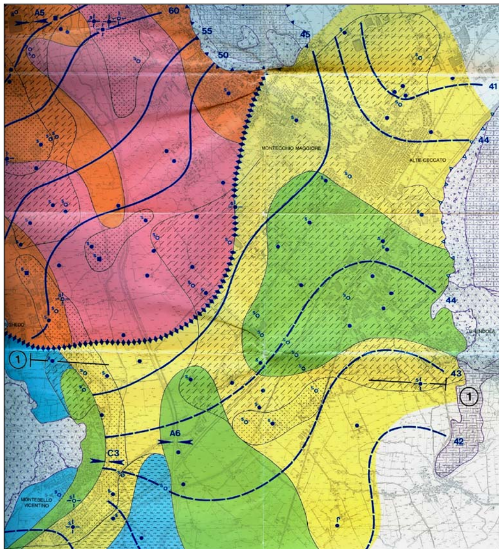
Figura 10 - Stralcio della carta della vulnerabilità naturale (Regione Veneto).
