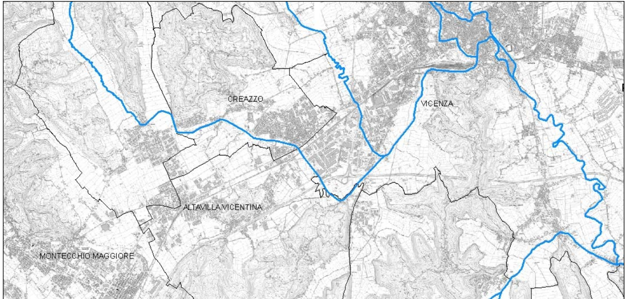
Figura 33 - Inquadramento territoriale Il tratta km 38+500 +44+250.
