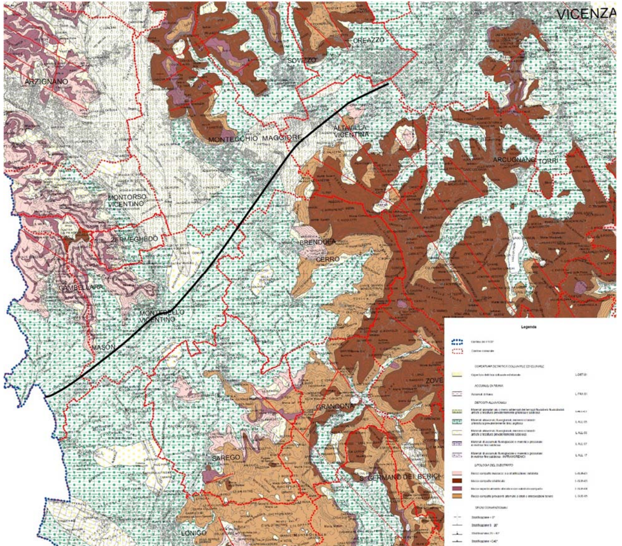
Figura 17 - Stralcio della Carta geolitologica (PTCP Provincia di Vicenza).
