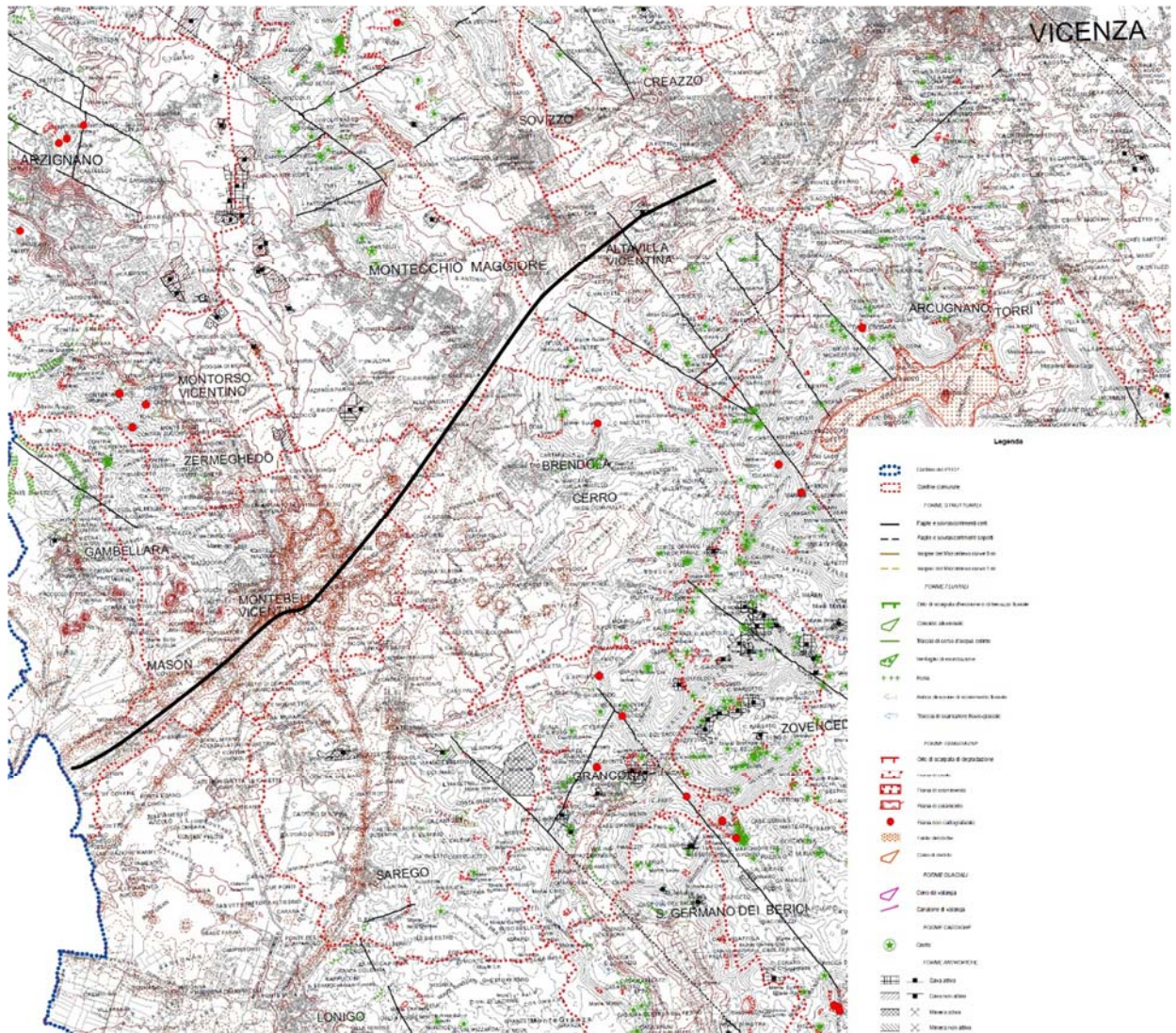
Figura 19 - Stralcio della Carta geomorfologica (PTCP Provincia di Vicenza).
