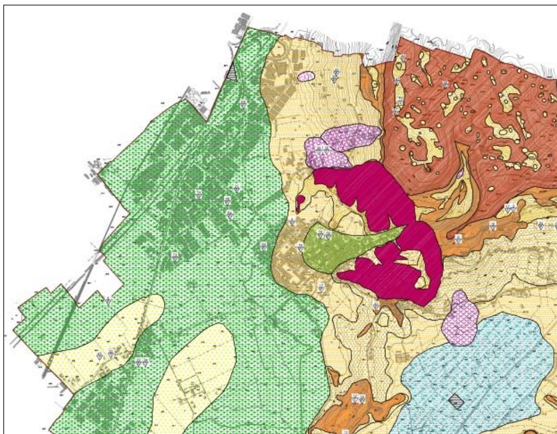
Figura 12 - Stralcio della Carta litologica del Comune di Brendola in scala 1:10.000 (Da: PAT, 2012).
