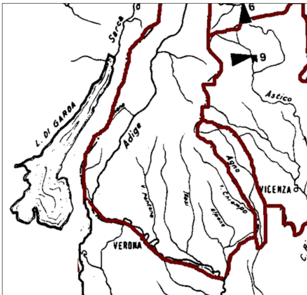
Figura 2 - Delimitazione del bacino idrografico e asta dei principali corsi d'acqua interferenti con l'opera in progetto
