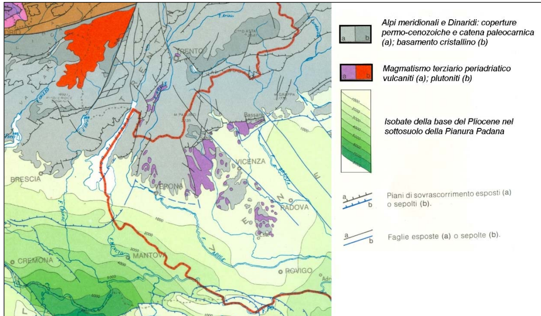
Figura 9 - Schema strutturale (Da carta Geologica del Veneto).
