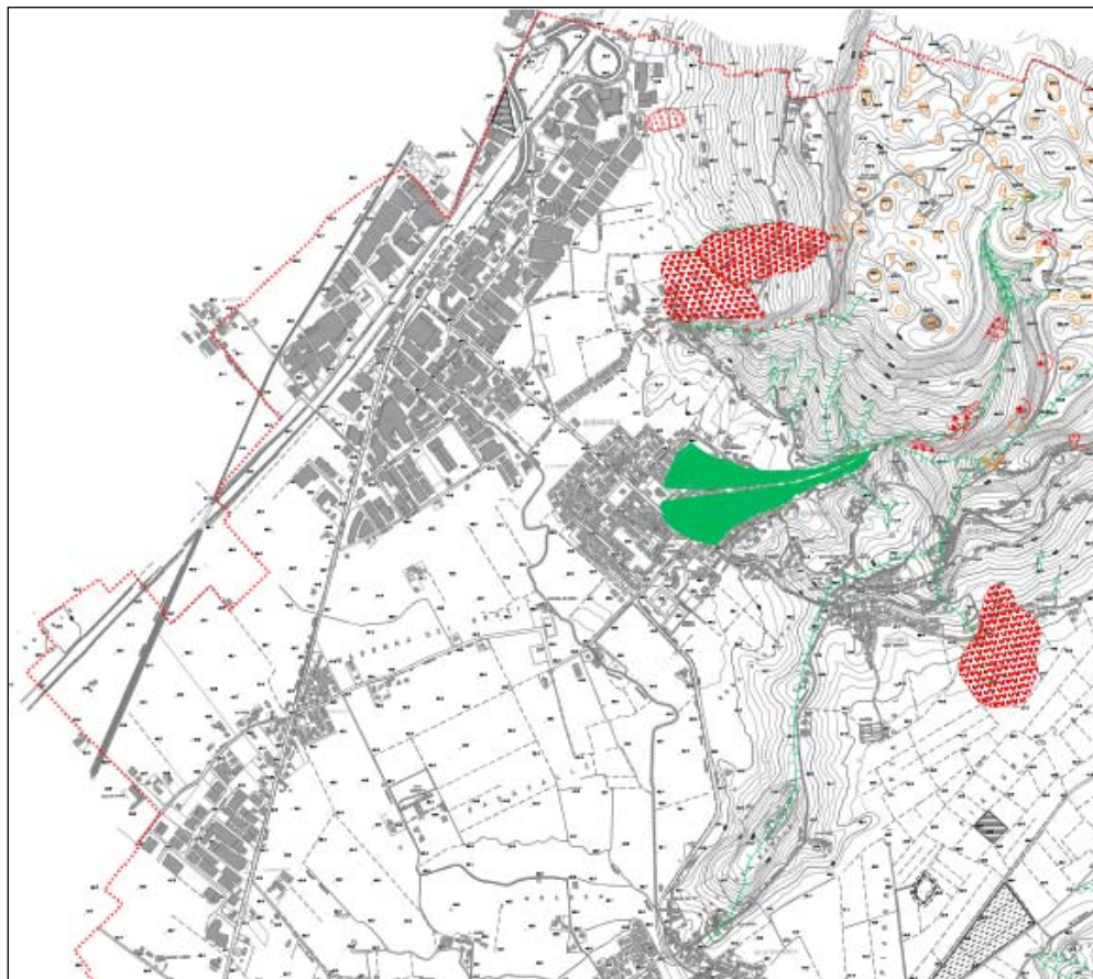
Figura 14 - Stralcio della Carta geomorfologica del Comune di Brendola in scala 1:10.000 (Da: PAT, 2012).
