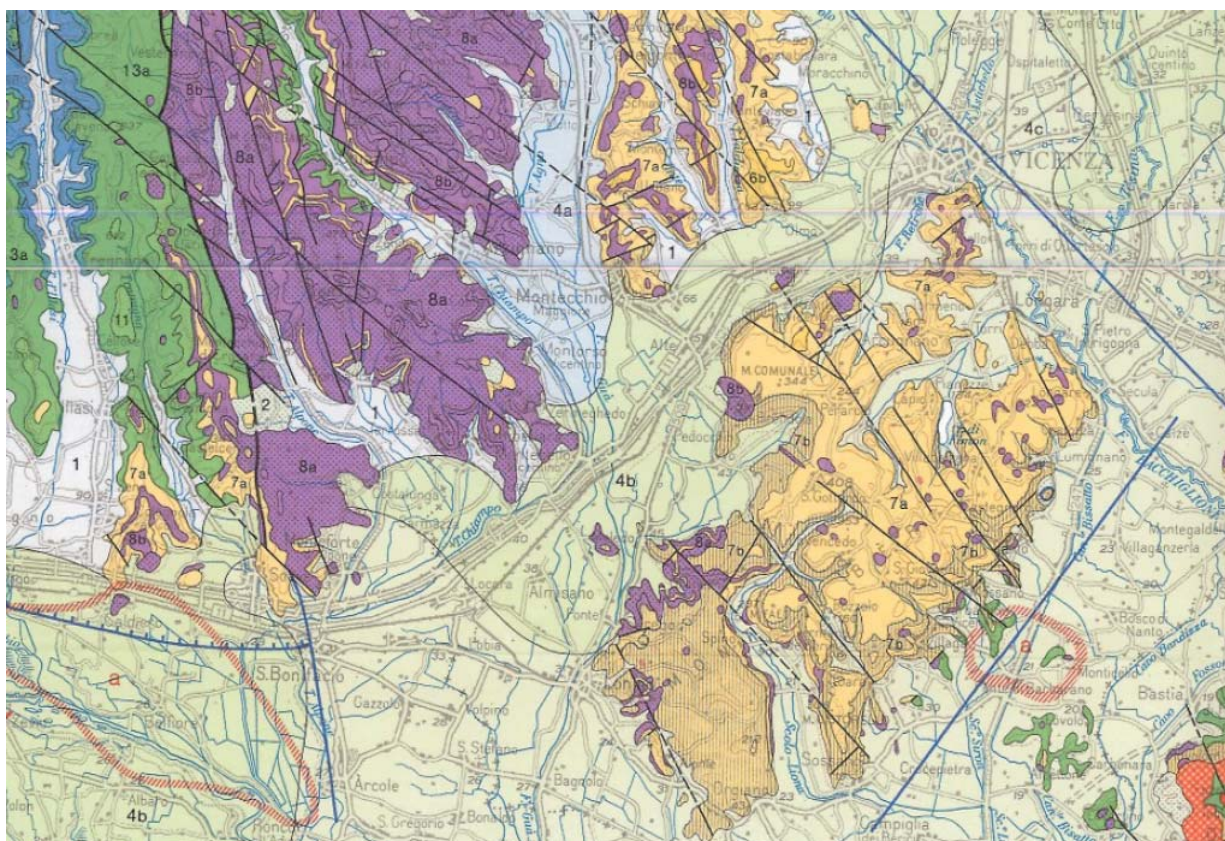
Figura 8 - Stralcio della Carta Geologica del Veneto in scala 1:250.000.
