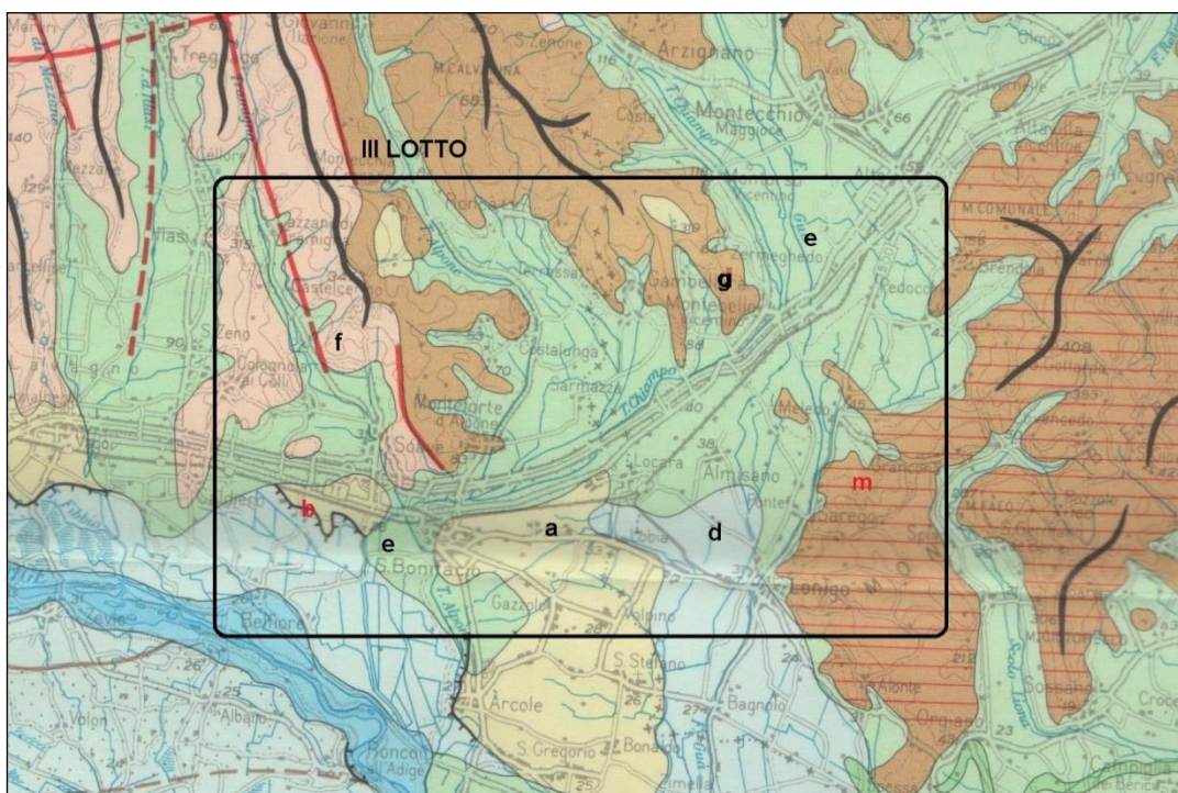
Figura 27 - Carta delle Unità Geomorfologiche (Da Regione Veneto).
