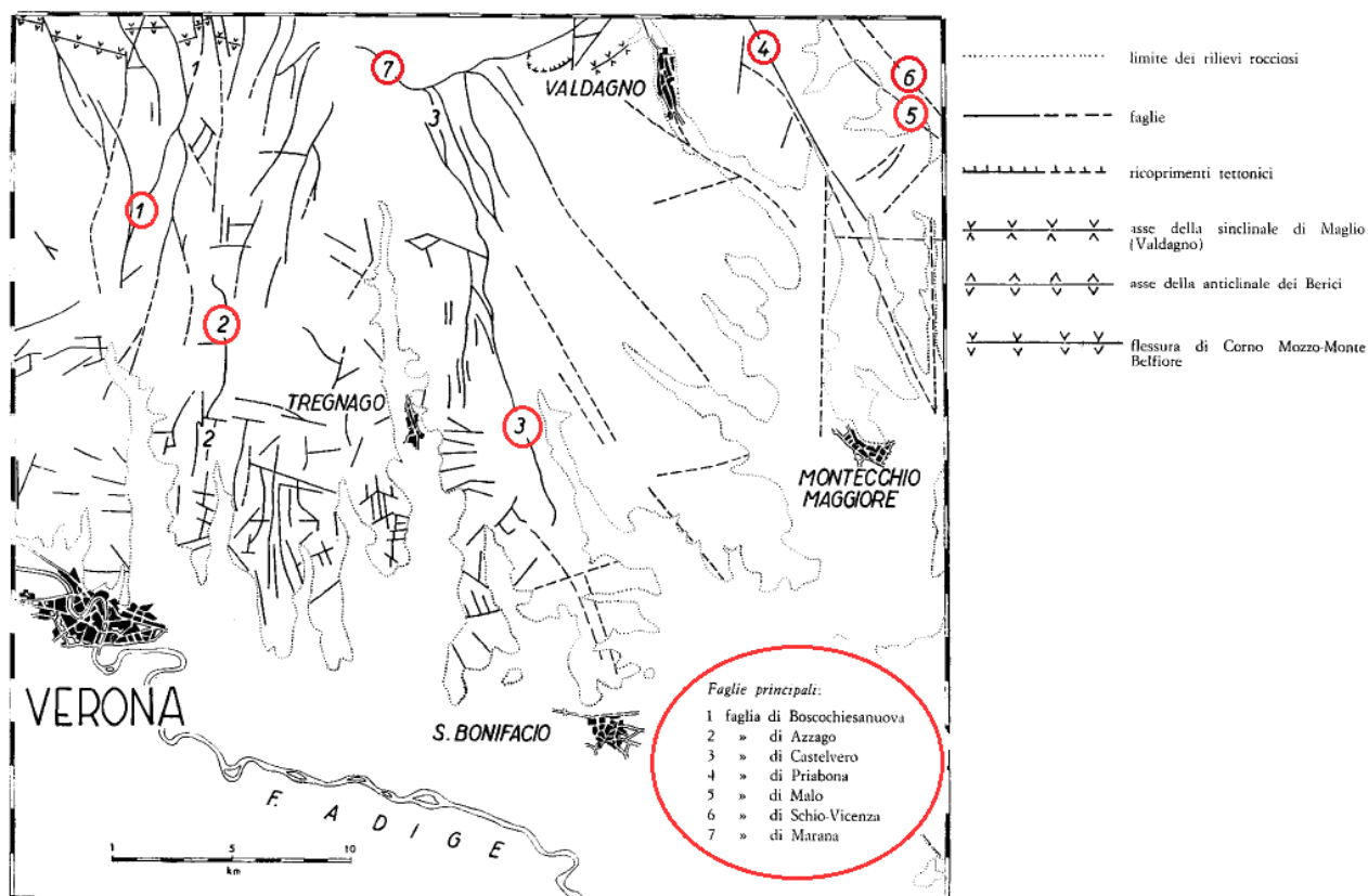
Figura 20 - Schema tettonico dei Monti Lessini e Berici.
