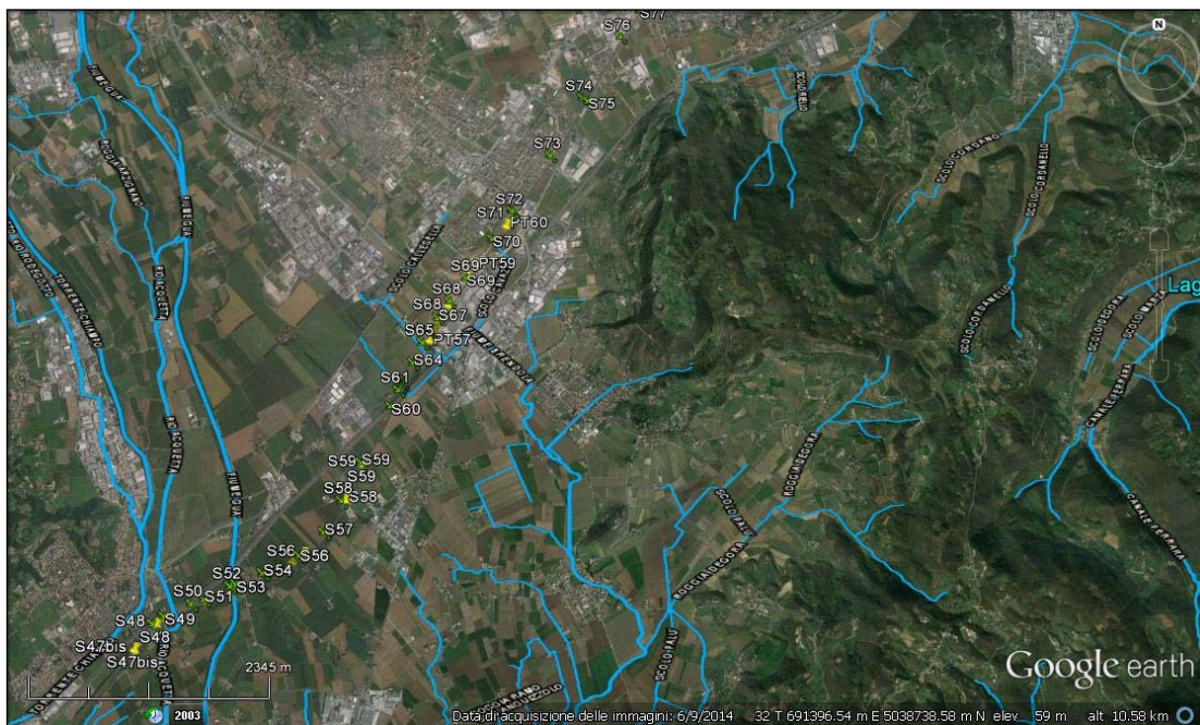
Figura 3 - Idrografia principale e secondaria nel bacino idrografico Agno-Guà.
