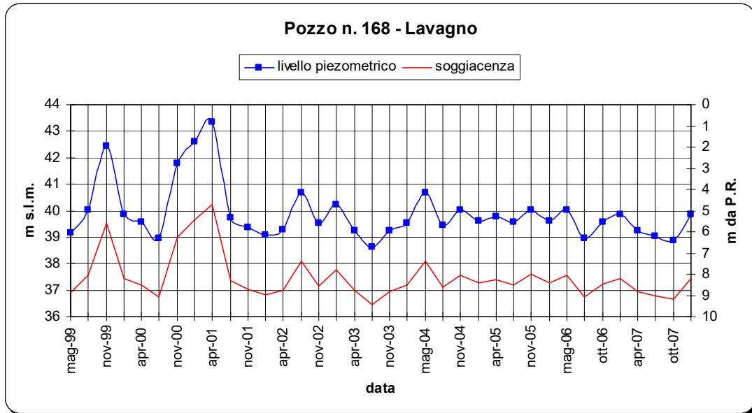
Figura 22 - Oscillazione freatica nel pozzo n.168 di Lavagno (1999-2007).
