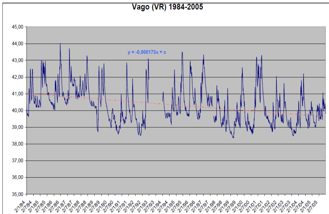
Figura 23 - Oscillazione freatica nel pozzo n. 56 di Vago (1984-2005).
