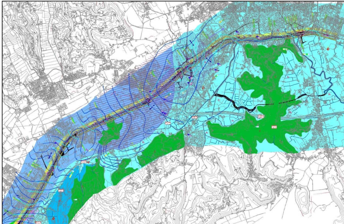
Figura 41 - Superficie piezometrica della falda nel tratto Montecchio M – Vicenza.
