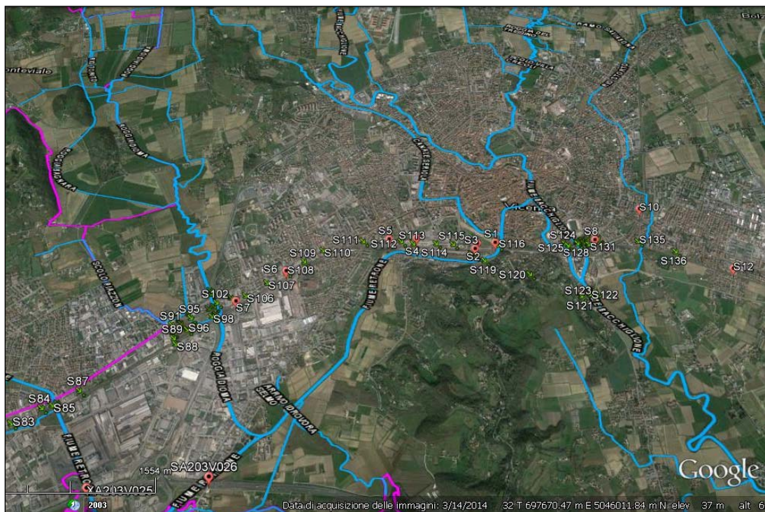
Figura 38b - Sondaggi geognostici eseguiti lungo la tratta km 38+500 e 44+250
