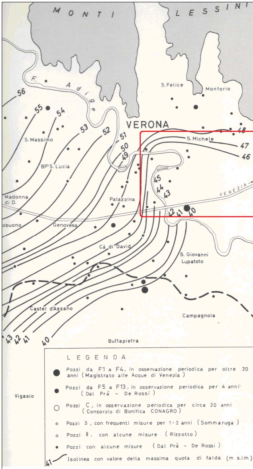
Figura 18 - Carta isopiezometrica di massima quota della falda (Dal Prà, De Rossi, 1991).
