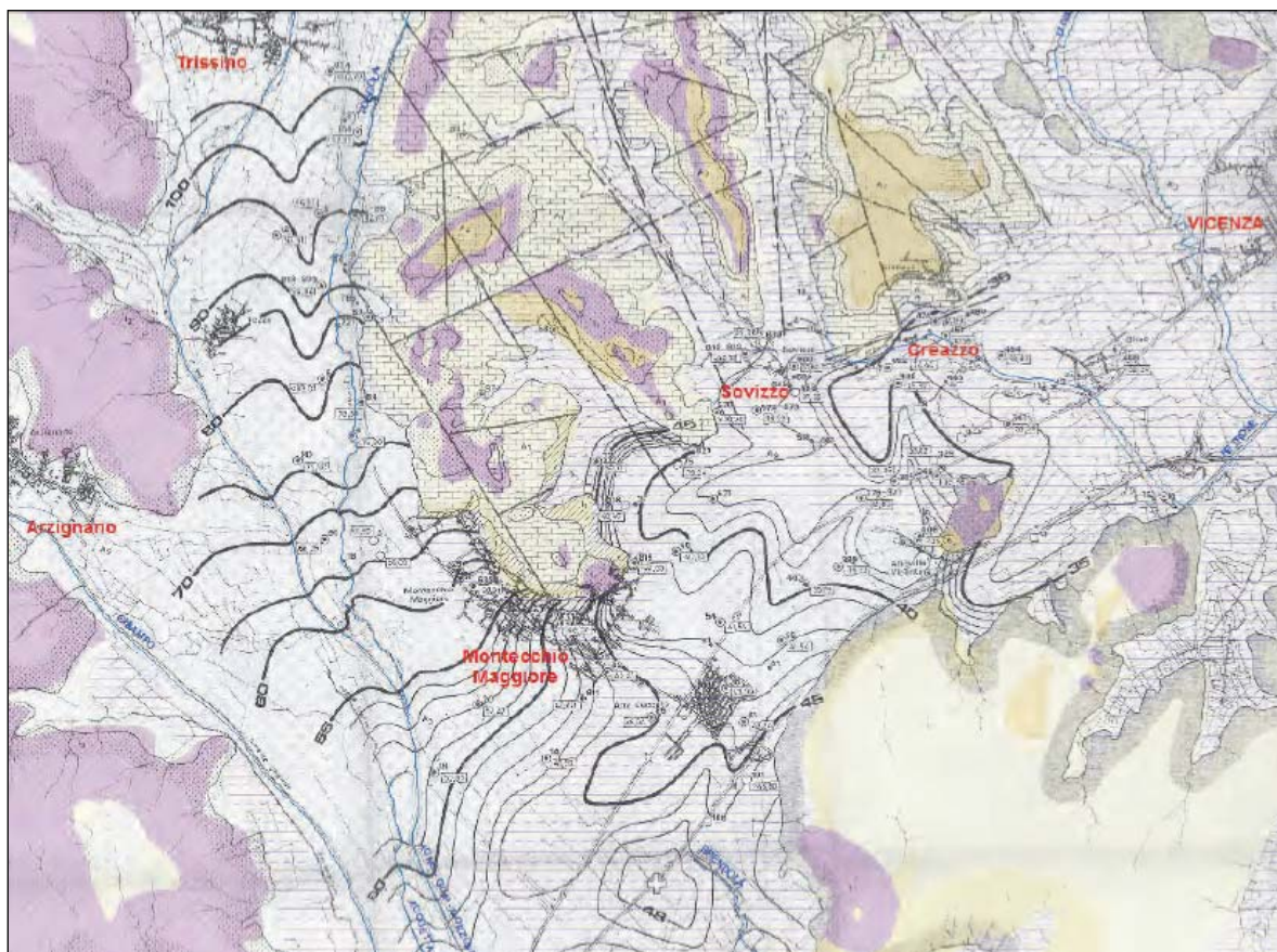
Figura 10 - Isofreatiche nella media-bassa valle dell'Agno nel settembre 1978 (Da studio IRSEV "Studio Geologico e chimico dell'inquinamento della falda acquifera nei comuni di Montecchio M., Creazzo, Sovizzo e Altavilla V.").
