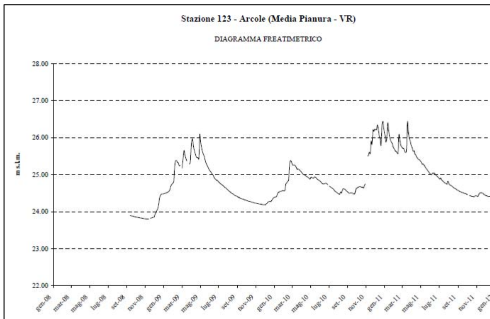
Figura 28 - Oscillazione freatica nel pozzo n. 123 di Arcole (2009-2012).
