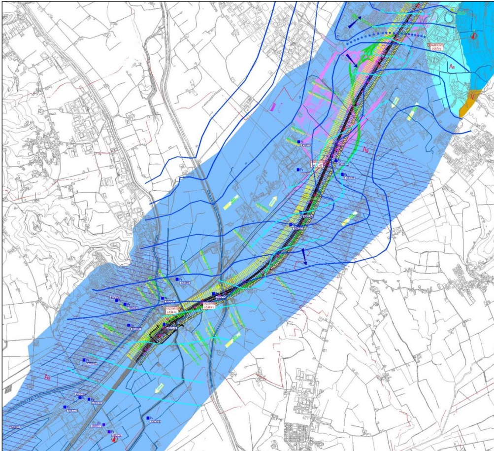
Figura 37 - Superficie piezometrica della falda nel tratto Montebello V.– Montecchio M.
