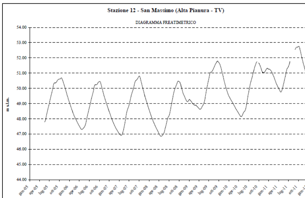
Figura 25 - Oscillazione freatica nel pozzo n. 12 San Massimo (2005-2012).
