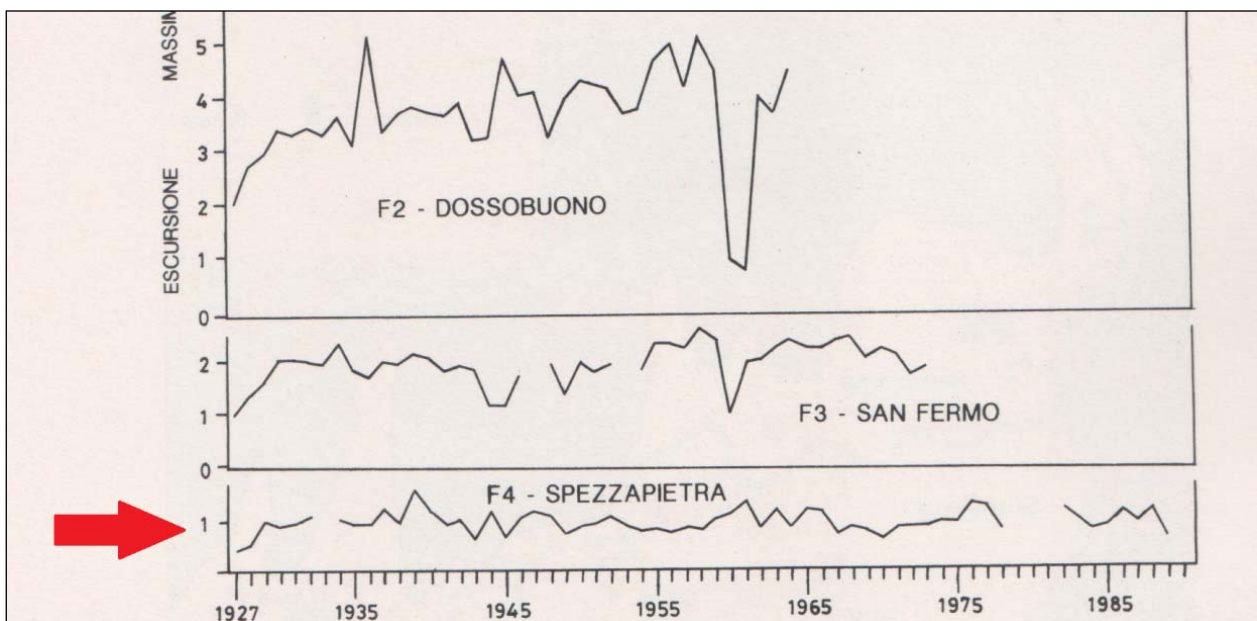
Figura 16 - Escursione massima annua della falda freatica 1926-1990.
