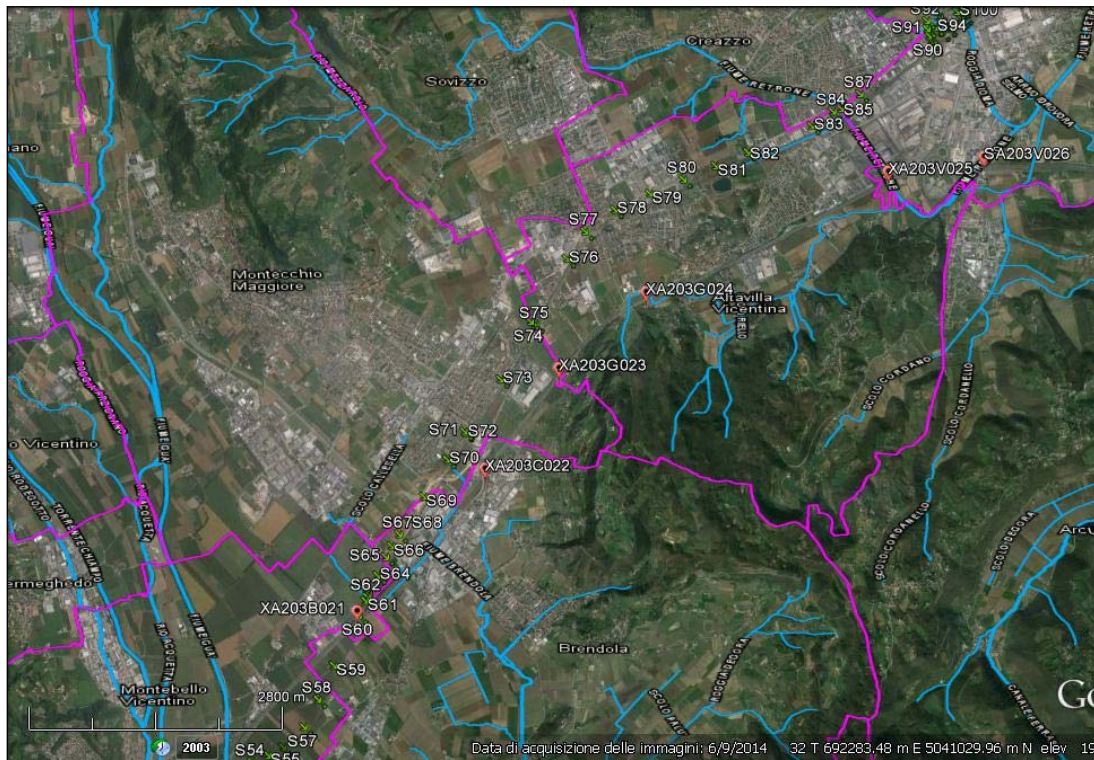
Figura 38a - Sondaggi geognostici eseguiti lungo la tratta km 38+500 e 44+250.
