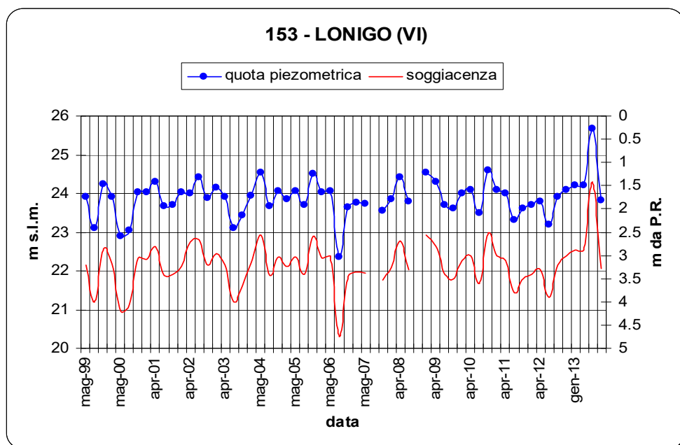
Figura 30 - Oscillazione freatica nel pozzo n. 153 di Lonigo (1999-2013).
