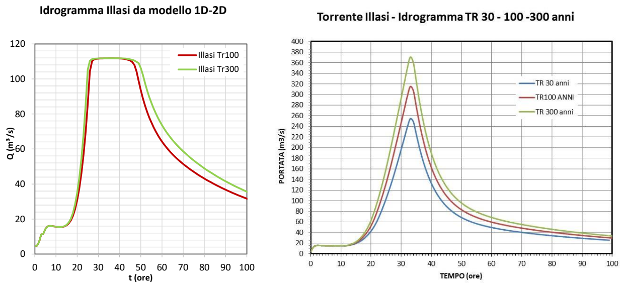
Figura 10.6 – Idrogrammi del T. Illasi: a sinistra quelli calcolati con il modello idraulico 1D-2D a destra quelli idrologici.
