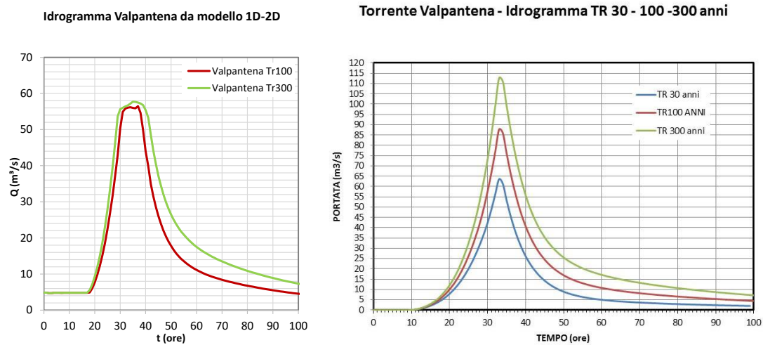
Figura 10.4 – Idrogrammi del T. Valpantena: a sinistra quelli calcolati con il modello idraulico 1D-2D a destra quelli idrologici
