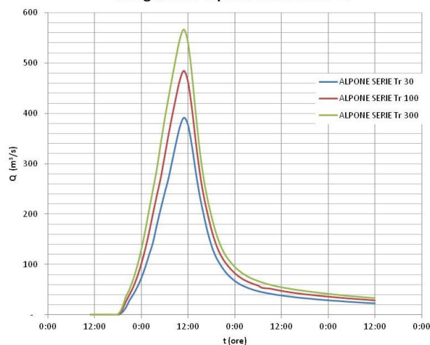
Figura 10.8 – Idrogrammi del T. Alpone: a sinistra quelli calcolati con il modello idraulico 1D-2D a destra quelli idrologici.
