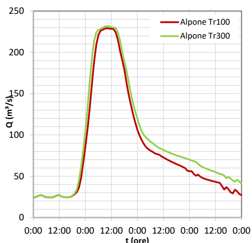
Figura 10.8 – Idrogrammi del T. Alpone: a sinistra quelli calcolati con il modello idraulico 1D-2D a destra quelli idrologici.
