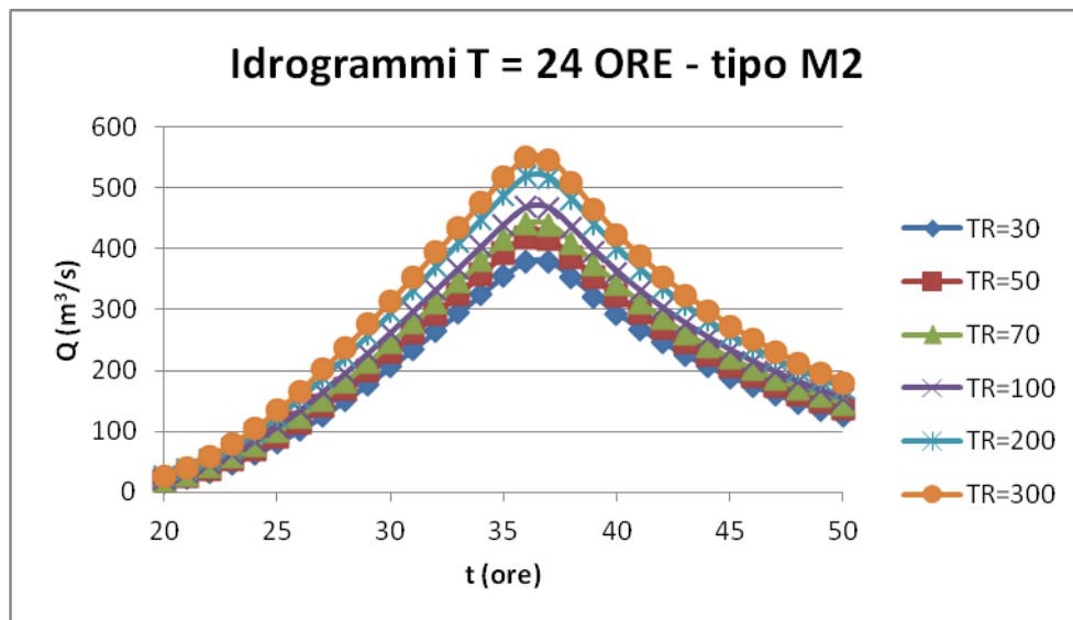
Figura 10.9 - Idrogrammi del fiume Guà
