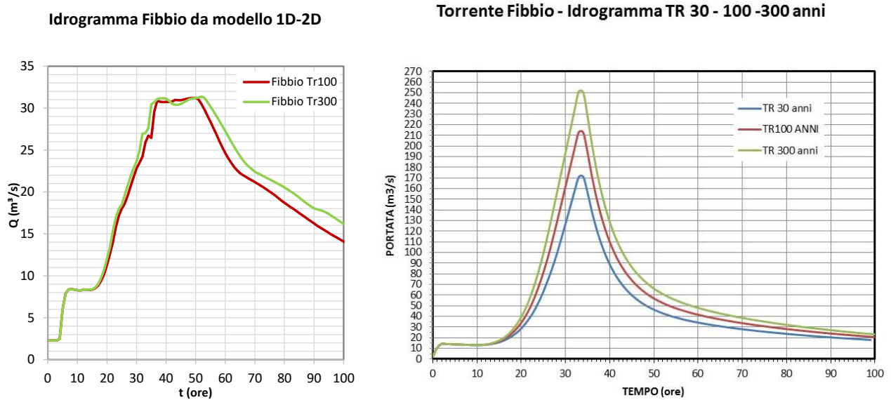
Figura 10.5 – Idrogrammi del T. Fibbio: a sinistra quelli calcolati con il modello idraulico 1D-2D a destra quelli idrologici.
