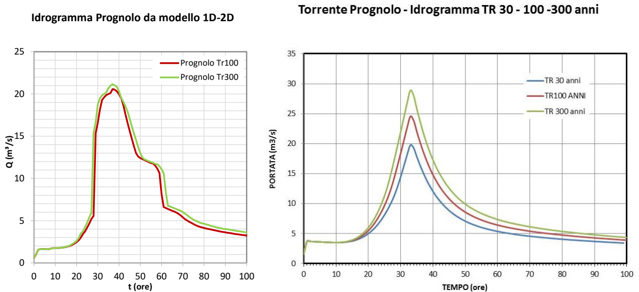
Figura 10.7 – Idrogrammi del T. Prognolo: a sinistra quelli calcolati con il modello idraulico 1D-2D a destra quelli idrologici.
