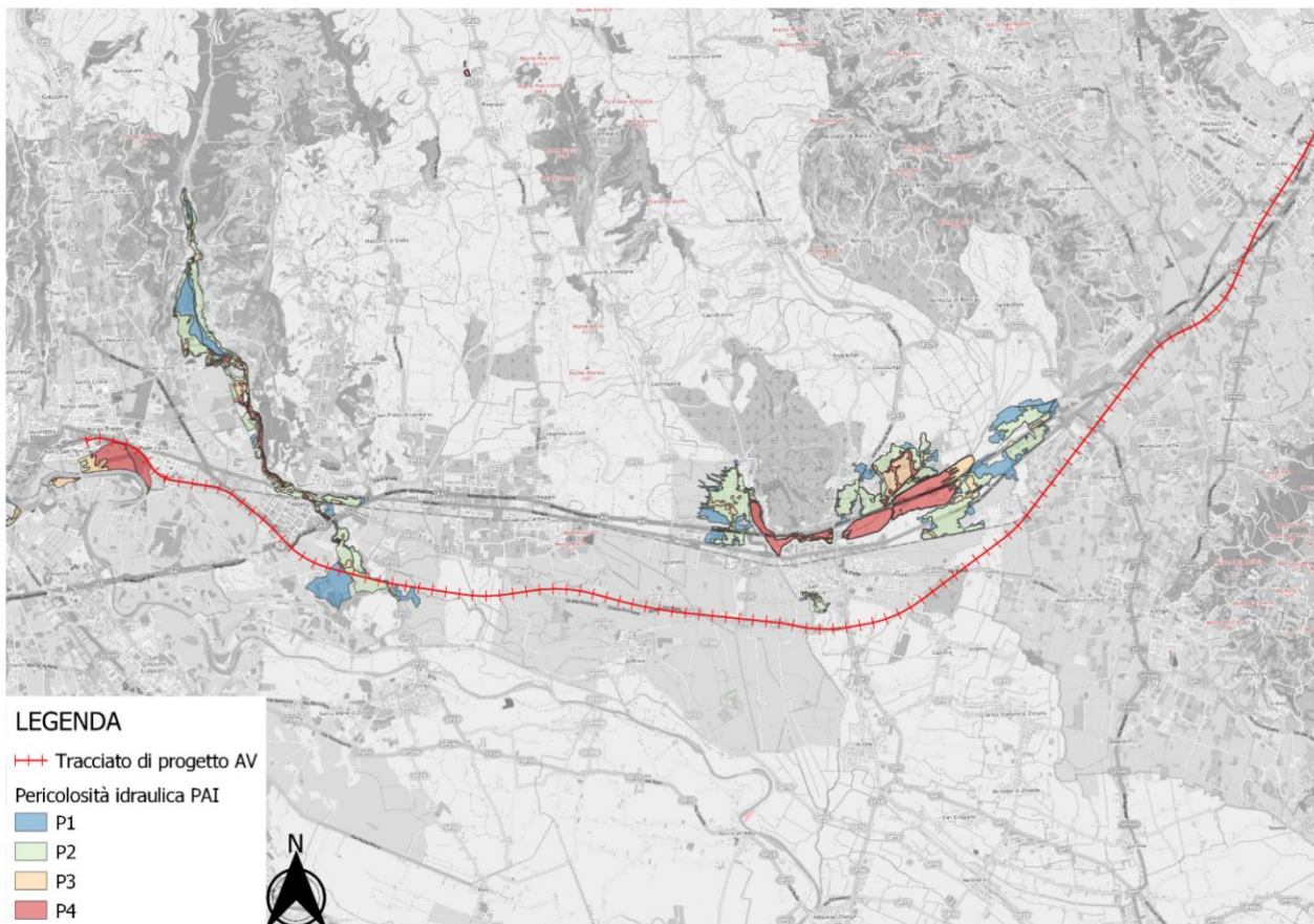
Figura 5.8 Pericolosità PAI bacino Adige nella zona di interesse del progetto AV
