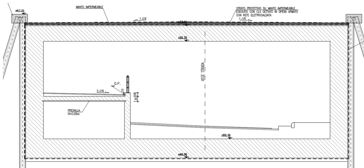
Figura 1.3: Sezione trasversale
