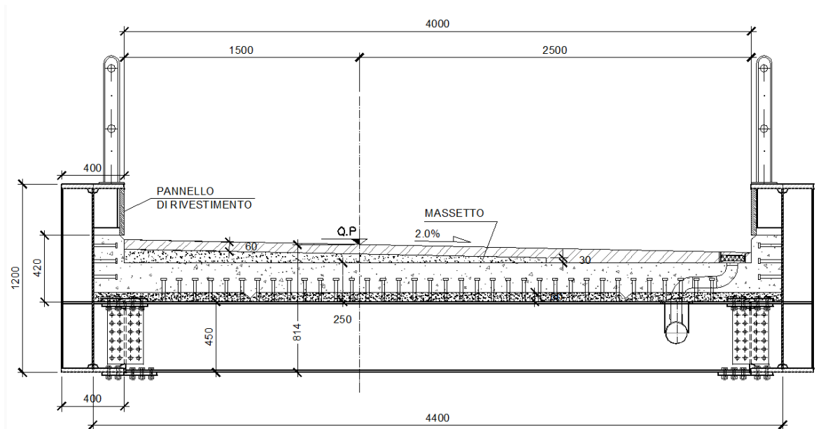
Figura 2: sezione trasversale ponte ciclopedonale
