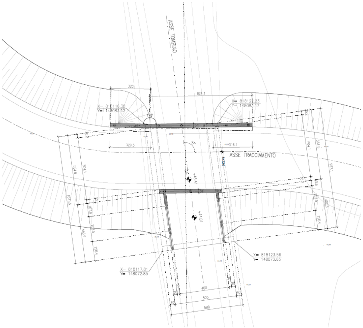
Figura 4: planimetria di progetto
