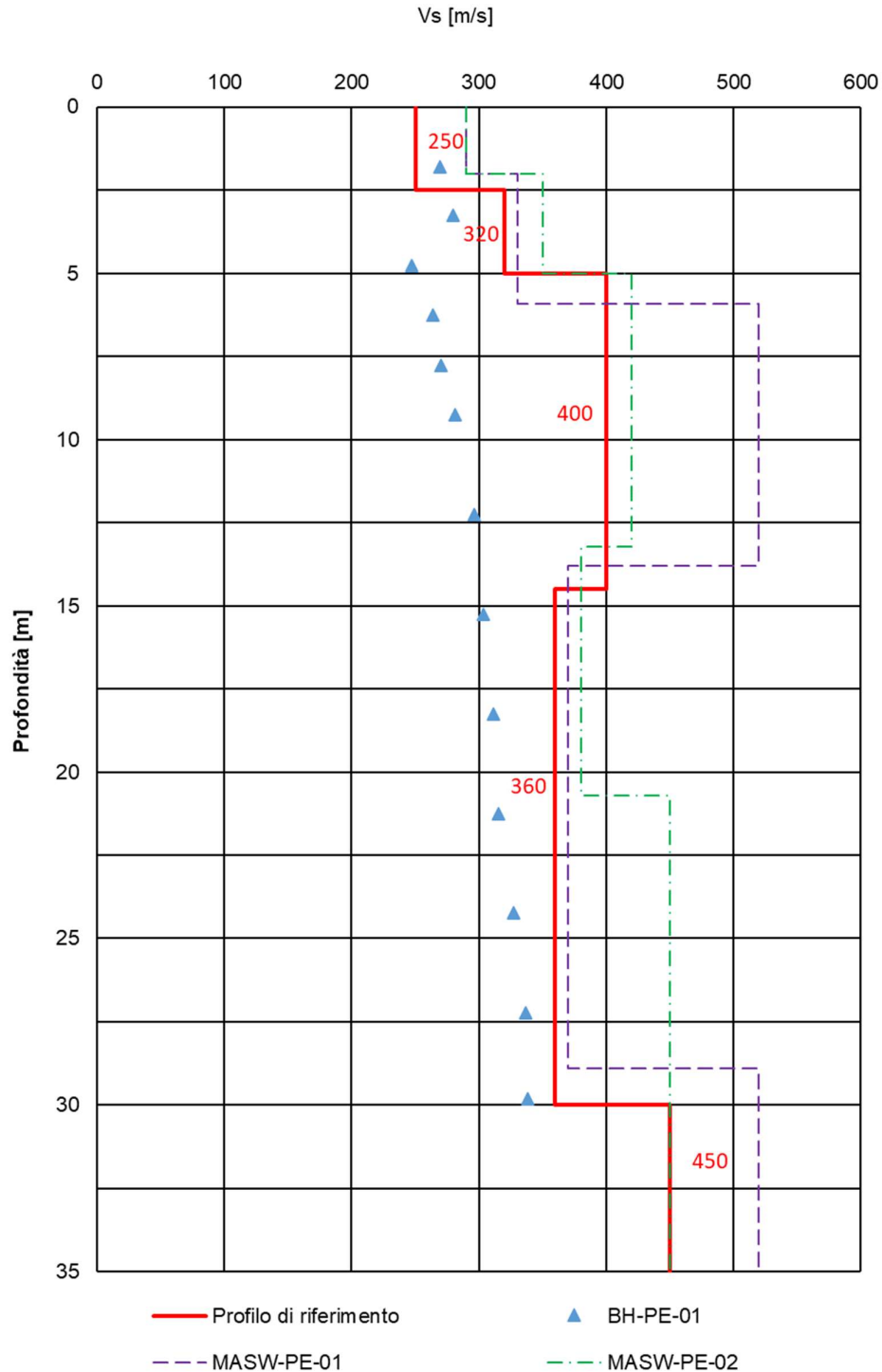
Figura 8 – Profilo di Vs di riferimento, a confronto con dati di correlazioni con SPT e prove geofisiche tipo MASW, tra pk 0+125 a pk 0+174
