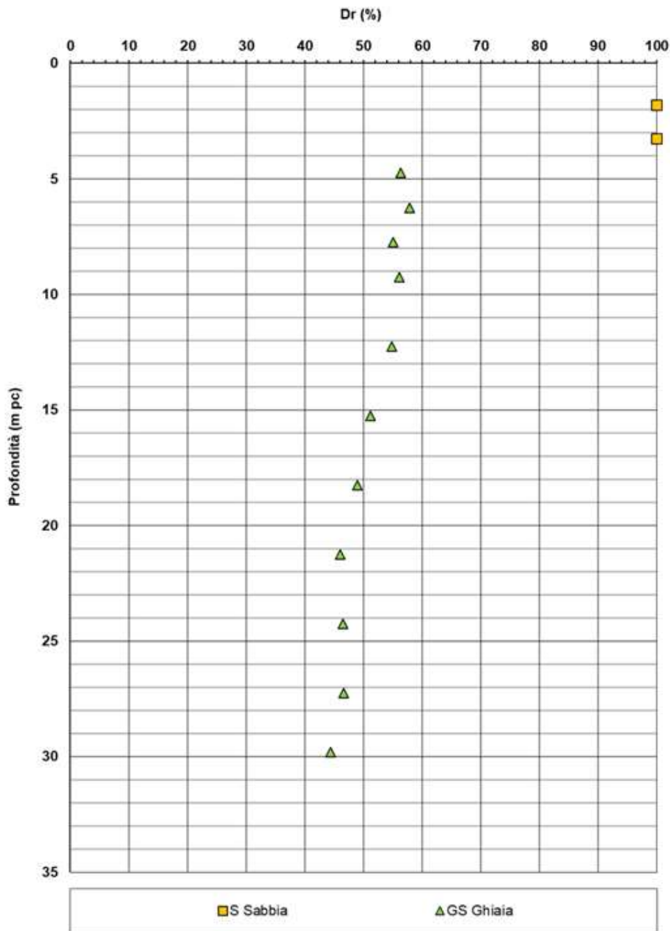
Figura 6 – Densità relativa da prove SPT tra pk 0+125 a pk 0+174
