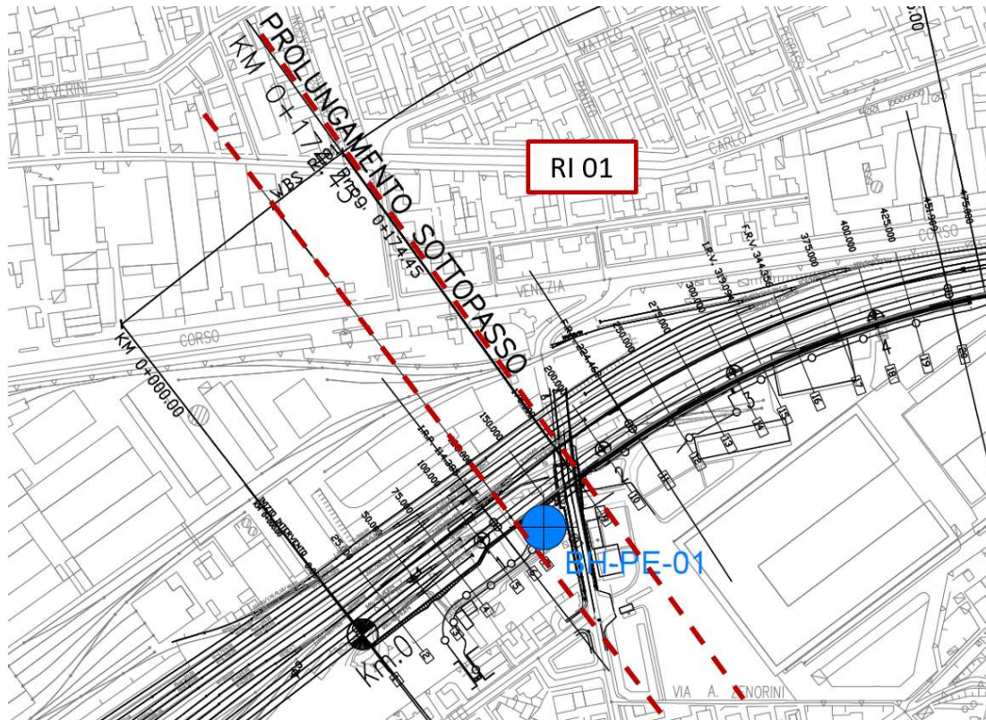
Figura 3 - Planimetria Rilevato RI01, estratto dalla Planimetria Generale (Doc. Rif. [3])
