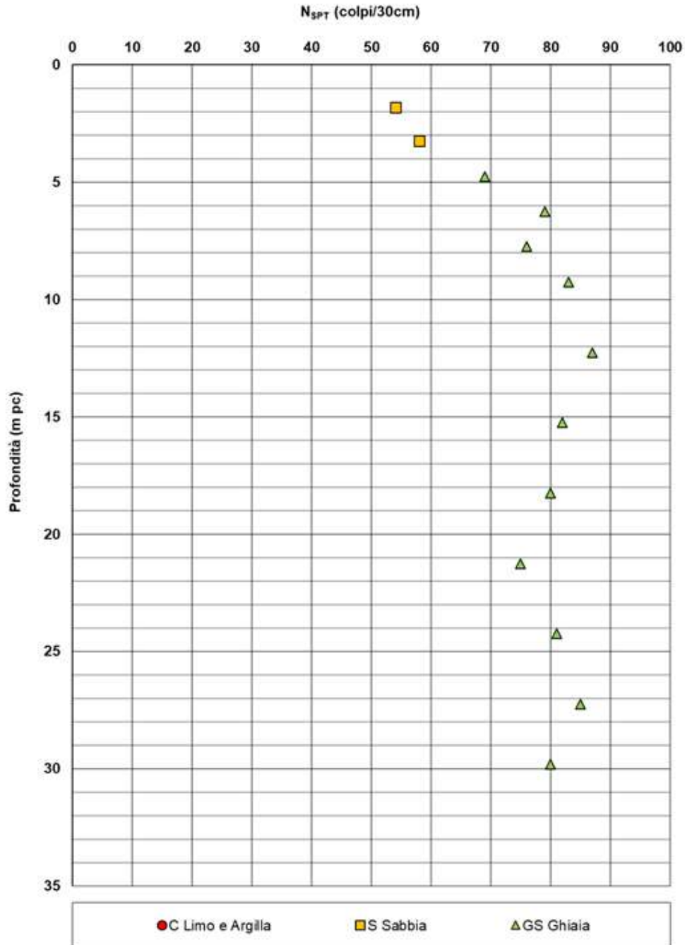
Figura 5 – Esito delle prove SPT tra pk 0+125 a pk 0+174
