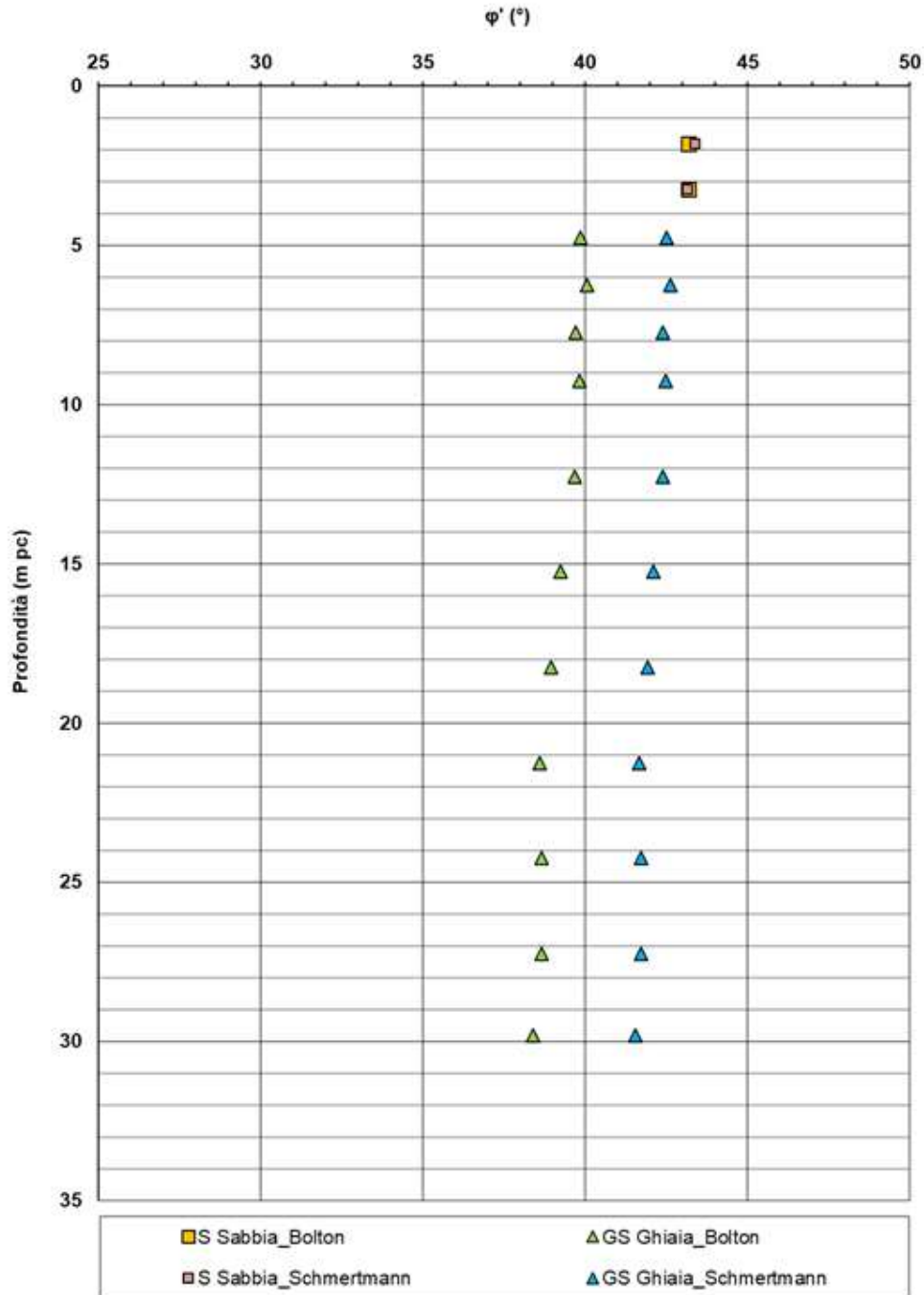
Figura 7 – Angoli di attrito da prove SPT tra pk 0+125 a pk 0+174
