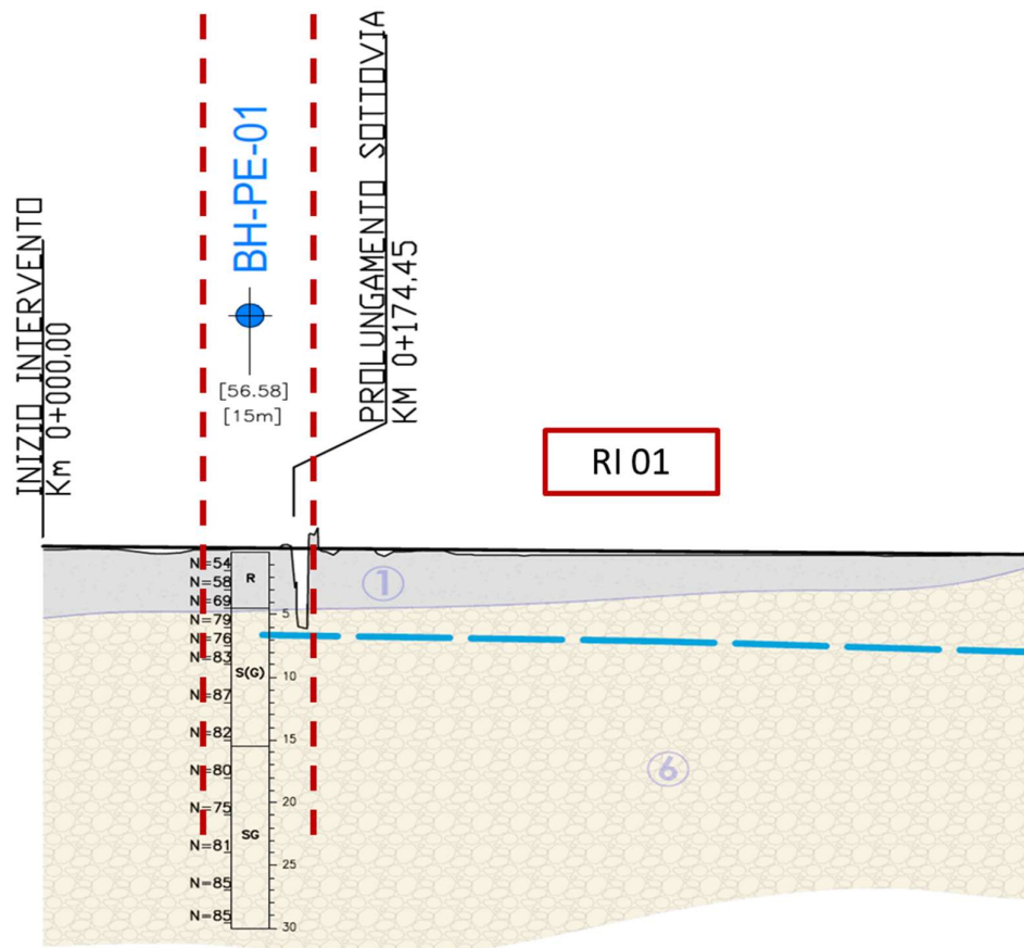
Figura 2 - Profilo Geotecnico Rilevato RI01, estratto dal Profilo Geotecnico Generale (Doc. Rif. [3])
