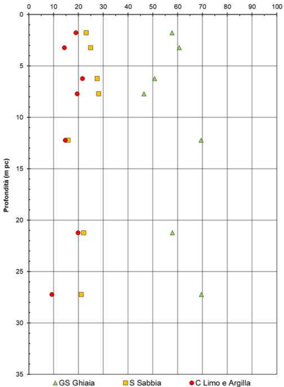
Figura 4 – Sintesi analisi granulometriche tra pk 0+125 a pk 0+174
