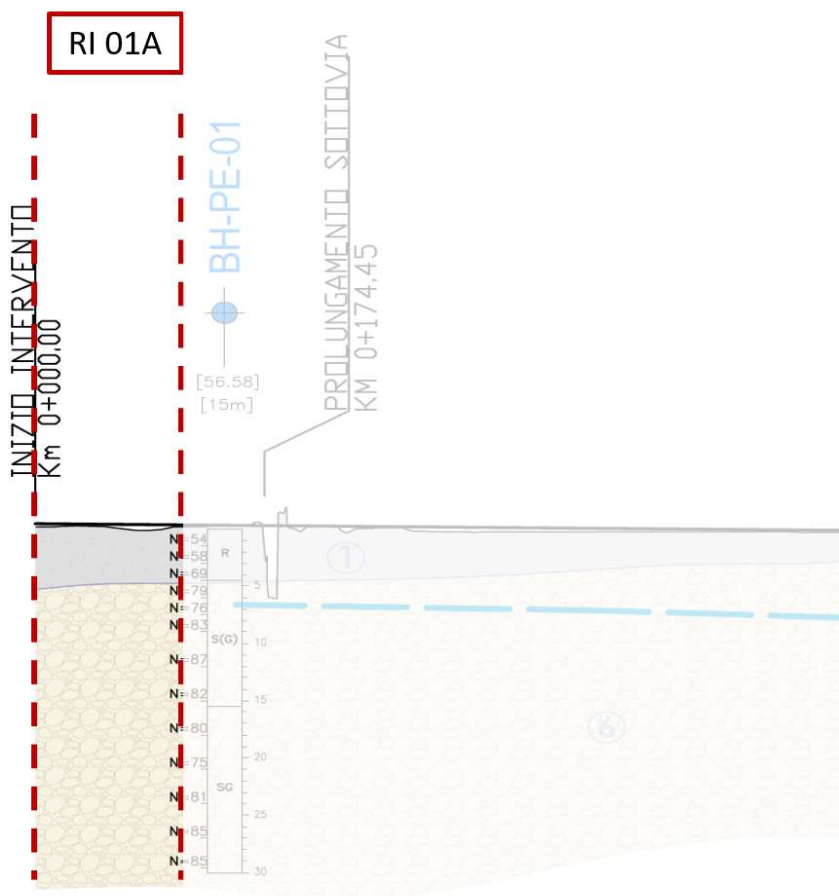
Figura 2 - Profilo Geotecnico Rilevato RI01A, estratto dal Profilo Geotecnico Generale (Doc. Rif. [3])
