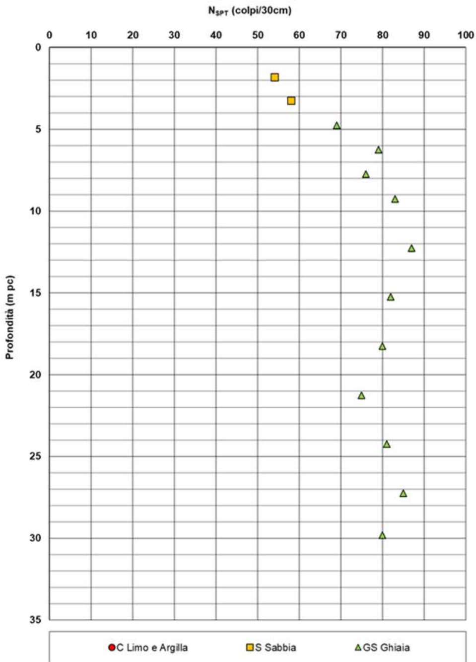
Figura 5 – Esito delle prove SPT tra pk 0+000 a pk 0+125
