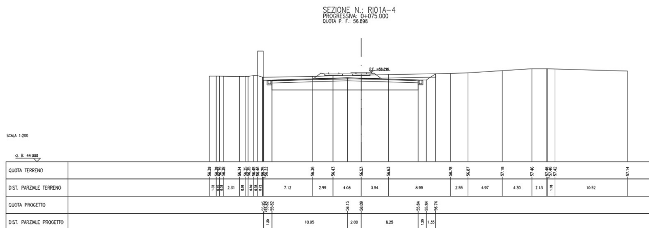
Figura 1 – Sezione di riferimento A (pk 0+075, n. RI01A-4) estratta da sezioni PE (Doc Rif. [1])
