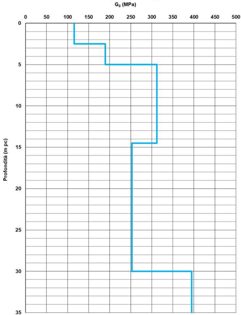
Figura 9 – Modulo di taglio G_0 tra pk 0+000 a pk 0+125
