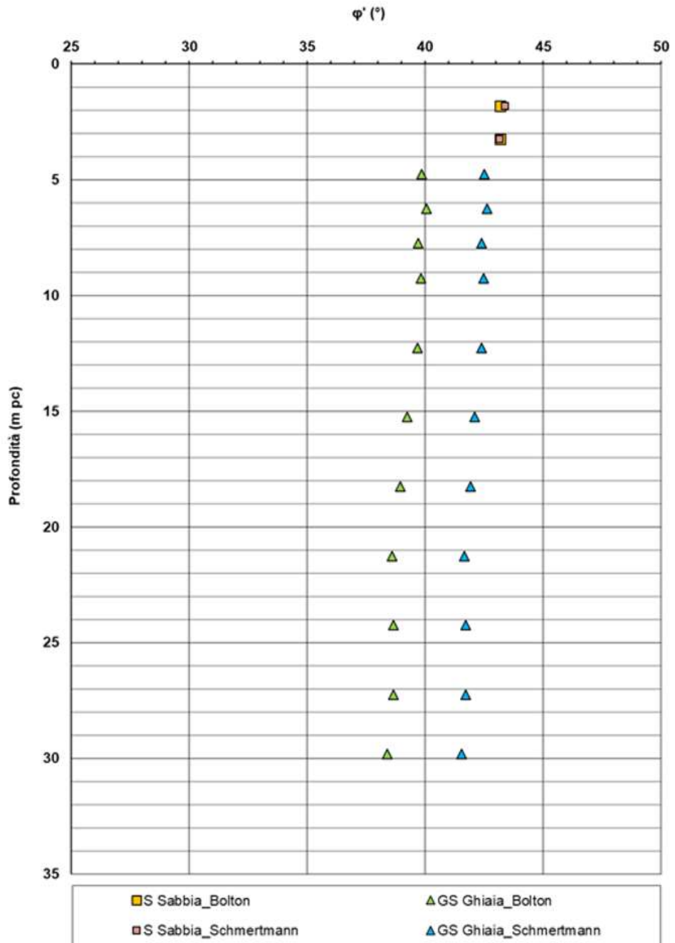
Figura 7 – Angoli di attrito da prove SPT tra pk 0+000 a pk 0+125
