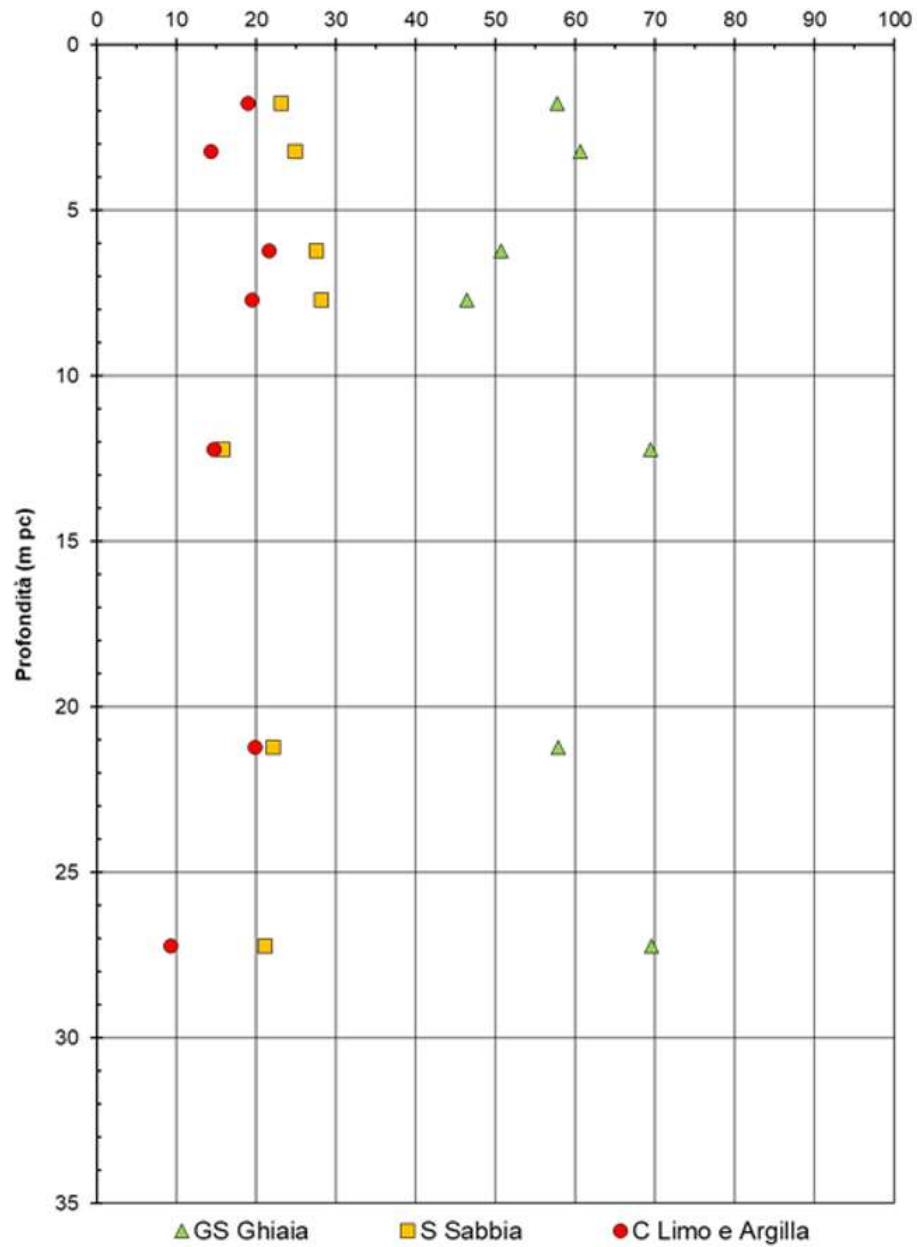
Figura 4 – Sintesi analisi granulometriche tra pk 0+000 a pk 0+125
