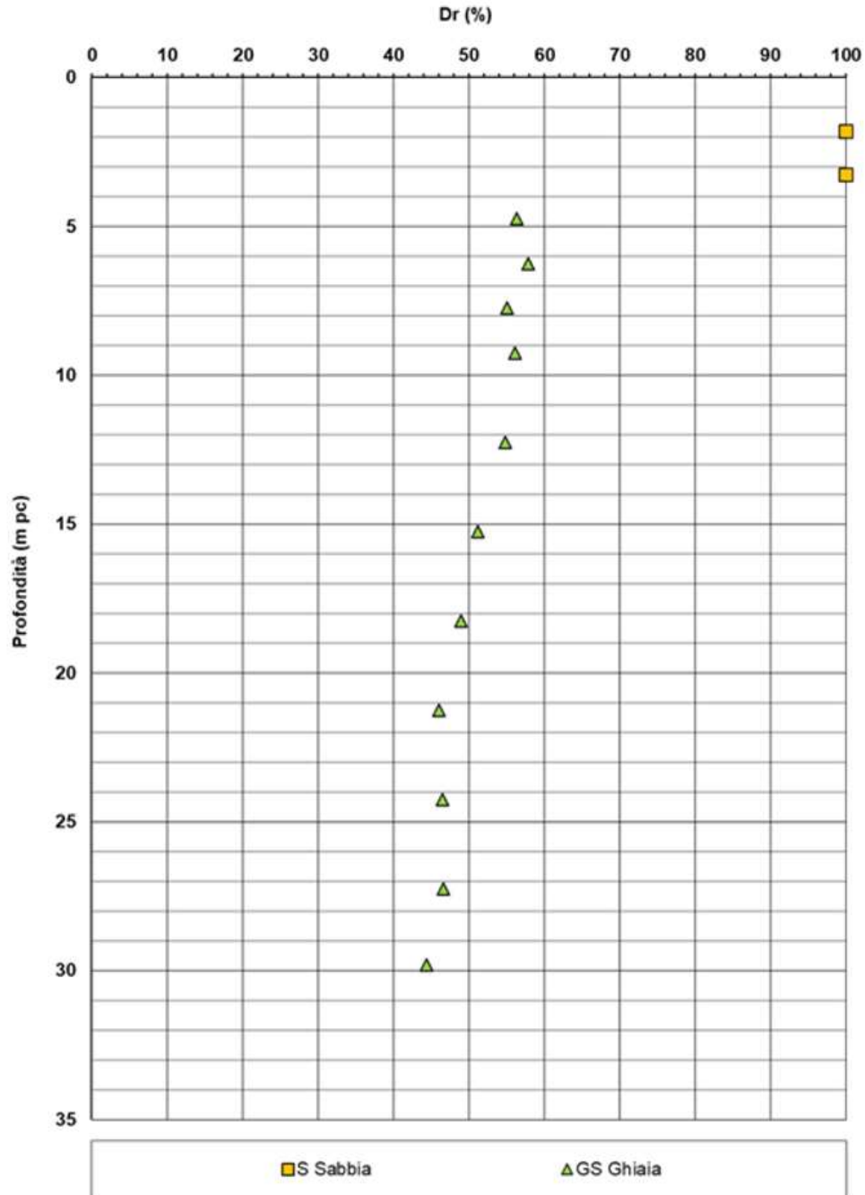
Figura 6 – Densità relativa da pro ve SPT tra pk 0+000 a pk 0+125
