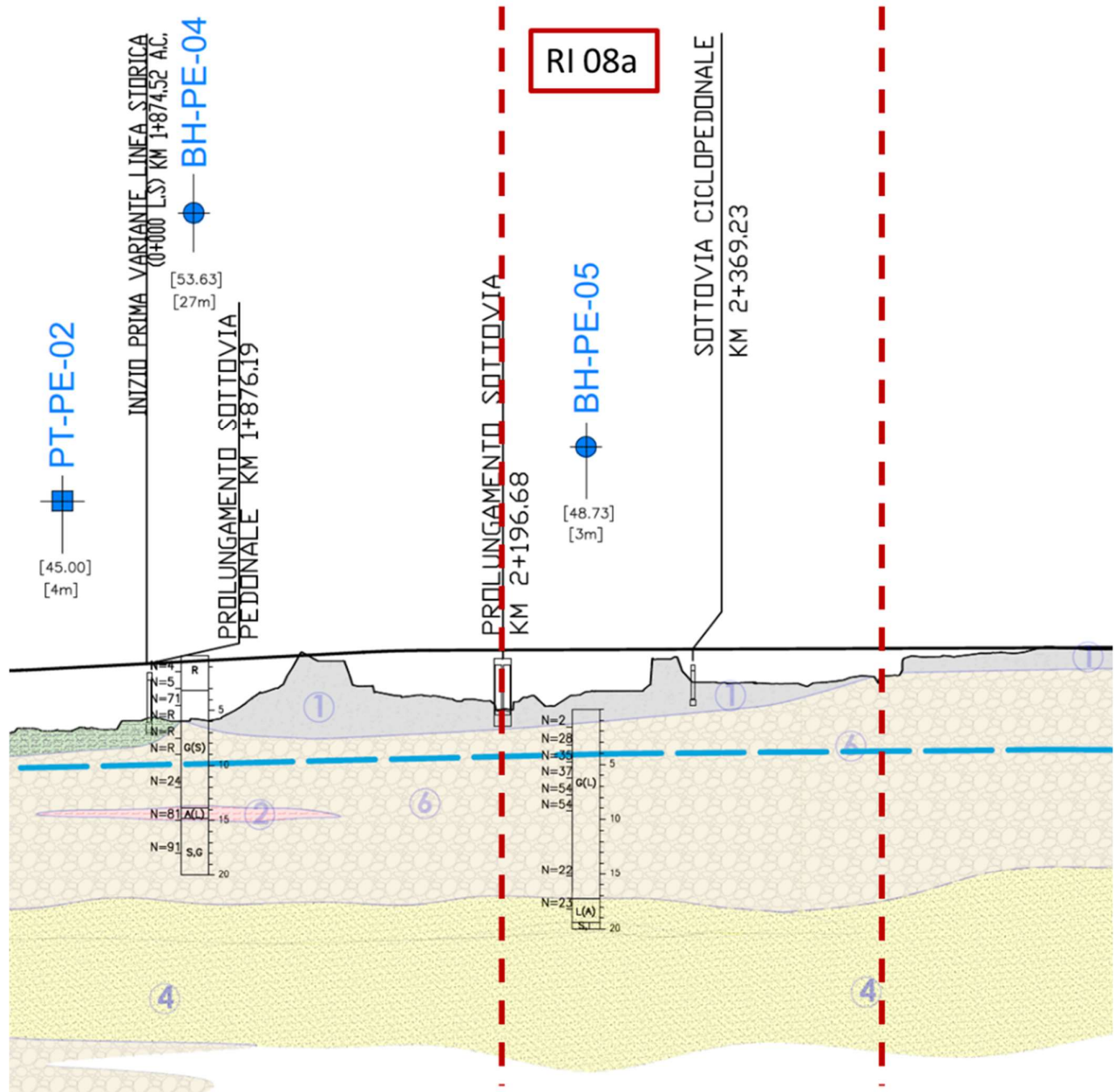
Figura 2 - Profilo Geotecnico Rilevato RI08A, estratto dal Profilo Geotecnico Generale (Doc. Rif. [3])
