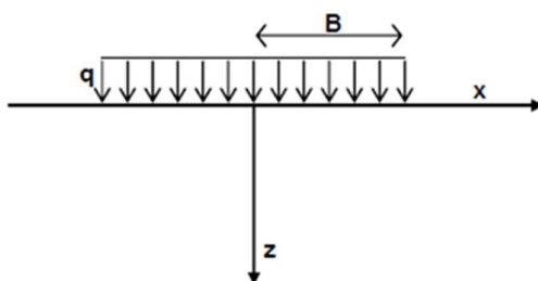
Figura 15 – Modello di calcolo Settle 3D – carico uniforme
