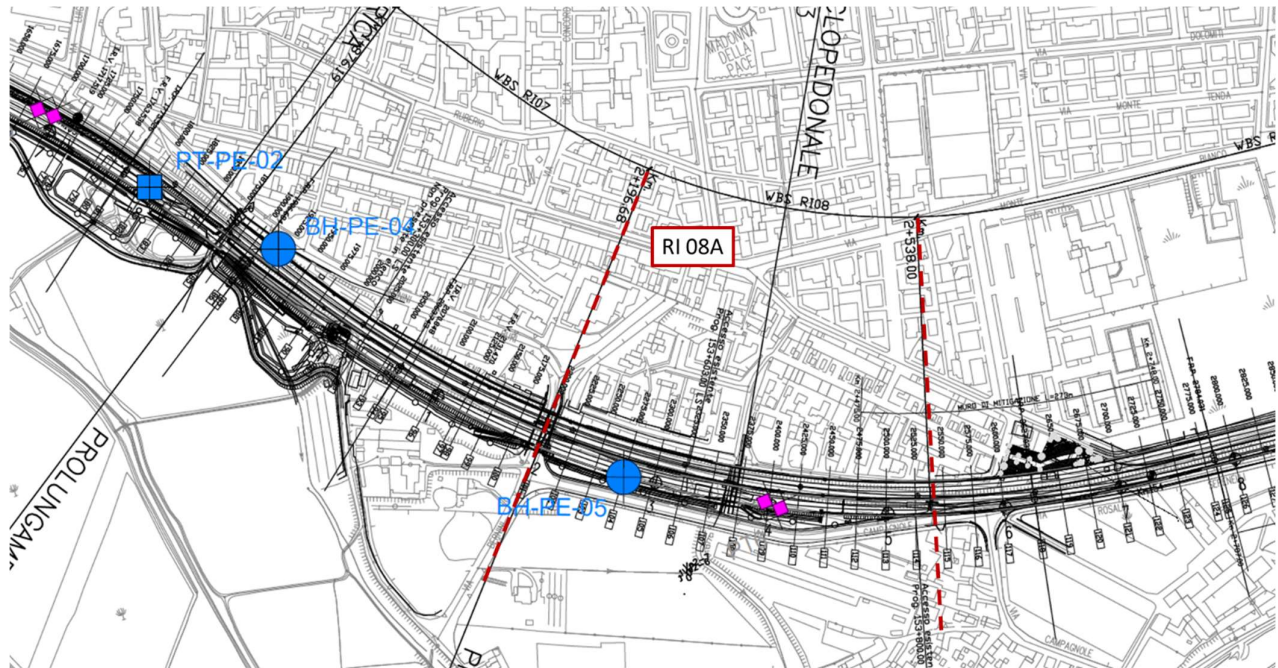
Figura 3 - Planimetria Rilevato RI08A, estratto dalla Planimetria Generale (Doc. Rif. [3])
